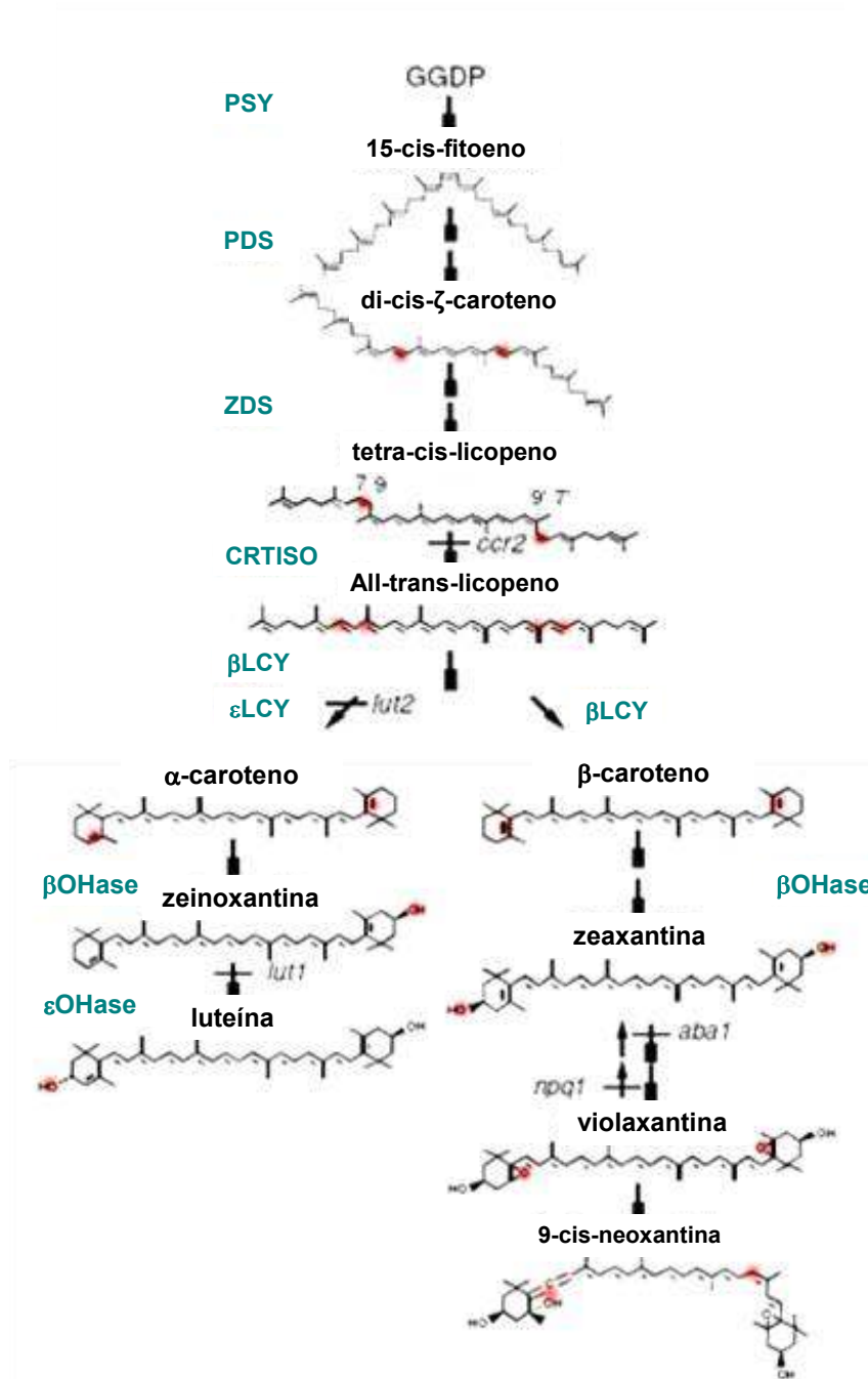
Figura 2: Biossíntese de carotenóides em plantas: o percurso mostra as principais etapas encontradas em quase todas as espécies vegetais. PSY: fitoeno sintase; PDS: fitoeno desaturase; B-LCY: β-caroteno ciclase; εLCY: ε-ciclase; βOHase: β-caroteno hidroxilase; εOHase: ε-caroteno hidroxilase.
