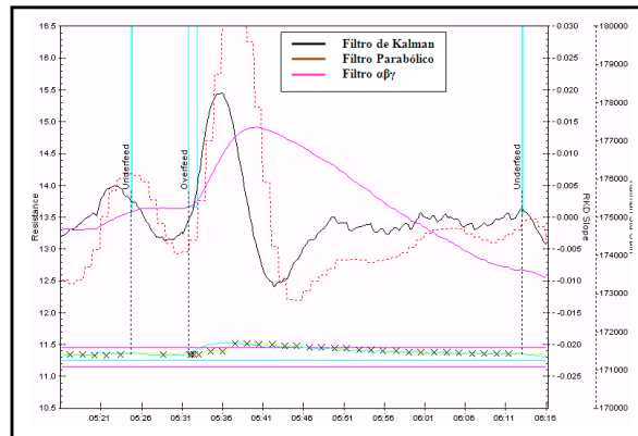
Figura 5.1: Medições do computador de processo - Cuba 1050 - 2 horas.
