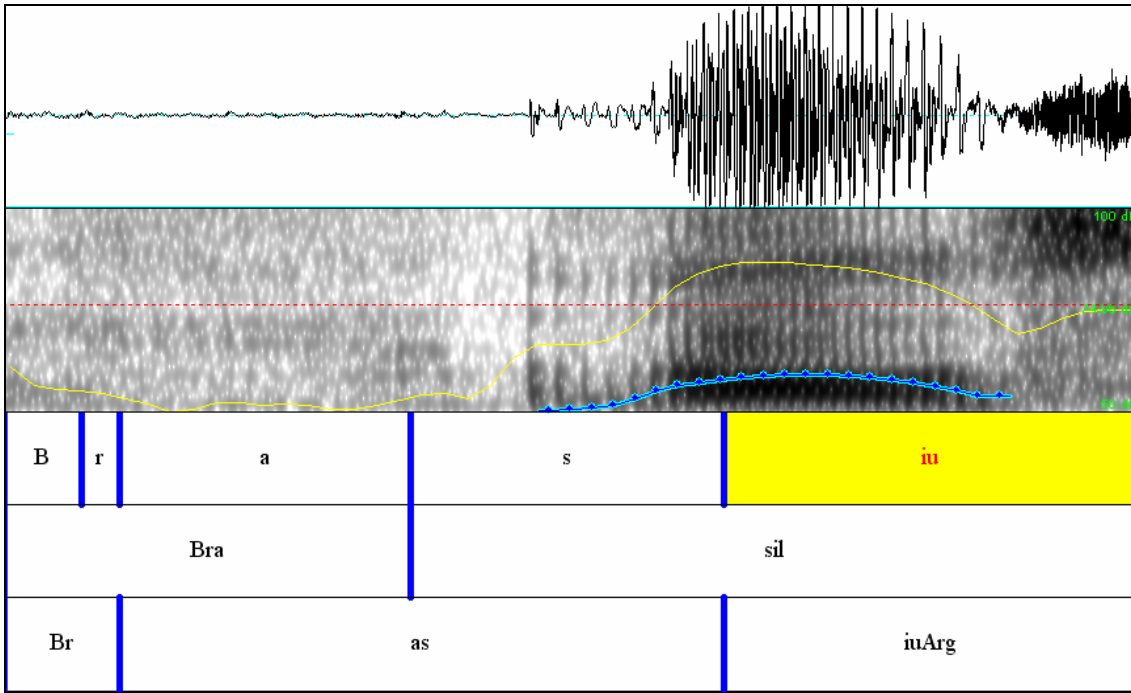
Figura 3 – TRAÇADO DA FORMA DA ONDA, ESPECTROGRAMA DE BANDA LARGA E CAMADAS DE SEGMENTAÇÃO DA PALAVRA “BRASIL”, MOSTRANDO OS CONTORNOS DE F0 NA LINHA AZUL PONTILHADA e INTENSIDADE NA LINHA AMARELA.
