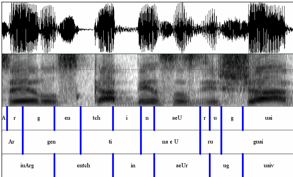
Figura 2 – TRAÇADO DA FORMA DA ONDA, ESPECTROGRAMA DE BANDA LARGA E CAMADAS DE SEGMENTAÇÃO DAS PALAVRAS “ARGENTINA E URUGUAI”, MOSTRANDO A DURAÇÃO DOS SEGMENTOS, DAS SÍLABAS E DAS UNIDADES VOGAL-VOGAL (GIPC).
