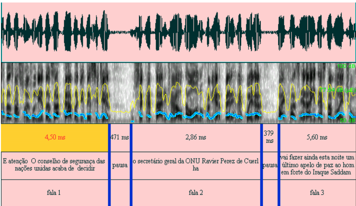
Figura 4 – TRAÇADO DA FORMA DA ONDA, ESPECTROGRAMA DE BANDA LARGA E CAMADAS DE SEGMENTAÇÃO DE UM TRECHO NARRADO POR UM JORNALISTA DA DÉCADA DE 80, MOSTRANDO OS SEGMENTOS DE FALA E AS PAUSAS EM MILISEGUNDOS.
