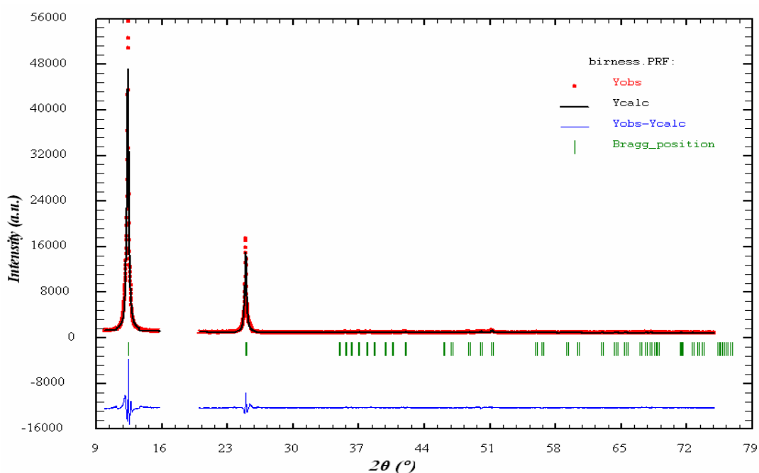
Figura 24: Diagrama de Rietveld para a amostra sintética de Na-birnessita (NaB2) após refinamento dos dados estruturais de célula unitária, background, deslocamento da amostra, W, U e V, posições atômicas, vibração isotrópica, assimetria, orientação preferencial.
