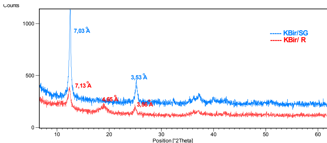
Figura 33: Difratograma de raios-X de K-birnessita obtida pelo método sol-gel (KBir/SG) e redução (KBir/ R). Fonte: Do autor
