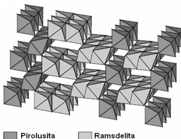
Figura 3. Estrutura idealizada de nsutita Fonte: (RZIHA, 1997).
