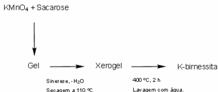
Figura 17: Diagrama esquemático mostrando a síntese sol-gel de k-birnessita. Fonte: (Suib et al., 1995).
