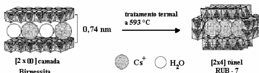
Figura 6: Uma reação modelo da transformação da estrutura birnessita para estrutura em túnel [2x4] por tratamento térmico Fonte: (FENG, 2003).
