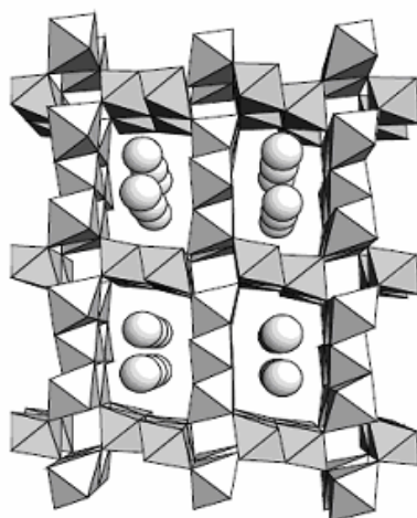
Figura 5. Ilustração da estrutura da romanechita. Fonte: (RZIHA, 1997).
