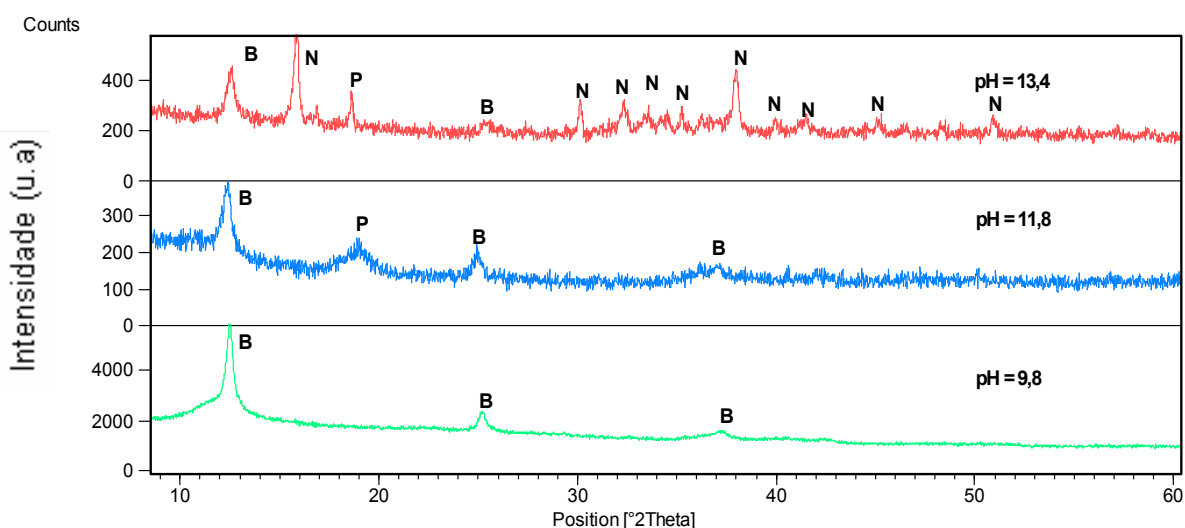
Figura 18: Difratograma de raios-X de Na-birnessita com variação de pH (Legenda: B-birnessita, P-pirocroita e N-outras fases de óxidos e hidróxidos de manganês não identificadas).
