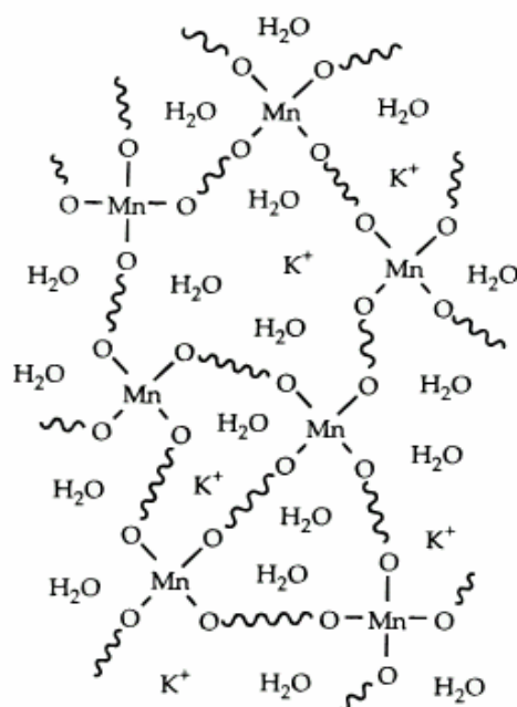
Figura 15: Ilustração do cross-linking para o gel de óxidos de manganês Fonte: (Ching et al., 1997).
