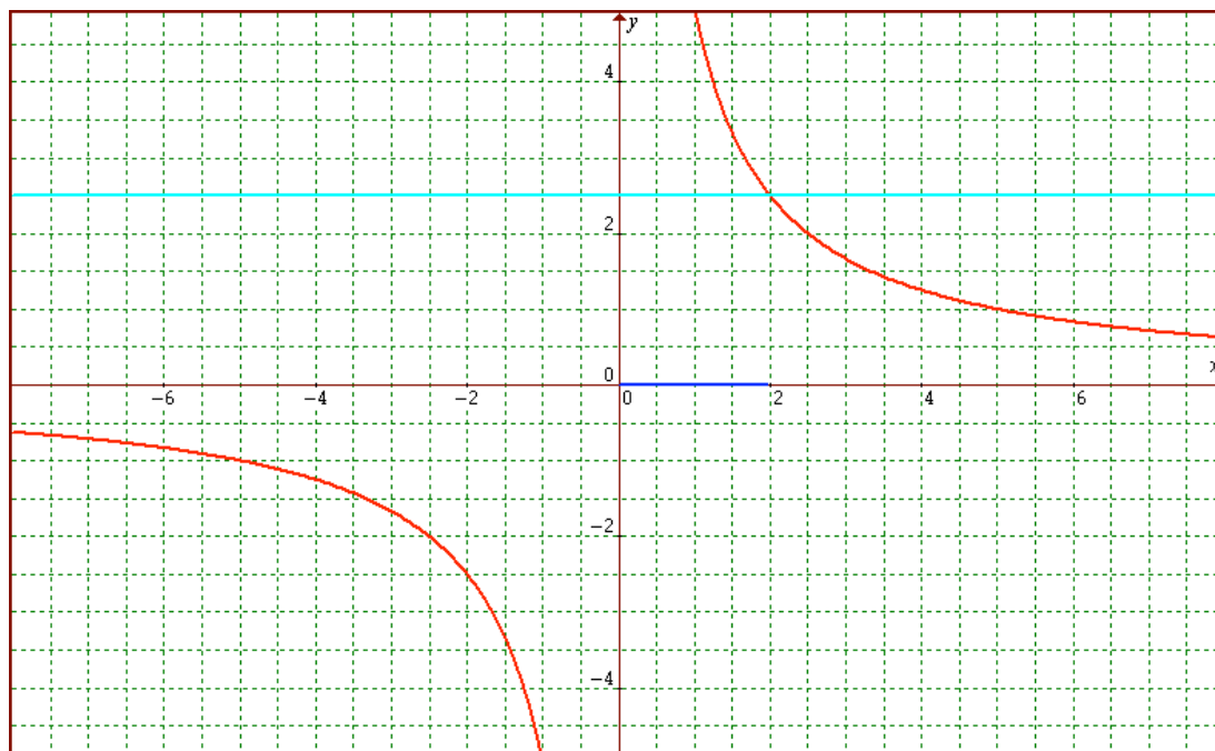
FIGURA 4: SOLUÇÃO GRÁFICA DA INEQUAÇÃO \frac{5}{x} > \frac{5}{2} .
