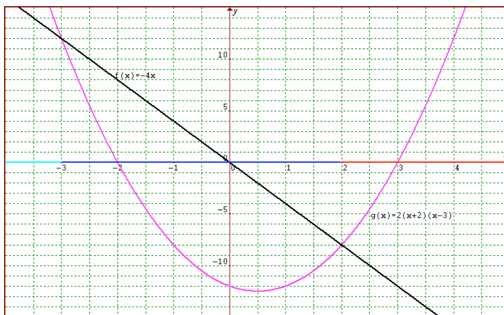
FIGURA 3: SOLUÇÃO GRÁFICA DE UMA INEQUAÇÃO
