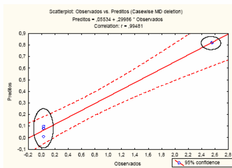
Figura 23 - Resultado da análise de correlação entre os dados preditos e observados pelo modelo. A diagonal representa um perfeito ajuste entre os dados.
