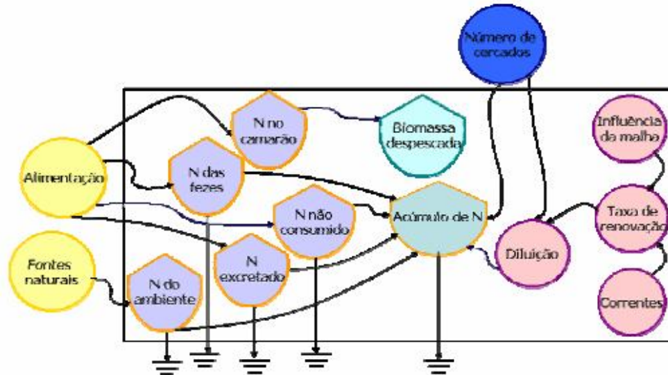
Figura 21 – Diagrama conceitual de um modelo da dinâmica do nitrogênio em um sistema semi-intensivo de cultivo do tipo cercados, representando a entrada de nitrogênio no sistema, passagens, transformações e saídas.
