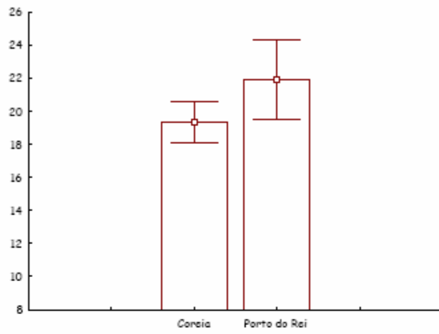
Figura 13 - Valores médios e erro padrão da salinidade ao longo do ciclo de produção na localidade da Coreia e do Porto do Rei, Ilha dos Marinheiros, Rio Grande, RS.
