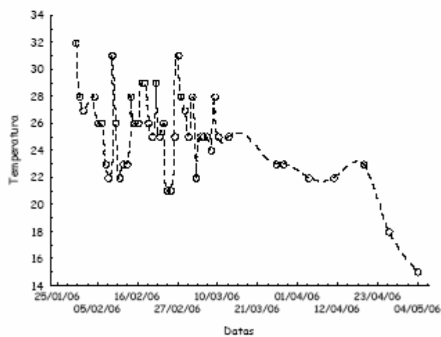
Figura 18 - Variação da temperatura da água ao longo do ciclo de produção na localidade da Coreia na Ilha dos Marinheiros, Rio Grande, RS.
