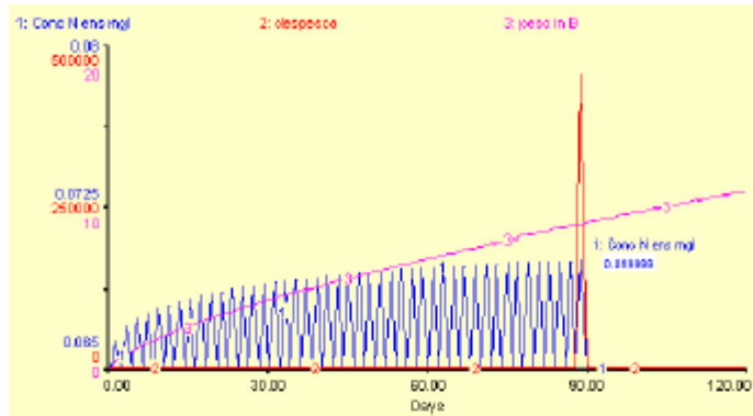
Figura 32 - Efeito do número de cercados (683) sobre a emissão de N- NT na enseada do Porto do Rei, com influência da malha e do estado de colmatção de 30% e valor médio de velocidade de corrente de 0,035m/s. Evolução da concentração de N-NT e crescimento dos organismos.
