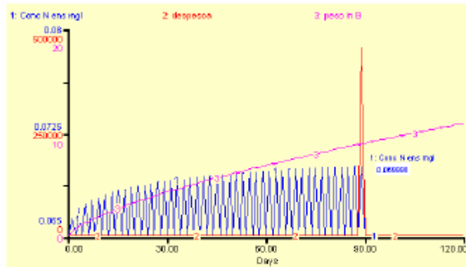
Figura 31 - Efeito do número de cercados (509) sobre a emissão de N-NT na enseada da Coreia, com uma influência do estado de colmatção da malha de 40% e velocidade de corrente de 0,04m/s. Evolução da concentração de N-NT e crescimento dos organismos.
