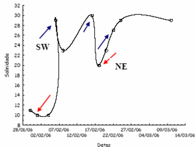
Figura 19 – Relação dos padrões de ventos e salinidade na localidade do Porto do Rei, ilha dos Marinheiros no estuário da Lagoa dos Patos, RS. As setas azuis indicam predominância de ventos do quadrante sul e as vermelhas, a predominância de ventos do quadrante norte.
