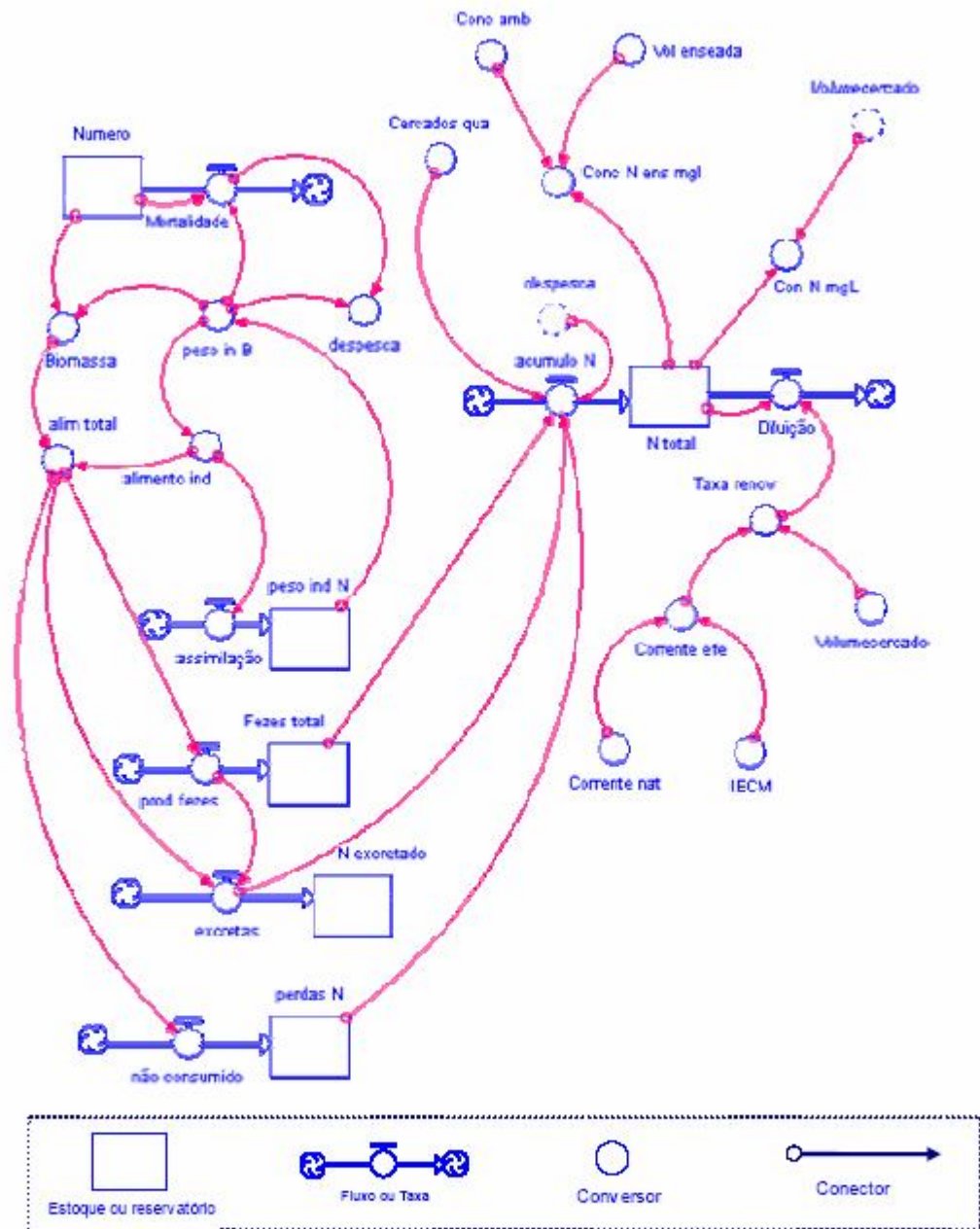
Figura 22 - Modelo numérico utilizado para determinação do número de cercados nas enseadas Porto do Rei e na Coreia, Ilha dos Marinheiros no estuário da Lagoa dos Patos.
