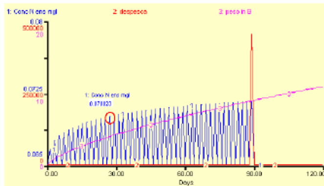
Figura 33 - Efeito do número de cercados (900) sobre a emissão de N-NT na enseada do Porto do Rei, com uma influência da malha e do estado de colmatação, sobre a passagem de água de 30% e valor médio de velocidade de corrente de 0,035m/s. Evolução da concentração de N-NT e crescimento dos organismos.
