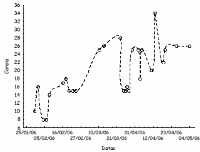
Figura 15 – Variação da salinidade ao longo do ciclo de produção na localidade da Coreia na Ilha dos Marinheiros, Rio Grande, RS.
