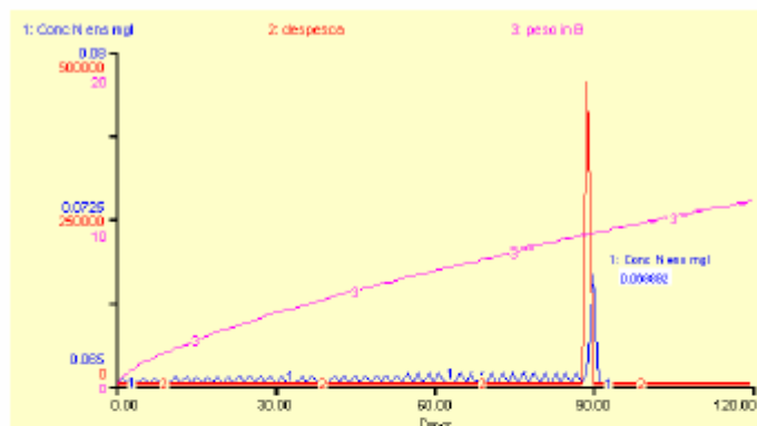
Figura 28 - Efeito de 41 cercados sobre a emissão de N-NT na enseada da Coreia, com uma influência da malha sobre a passagem da água de 20% e valor de velocidade de corrente de 0,01m/s. Evolução da concentração de N-NT e crescimento dos organismos.
