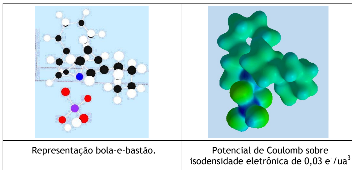
Figura 4.21. Modelo para o [(\text{OH})_2\text{Si}(\mu\text{-O})_2]\text{Zr}(\text{nBuCp})_2
