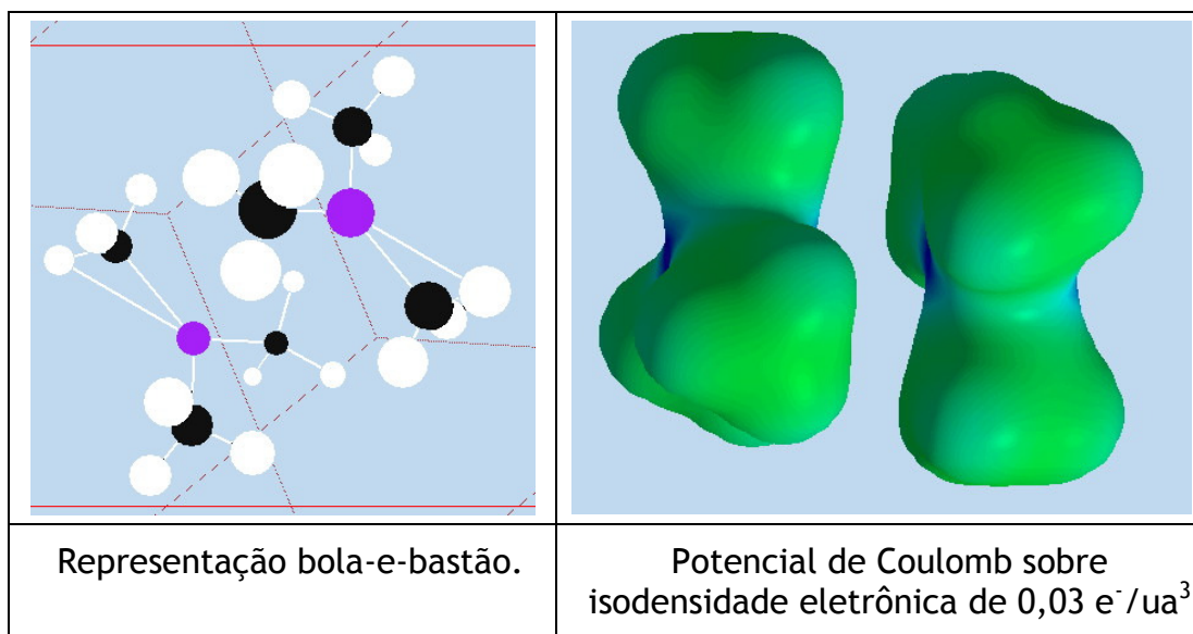
Figura 4.7. Dímero de TMA com alumínios ligados
