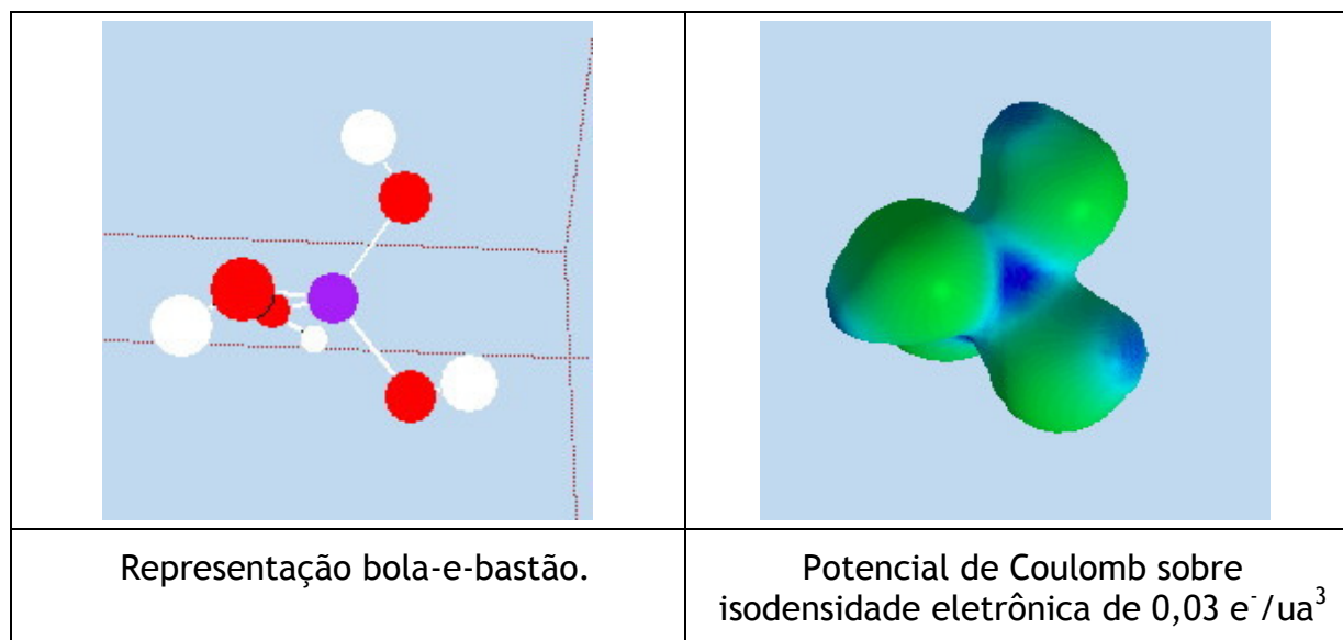
Figura 4.14. \text{Si}(\text{OH})_4 : modelo para o ácido silícico.
