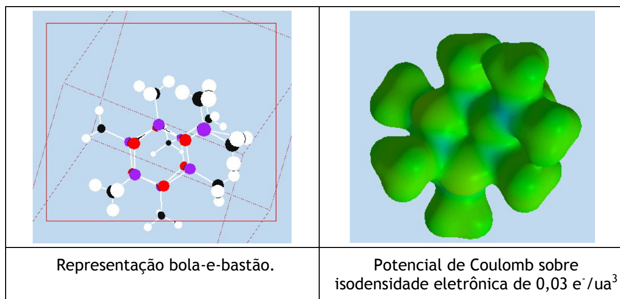
Figura 4.11. MAO 6 .TMA - modelo para co-catalisador MAO com sítio ácido de Lewis.
