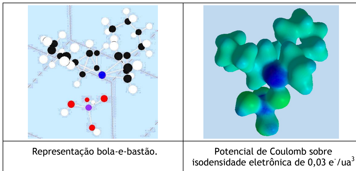
Figura 4.22. Modelo para o \{[(OH)_3Si(\mu-O)]Zr(nBuCp)_2\}^+
