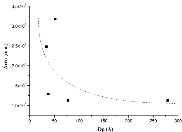
Figura 31. Concentração do acetato de isoamila adsorvido na fibra DVB-CAR-PDMS, em presença de sílicas, dotadas de diferentes valores de diâmetro de poro.
