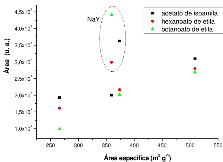
Figura 41. Concentração dos analitos adsorvidos na fibra DVB-CAR-PDMS, em presença de zeólitas dotadas de diversas áreas específicas.
