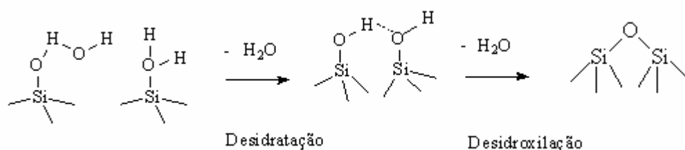
Esquema 6. Desidratação e desidroxilação da superfície da sílica.
