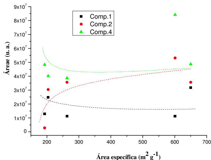
Figura 32. Concentração dos analitos acetato de isoamila (1), hexanoato de etila (2) e octanoato de etila (4) adsorvidos na fibra DVB-CAR-PDMS, em presença de sílicas, dotadas de diferentes valores de área específica.
