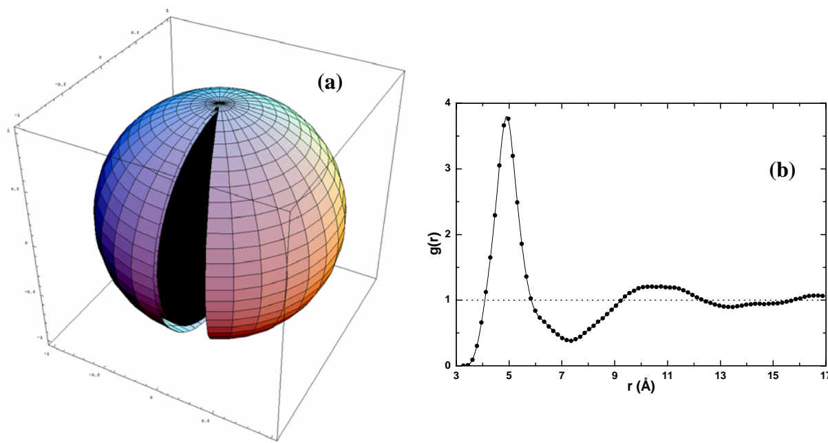
Figura 31: (a) Desenho esquemático da casca esférica onde é medida a função num dado r e o volume para a normalização; (b) Uma RDF típica.
