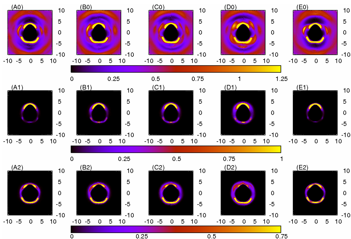
Figura 106: SDF_{YX} (abscissas e ordenadas em Å) medidas a partir das origens dos sistemas de coordenadas dos cátions em direção aos átomos de flúor dos fluoretos ( F^- ) dos cinco ILs compostos de ânions “complexos”, em conjunto com as suas respectivas SDFs “rankeadas”: (A0) total EMI·F·1,0HF, (B0) total EMI·F·2,0HF, (C0) total EMI·F·2,3HF, (D0) total EMI·F·3,0HF, (E0) total EMI·F, (A1) par mais próximo do EMI·F·1,0HF, (B1) par mais próximo do EMI·F·2,0HF, (C1) par mais próximo do EMI·F·2,3HF, (D1) par mais próximo do EMI·F·3,0HF, (E1) par mais próximo do EMI·F, (A2) segundo par mais próximo do EMI·F·1,0HF, (B2) segundo par mais próximo do EMI·F·2,0HF, (C2) segundo par mais próximo do EMI·F·2,3HF, (D2) segundo par mais próximo do EMI·F·3,0HF, (E2) segundo par mais próximo do EMI·F.
