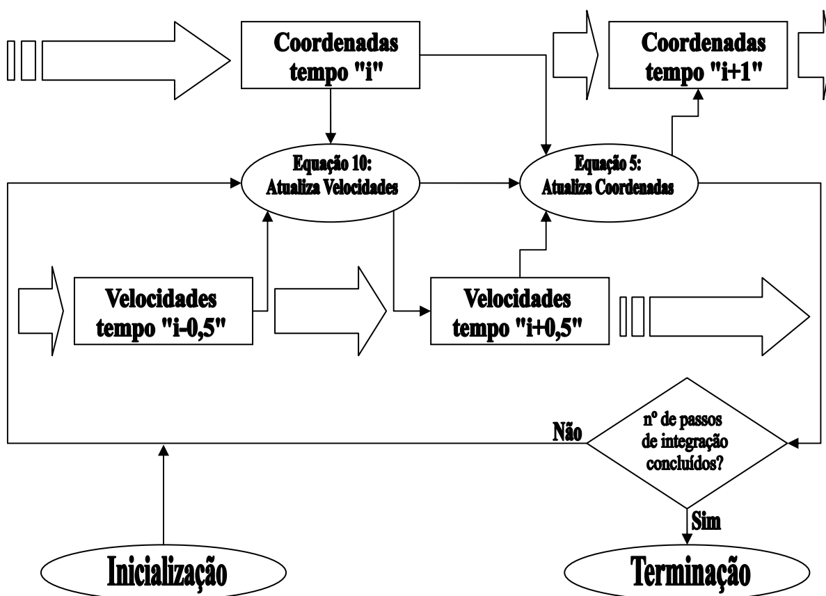
Figura 5: Esquema de funcionamento geral do algoritmo Leap-Frog Verlet em simulações de Dinâmica Molecular (MD).
