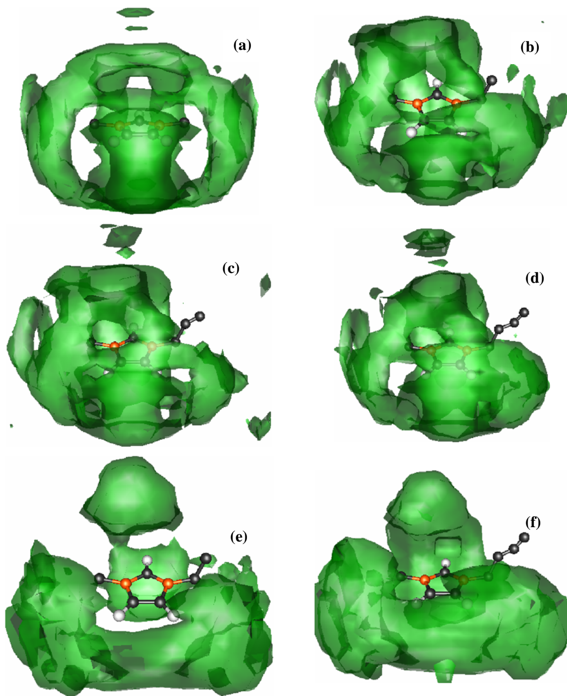
Figura 58: 3D-SDFs (em verde) medidas de H2\cdots X , H4\cdots X e H5\cdots X (onde X = Cl ou F ) ao redor dos cátions dos ILs: (a) MMI\cdot AlCl_4 , (b) EMI\cdot AlCl_4 , (c) PMI\cdot AlCl_4 , (d) BMI\cdot AlCl_4 , (e) EMI\cdot BF_4 , (f) BMI\cdot BF_4 . Em todos os casos as regiões de densidade populacional apresentadas representam populações iguais ou maiores que 2,0.
