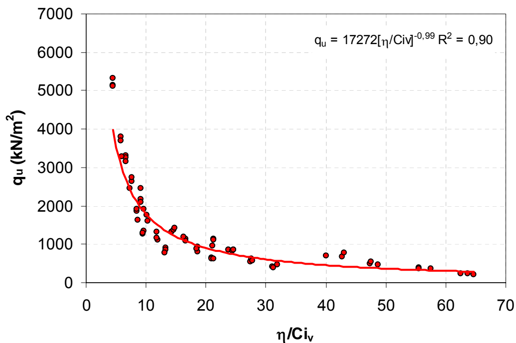
Figura 4.7- Resistência à compressão simples x relação vazios/cimento.
