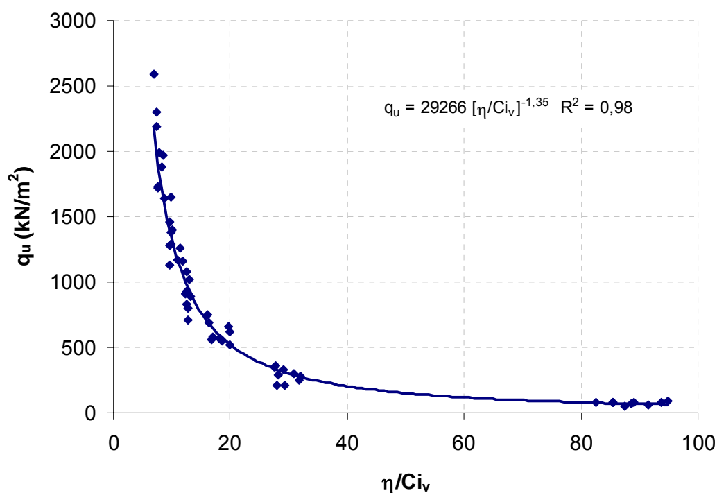
Figura 4.5 – Resistência à compressão simples x fator vazios/cimento expresso em termos da porosidade e do teor de cimento volumétrico.
