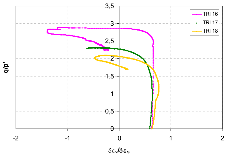
Figura 4.74 – Tensão-dilatância de amostras com 10,3% de cimento e índice de vazios inicial de 0,80.
