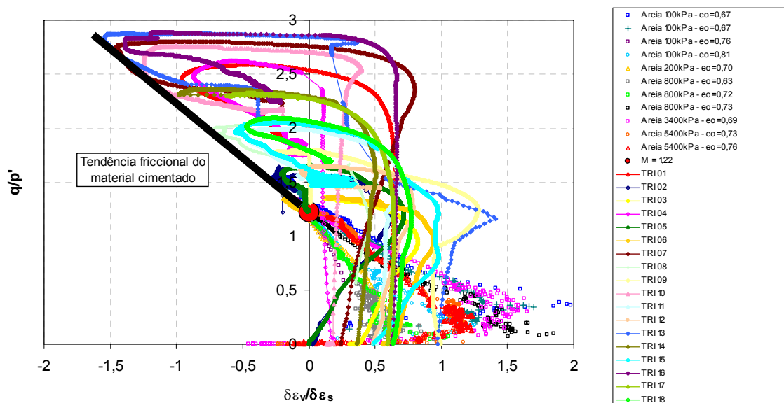
Figura 4.82 – Dilatância de ensaios realizados na areia (Santos, 2008)
