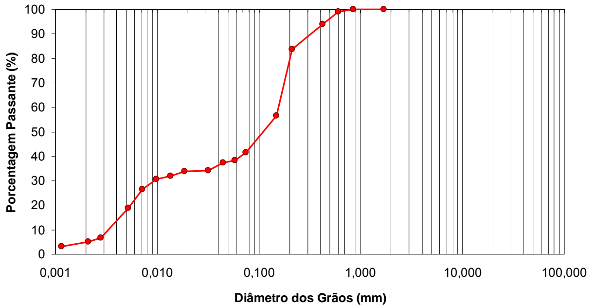
Figura 4.6 – Curva granulométrica do SRAB.
