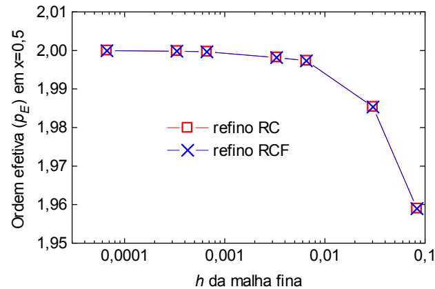
Figura 4.10 – Ordem efetiva do problema 5B para malha grossa uniforme.
