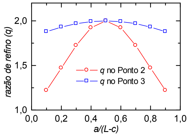
Figura 3.5 – Valor da razão de refino ( q ) que reproduz a ordem assintótica ( p_L ), para as malhas da Fig. 3.3 com c = 3L/4 .
