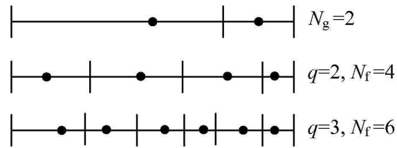
Figura 6 – Refinos aleatórios (RA).
