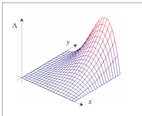
Figura 6.6 – Superfície gerada pela Eq (6.11).
