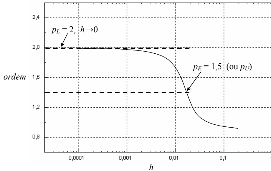
Figura 2.5 – Ordem efetiva ( p_E ) e assintótica ( p_L ) com redução de ( h ).
