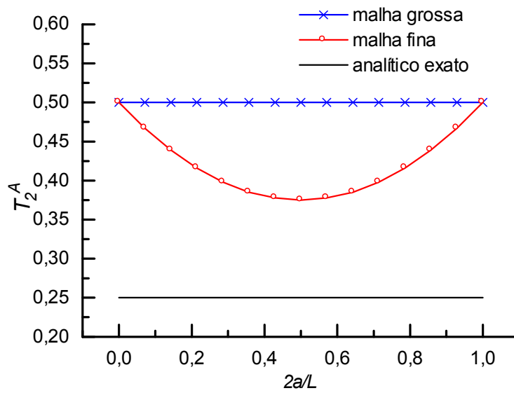
Figura 3 – Soluções do problema A ( T^A ) no ponto 2 para as malhas da Fig. 2.
