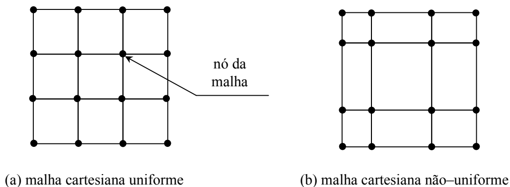
Figura 2.1 – Exemplos de discretização para diferenças finitas.
