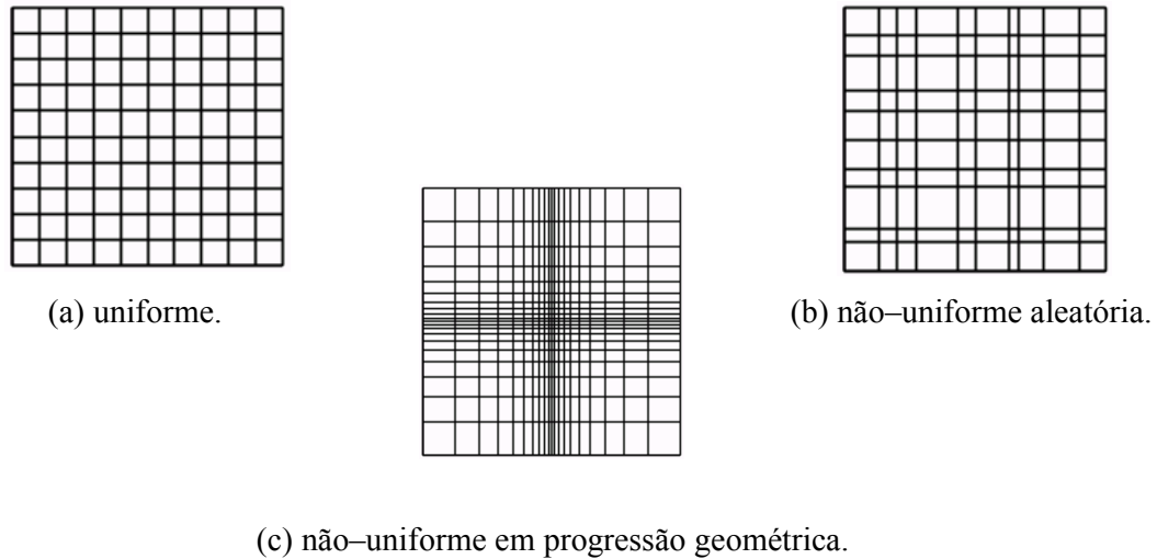
Figura 5.2 – Malhas bidimensionais cartesianas para diferenças finitas.
