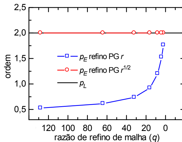
Figura 3.13 – Ordem efetiva do problema 3A, para malha grossa com N_g = 1000 e r=1,01 .
