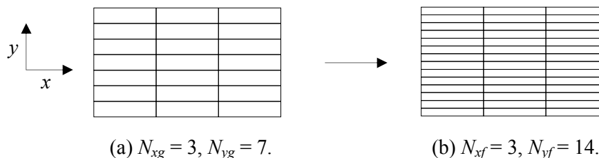
Figura 5.7 – Malha (a) grossa uniforme por direção e (b) malha fina obtida com refino uniforme em y (refino direcional).
