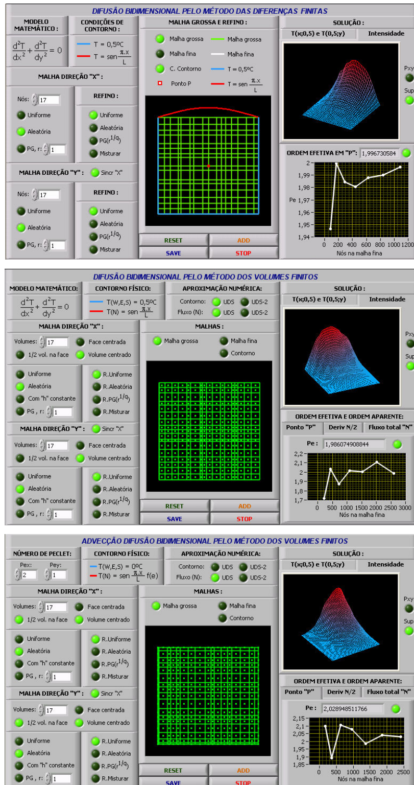
Figura 2.9 – Interface gráfica de programas 2D.
