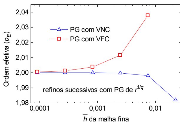
Figura 4.17 – Ordem efetiva do problema 8, no intervalo x = [0;0,5] , para malha grossa não-uniforme do tipo VFC .
