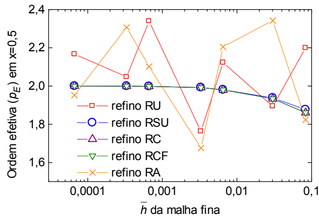
Figura 4.11 – Ordem efetiva do problema 6A para malha grossa não-uniforme do tipo VFC .
