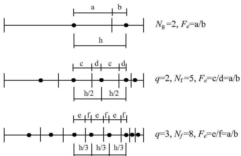
Figura 4 – Refinos entre centros (RC).
