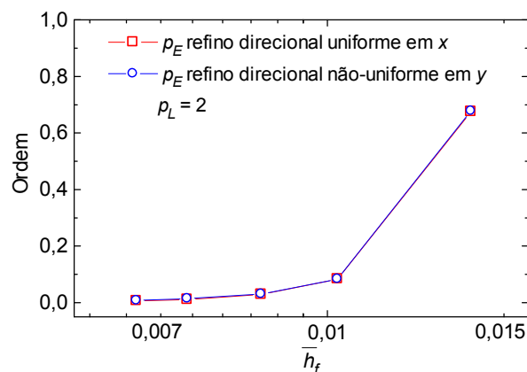
Figura 5.8 – Ordem efetiva do problema 9, no ponto P , para malha grossa não-uniforme com refino direcional.
