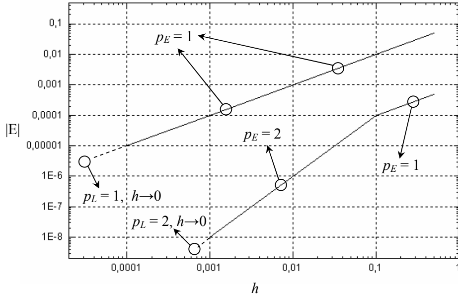
Figura 2.4 – Ordem assintótica ( p_L ) e efetiva ( p_E ) do erro (adaptado de Marchi, 2001).
