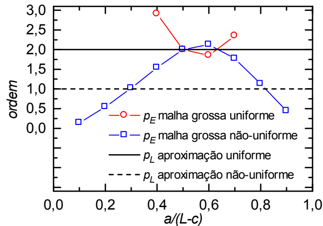
Figura 3.9 – Ordem efetiva (p_E) do problema 2A no ponto 2, para as malhas da Fig. 3.3.
