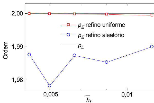
Figura 5.4 – Ordem efetiva do problema 9A, no ponto P , para malha grossa uniforme.
