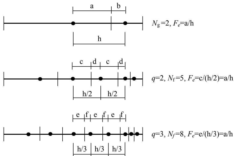
Figura 4.6 – Refinos entre centros com F_e constante ( RCF ).
