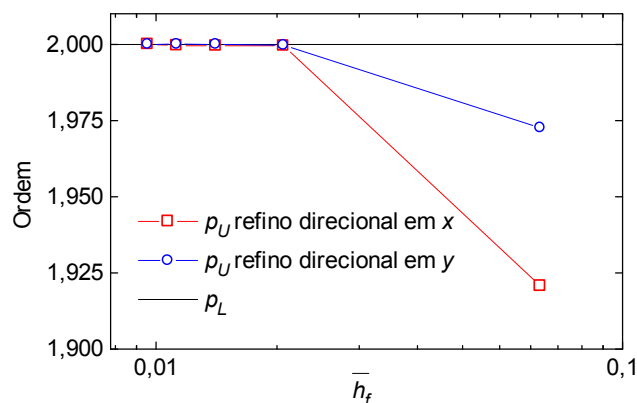
Figura 6.4 – Ordem aparente do problema 10A, no ponto P , para malha grossa não-uniforme VNC e com refino direcional do tipo RU .
