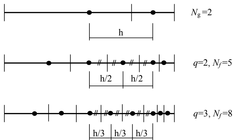
Figura 4.5 – Refinos entre centros (RC).
