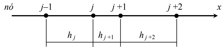
Figura 2.6 – Malha unidimensional não-uniforme.
