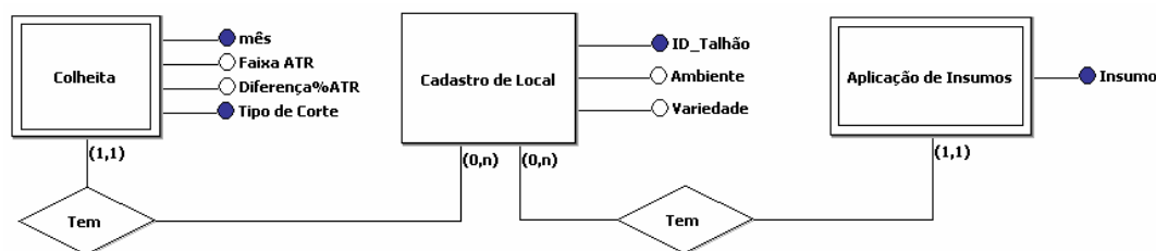
FIGURA 4.1: ESQUEMA DO BANCO DE DADOS PREPARADO PARA A MINERAÇÃO
