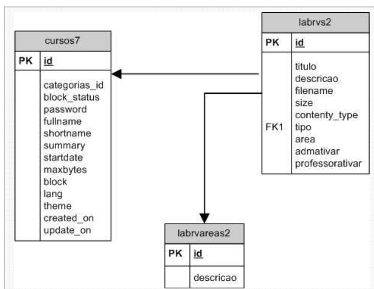
Figura 6.28 – Modelo de dados do Módulo de Lab2D/3D
