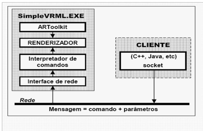
Figura 4.8 – Estrutura do NetArTollKit
