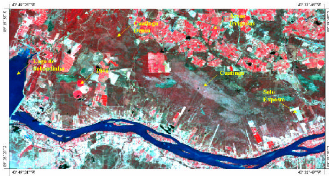
Figura 4.1a - Composição RGB das bandas 4, 3, 2 do Mapeador Temático do Landsat 5, uma visão geral da área de interesse em 04/12/2000
