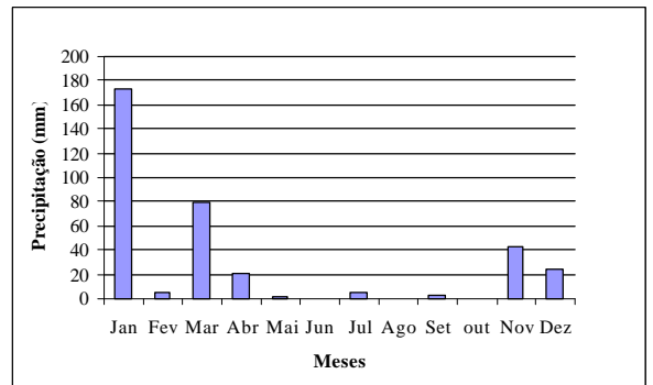
Figura 3.3f- Precipitação mensal em 2003
