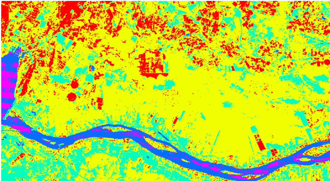
Figura 4.9a – Carta do IVDN obtida com o Landsat 5 em 04/12/2000
