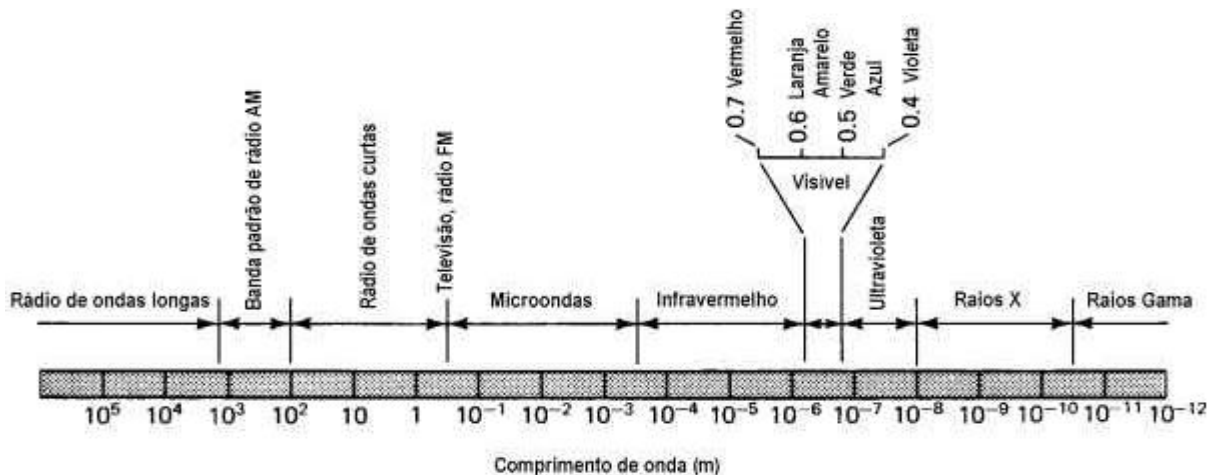
Figura 2.2: Espectro da radiação eletromagnética. Fonte: Barbosa (1996).
