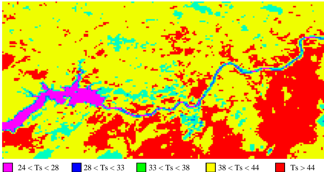
Figura 4.15- Carta da temperatura da superfície(°C) obtida com o NOAA-16 em 04/10/2001
