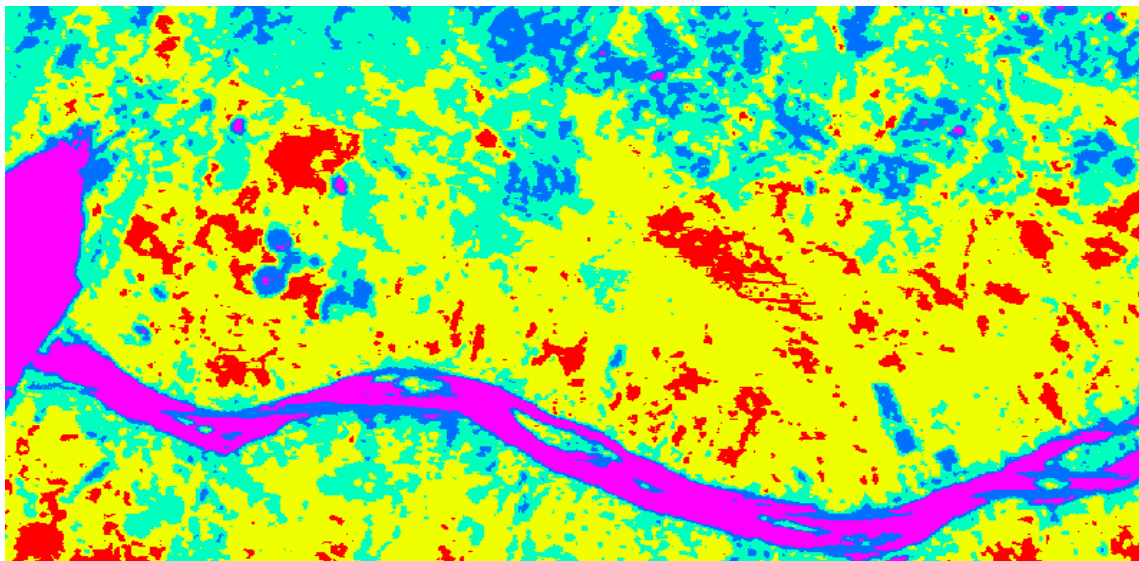
Figura 4.41b - Carta do fluxo de calor sensível ( Wm^{-2} ) obtido com o Landsat 5 da em 04/10/2001
