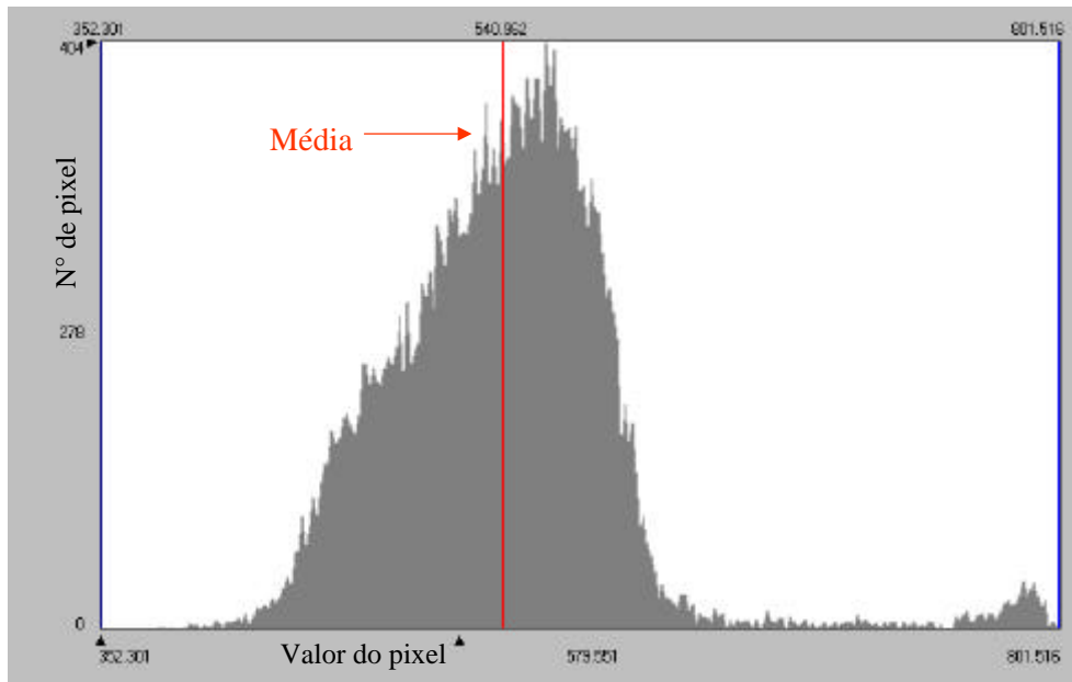
Figura 4.32- Histograma de frequência do saldo de radiação ( \text{Wm}^{-2} ) obtido com o NOAA-16 em 24/09/2003
