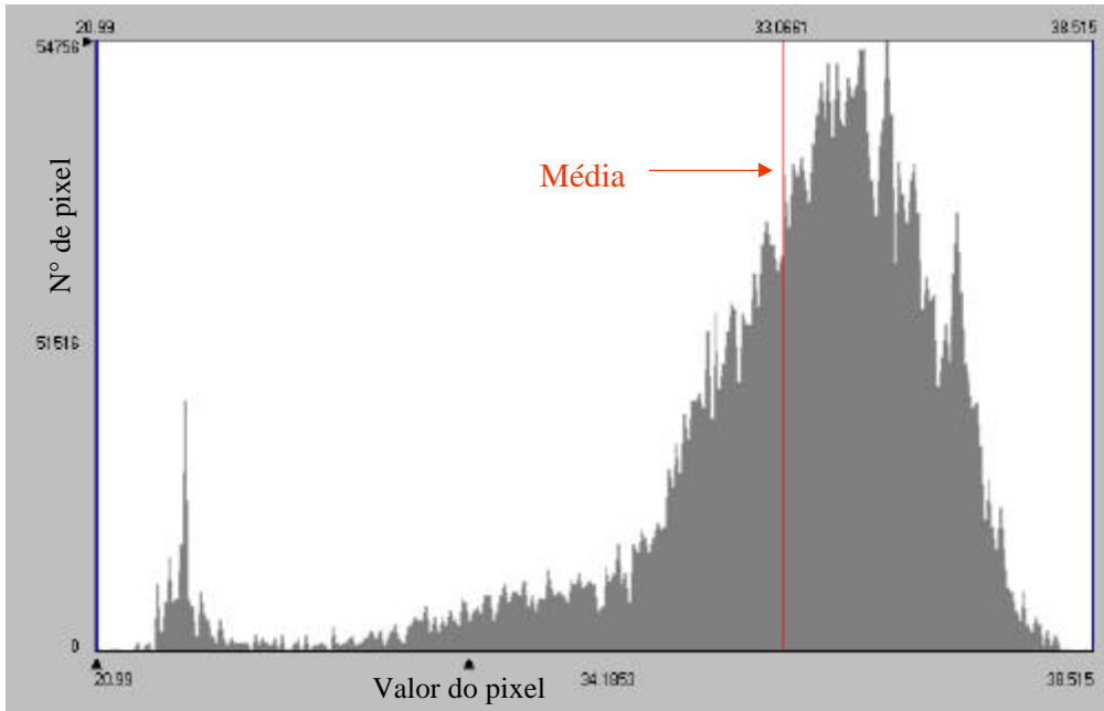
Figura 4.19 - Histograma de freqüência da temperatura da superfície (°C) obtida com Landsat 5 em 24/09/2003
