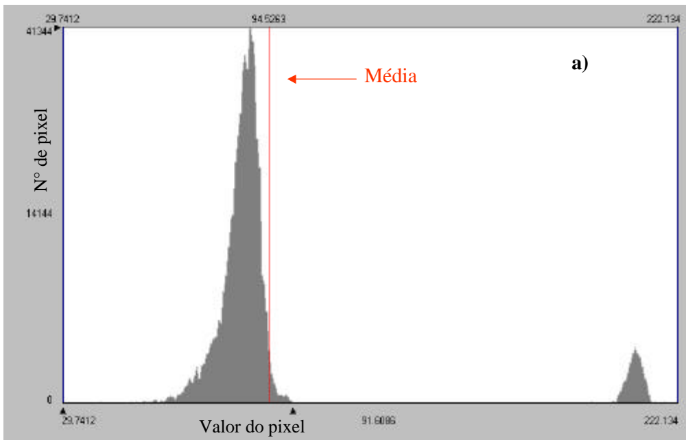
Figura 4.34a - Histograma de frequência do Fluxo de calor no solo ( Wm^{-2} ) obtido com o Landsat 5 em 04/12/2000
