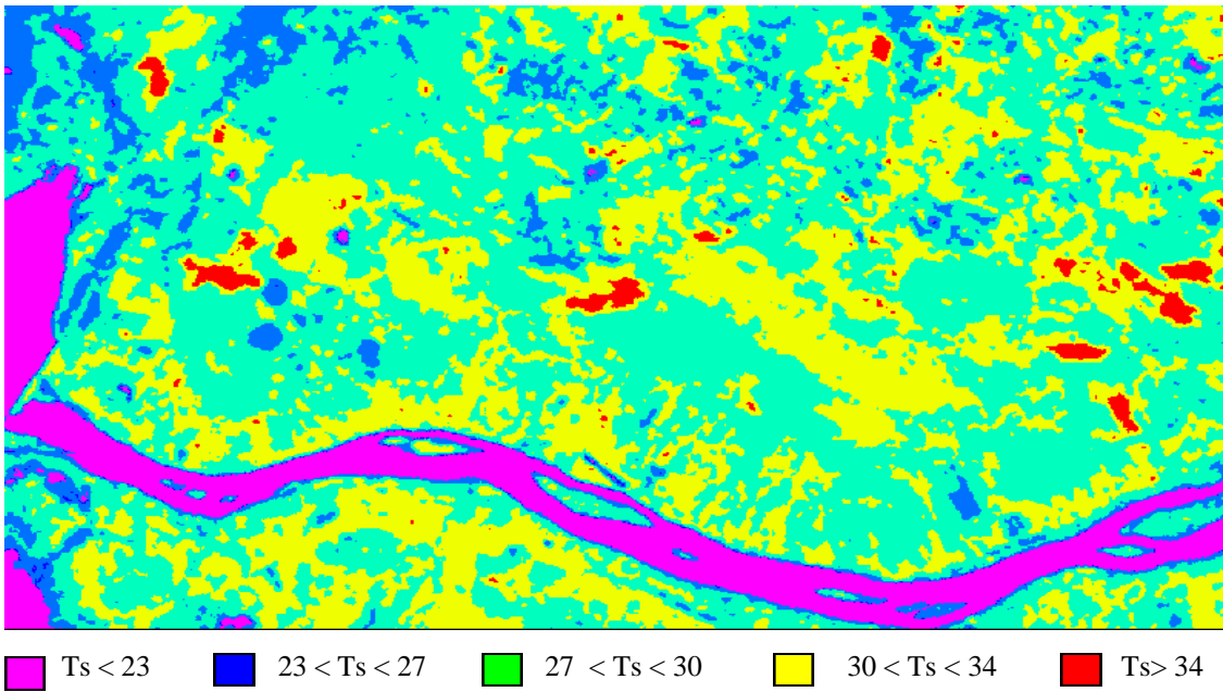
Figura 4.13a – Carta da temperatura da superfície (°C) obtida com o Landsat 5, em 04/12/2000
