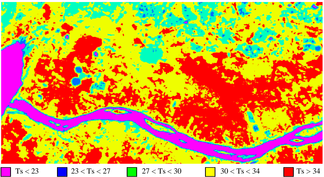
Figura 4.13b - Carta da temperatura da superfície (°C) obtida com o Landsat 5, em 04/10/2001
