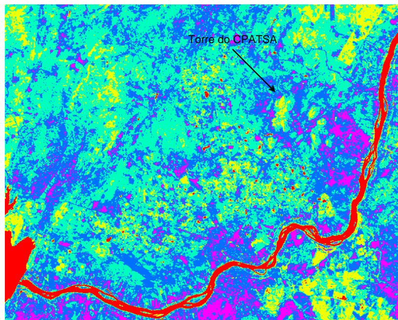
Figura 4.63 - Carta de evapotranspiração (mm/dia) obtida com Landsat 5 em 12/10/2004
