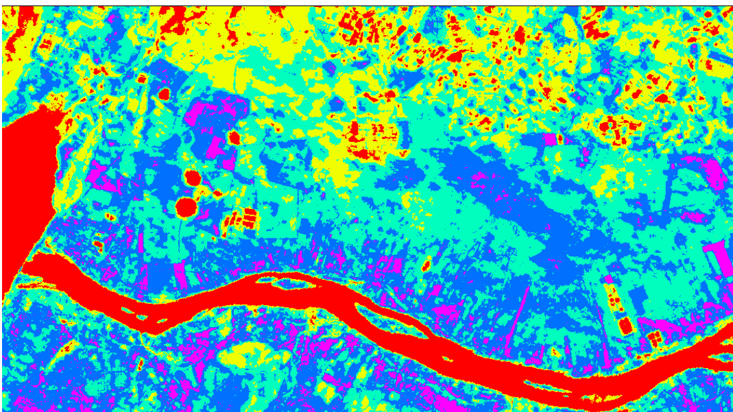
Figura 4.49a - Carta do fluxo de calor latente ( \text{Wm}^{-2} ) obtido com o Landsat 5 em 04/12/2000
