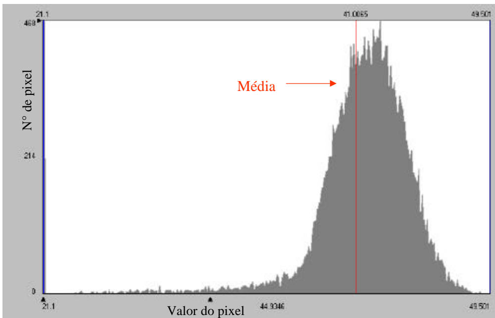
Figura 4.20 - Histograma de freqüência da temperatura da superfície (°C) obtida com o NOAA-16 em 24/09/2003
