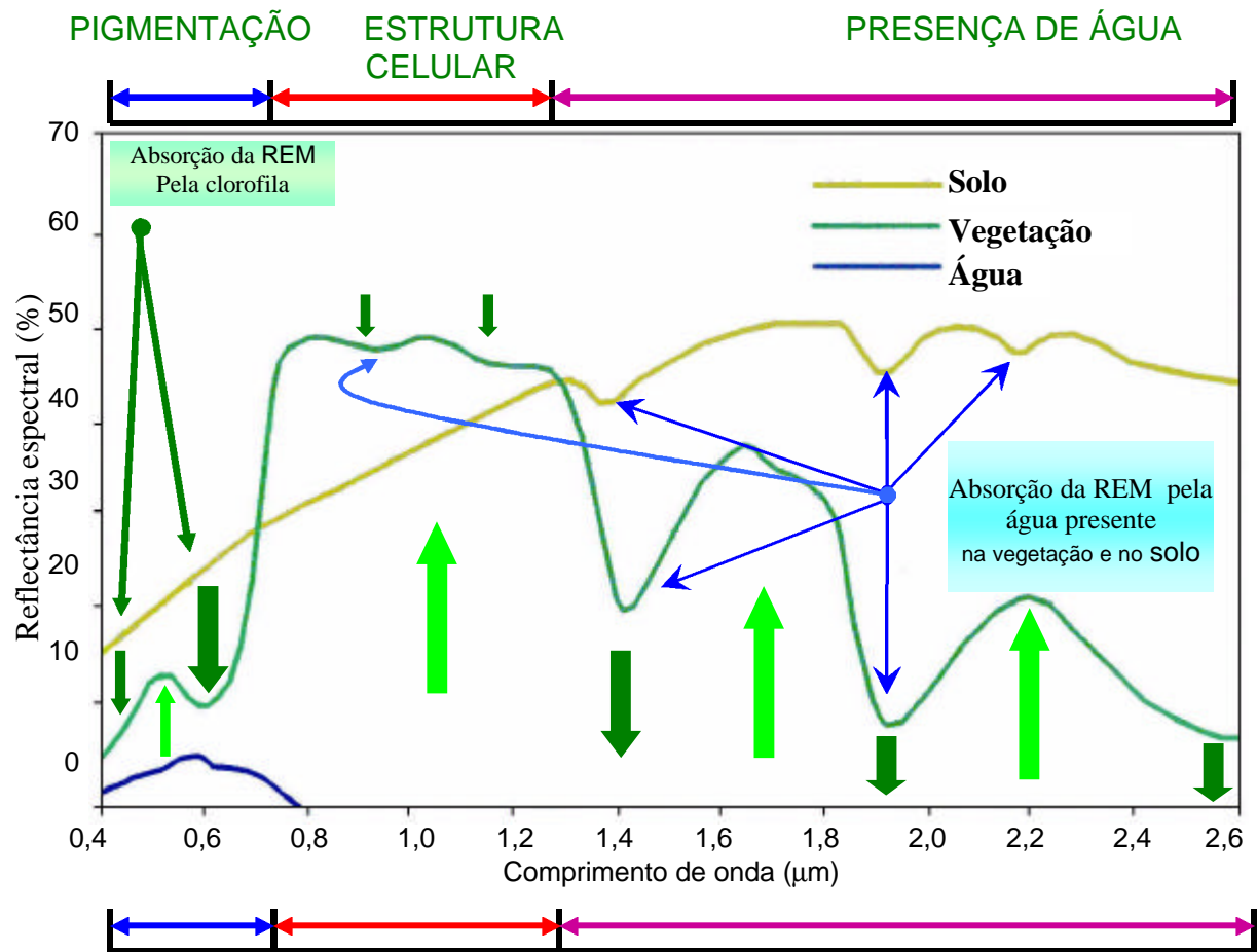
Figura 2.3: Curvas típicas da refletância espectral para os principais alvos da superfície terrestre: solo, água e vegetação. (Fonte: adaptado de Lillesand e Kiefer, 1994).
