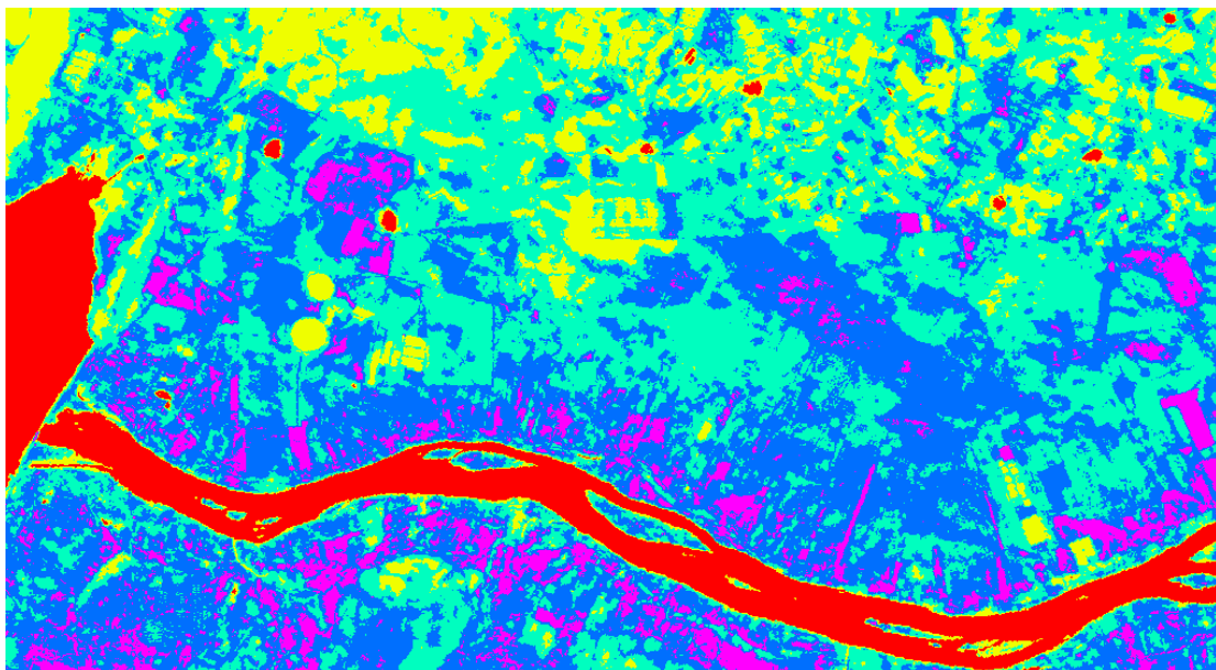
Figura 4.57b - Carta de evapotranspiração (mm/dia) obtida com o Landsat 5 em 04/10/2001
