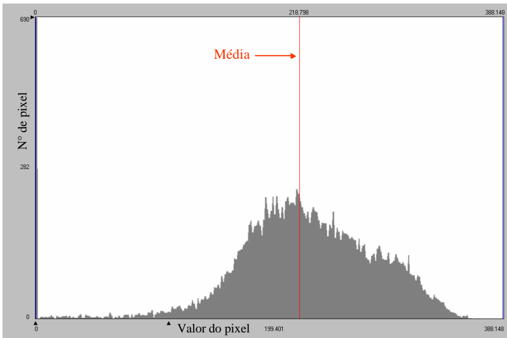
Figura 4.44 - Histograma de frequência do fluxo de calor sensível ( \text{Wm}^{-2} ) obtido com NOAA em 04/10/2001
