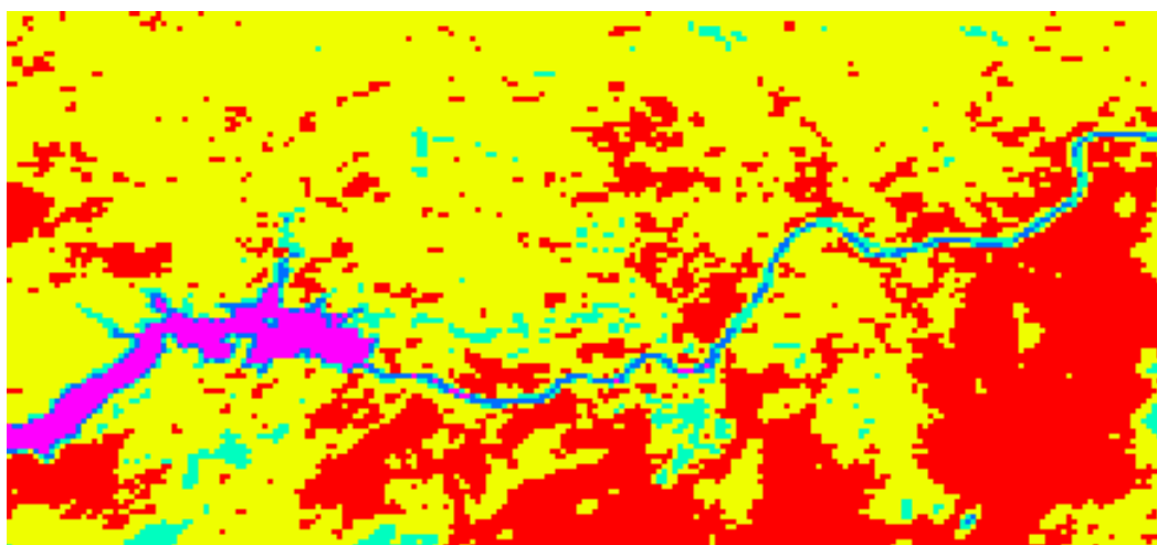
Figura 4.22- Carta da radiação de onda longa emitida pela superfície ( Wm^{-2} ) obtida com o NOAA-16 em 04/10/2001
