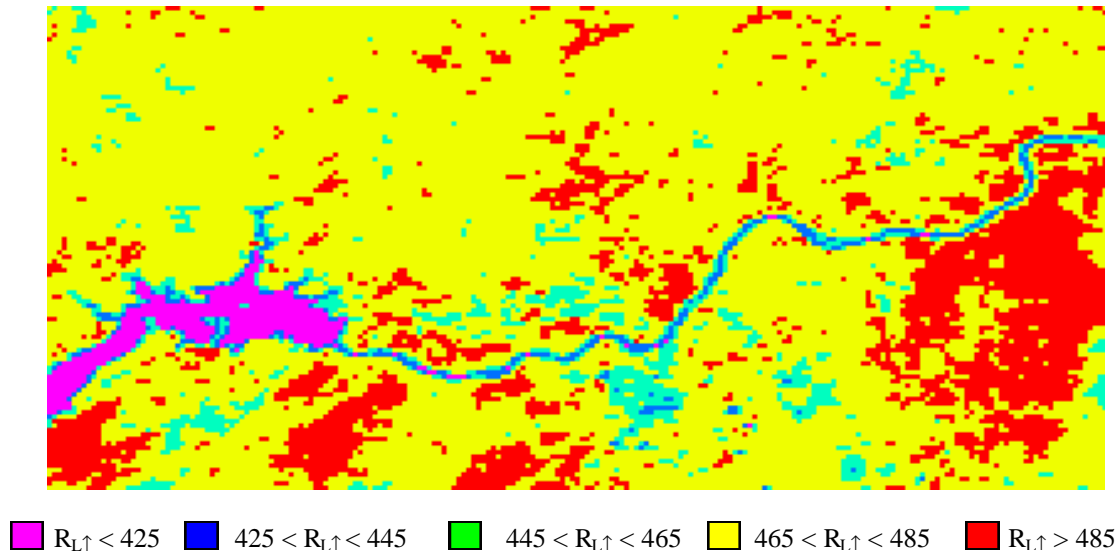
Figura 4.24- Carta da radiação de onda longa emitida pela superfície ( Wm^{-2} ) obtida com o NOAA-16 em 24/09/2003
