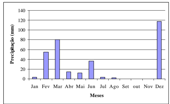
Figura 3.3d- Precipitação mensal em 2000
