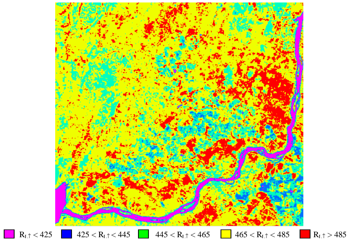
Figura 4.23 - Carta da radiação de onda longa emitida pela superfície ( \text{Wm}^{-2} ) obtido com Landsat 5 em 24/09/2003
