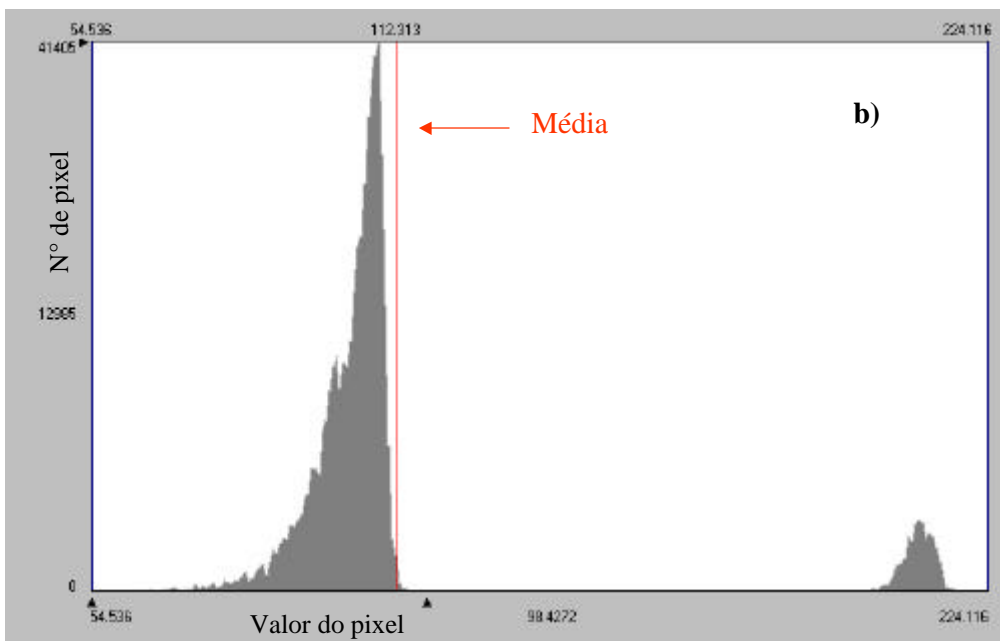
Figura 4.34b - Histograma de frequência do fluxo de calor no solo ( Wm^{-2} ) obtido com o Landsat 5 em 04/10/2001
