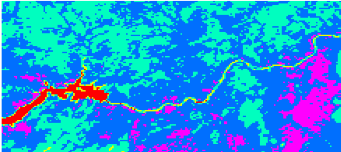
Figura 4.27 - Carta do saldo de radiação ( Wm^{-2} ) obtido com o NOAA-16 em 04/10/2001
