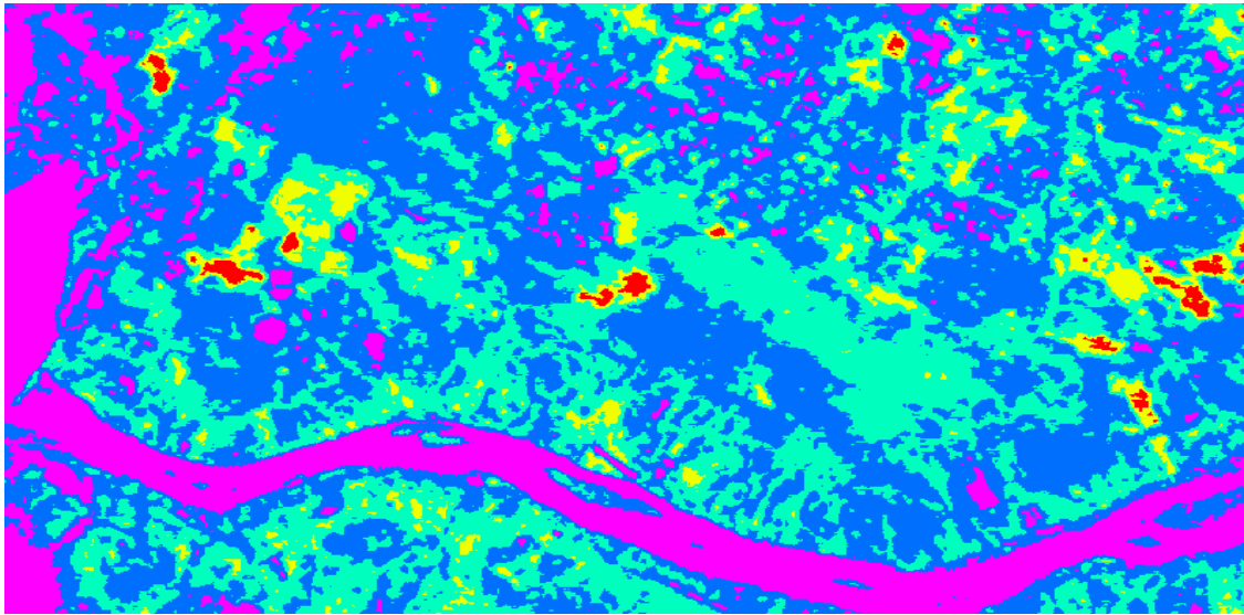
Figura 4.41a - Carta do fluxo de calor sensível ( Wm^{-2} ) obtido com o Landsat 5 em 04/12/2000
