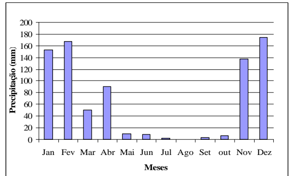
Figura 3.3e- Precipitação mensal em 2001
