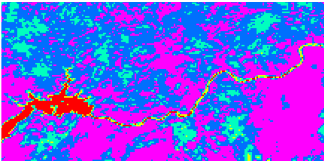
Figura 4.60 - Carta de evapotranspiração (mm/dia) obtida com o NOAA-16 em 24/09/2003
