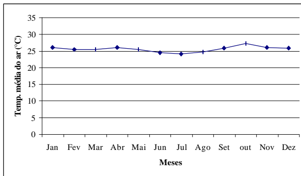
Figura 3.3a – Temperatura média do ar em 2000
