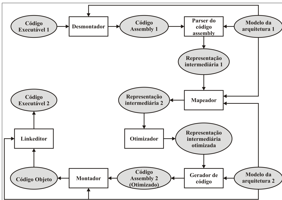
Figura 5.1: Fluxo de tradução binária
