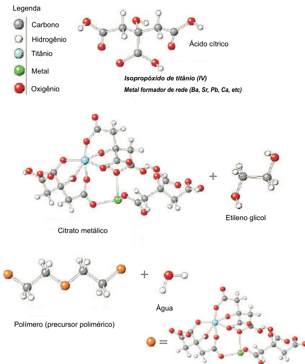
Figura 2.16: Representação esquemática da preparação de uma resina pelo método dos precursores poliméricos 61
