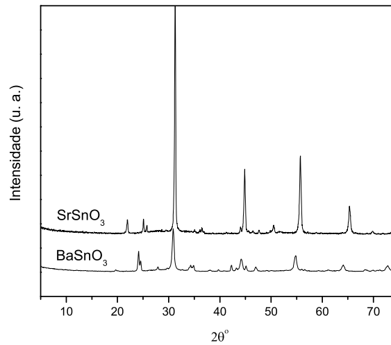
Figura 4.6: Difrátogramas de raios X da evolução estrutural dos sistemas SS e ST calcinados a 700°C/2h
