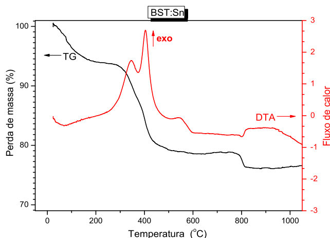
Figura 4.2: Resultados de ATG/ATD dos pós de \text{Ba}_{0,5}\text{Sr}_{0,5}\text{Ti}_{1-x}\text{Sn}_x\text{O}_3 ( x=0,05 ) caracterizado a uma temperatura de 700^\circ\text{C}/4\text{h} .
