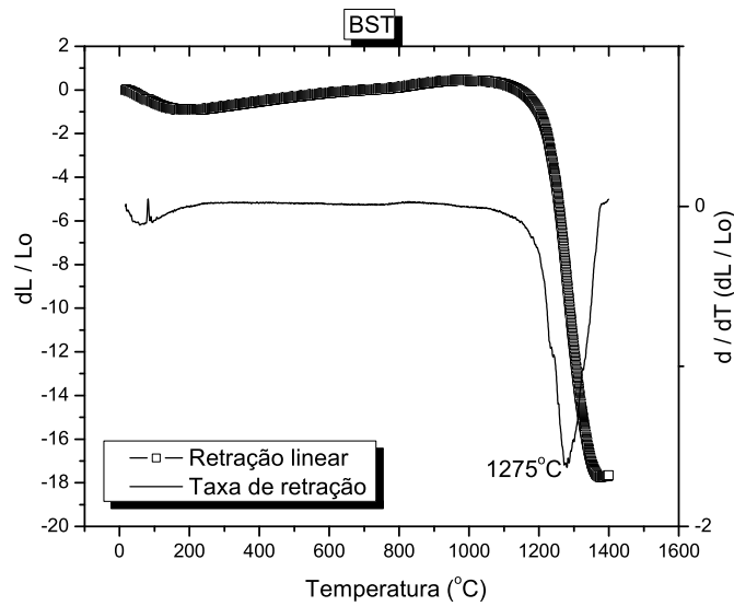
Figura 4.27: Dados obtidos por dilatometria para a amostra \text{Ba}_{0,5}\text{Sr}_{0,5}\text{TiO}_3
