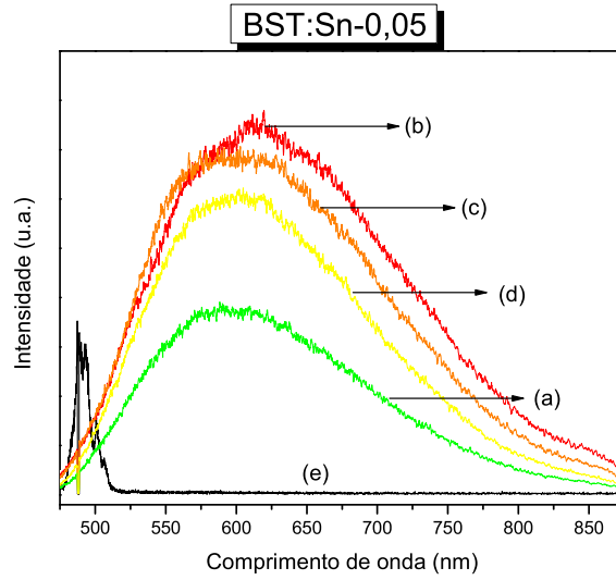
Figura 4.12: Espectro de fotoluminescência para os pós de BST:Sn desordenados calcinados a 300°C, em fluxo de oxigênio, por (a) 20h, (b) 30h, (c) 40h e (d) 50h e (e) cristalino calcinado a 700°C/4h
