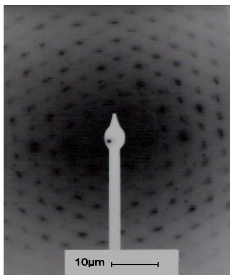
Figura 4.26: Difração de elétrons do BST:Sn-0,20 semi-cristalino (600°C/2h)
