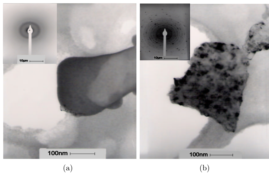
Figura 4.25: Projeção da microestrutura do pó de BST:Sn-0,20 em duas situações diferentes: (a) de-sordenado ( 300^{\circ}\text{C}/30\text{h} ) e (b) cristalino ( 700^{\circ}\text{C}/2\text{h} ), com respectivas difrações de elétrons inseridas
