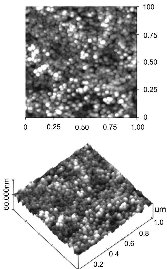
Figura 4.20: Micrografia de força atômica para os filmes finos de BST sobre substrato de Si/SiO 2 /Ti/Pt
