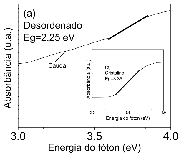
Figura 4.16: Dependência espectral da absorbância para os filmes finos de BST:Sn-0,20 desordenado tratado a 350°C/21h (a) e cristalino tratado a 700°C/2h (b)
