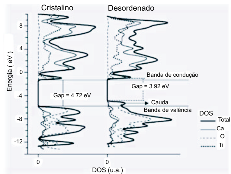
Figura 2.12: Densidade total dos estados para o \text{CaTiO}_3 desordenado e cristalino 38
