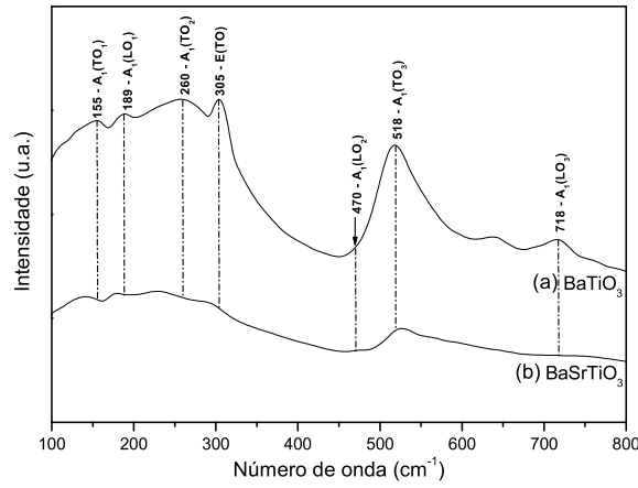
Figura 4.8: Espectroscopia Raman despolarizado a temperatura ambiente para os pós de BT e BST 2
