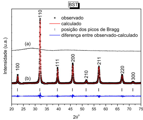
Figura 4.5: (a) XRD para pós BST desordenado calcinado a 300°C para 30h e (b) Gráfico de Rietveld mostrando os difratogramas observado-calculado e as posições do pico de Bragg para BST puro calcinado a 700°C/4h 2
