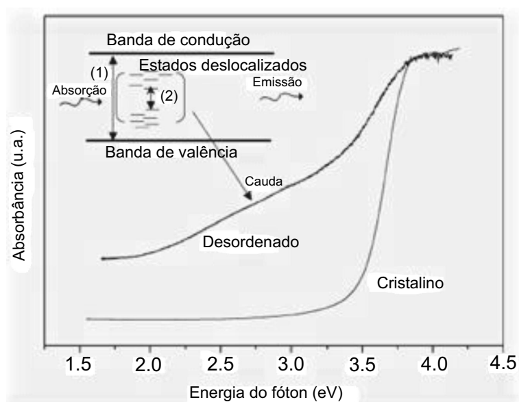
Figura 2.11: Espectro de absorvância de \text{CaTiO}_3 desordenado e cristalino; (1) processo de recombinação direta da energia do “gap” (pouco provável para sólidos cristalinos); (2) provável energia de “gap” para o processo de recombinação 38
