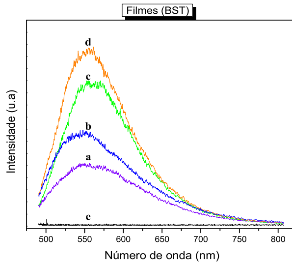
Figura 4.14: Espectro de fotoluminescência dos filmes finos de BST calcinados a 350^{\circ}\text{C} , em atmosfera de oxigênio, por (a) 2h, (b) 4h, (c) 8h e (d) 16h e a (e) 700^{\circ}\text{C}/2\text{h}
