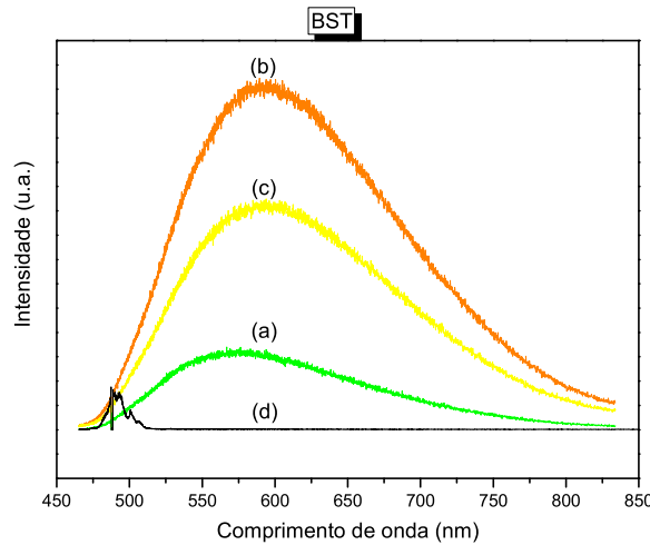
Figura 4.10: Espectro de fotoluminescência para os pós de BST desordenados calcinados a 300^{\circ}\text{C} , em fluxo de oxigênio, por (a) 20h, (b) 30h e (c) 40h, e (d) calcinado a 700^{\circ}\text{C}/4\text{h}^2
