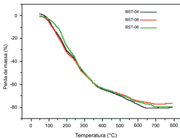
Figura 4.1: Resultado de termogravimetria das resinas de \text{Ba}_x\text{Sr}_{1-x}\text{TiO}_3 ( x = 0,4; 0,6 e 0,8 ) secas a 100^\circ\text{C} , por 10 horas.
