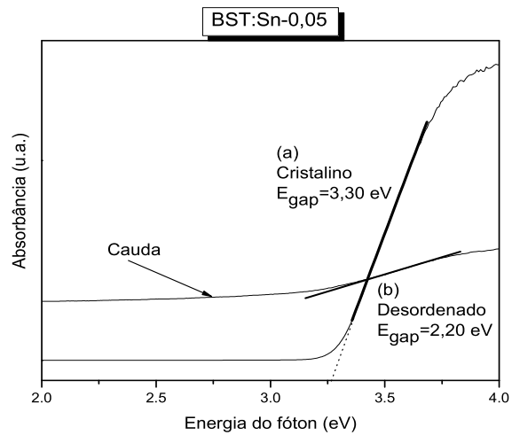
Figura 4.13: Dependência espectral da absorvância para os pós de BST:Sn cristalino ( E_g=3,30\text{eV} ) e BST:Sn desordenado ( E_g=2,20\text{eV} )
