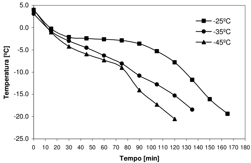
Figura 4.12. Curvas de congelamento para peitos de machos com 30 dias, em diferentes temperaturas de congelamento.
