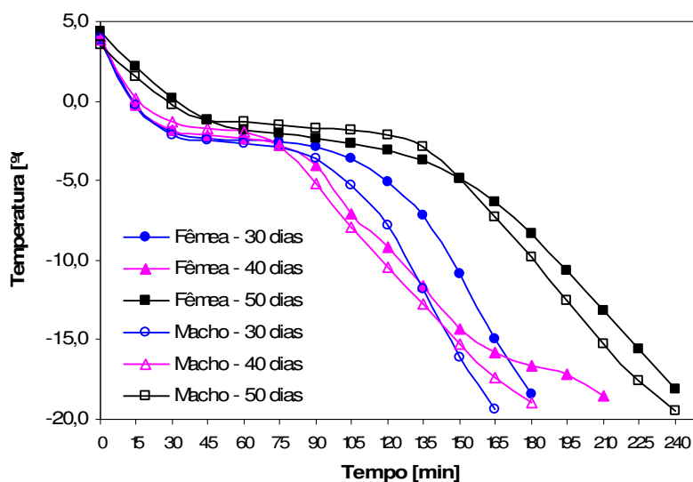
Figura 4.15: Curvas de congelamento para peitos de frango de diferentes idades e sexo obtidos a temperatura de congelamento de -25^{\circ}\text{C} .
