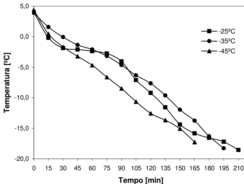
Figura 4.10. Curvas de congelamento para peitos de frango fêmea com 40 dias, em diferentes temperaturas de congelamento.
