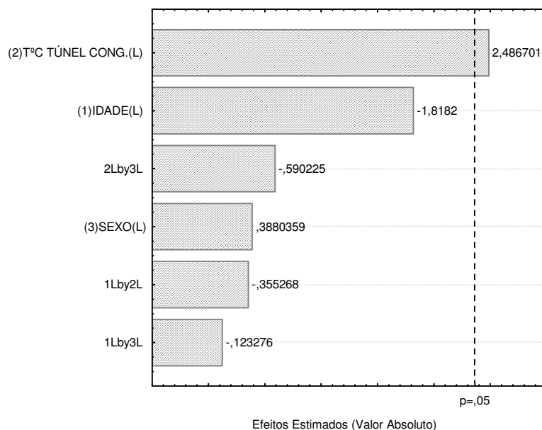
Figura 4.20. Gráfico de Pareto para as análises de cinzas em peitos de frangos machos e fêmeas determinados após o congelamento dos frangos.
