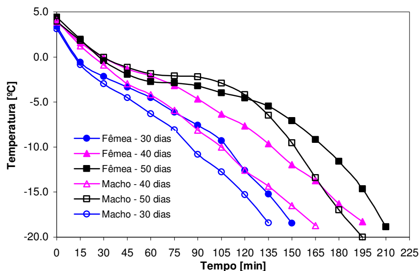
Figura 4.16: Curvas de congelamento para peitos de frango de diferentes idades e sexo obtidos a temperatura de congelamento de -35^{\circ}\text{C}
