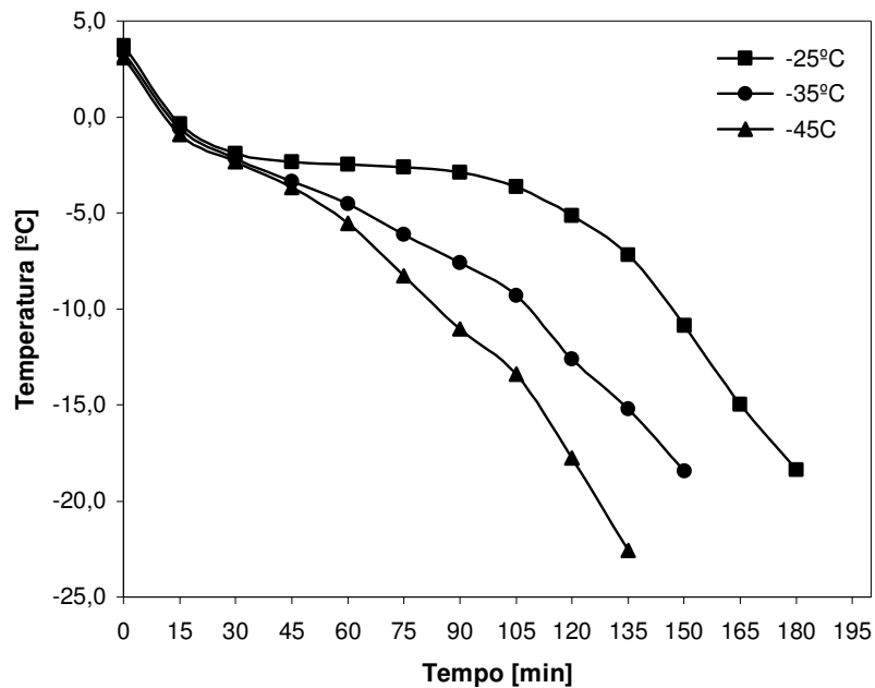
Figura 4.9. Curvas de congelamento para peitos de frango fêmea com 30 dias de idade, em diferentes temperaturas de congelamento.
