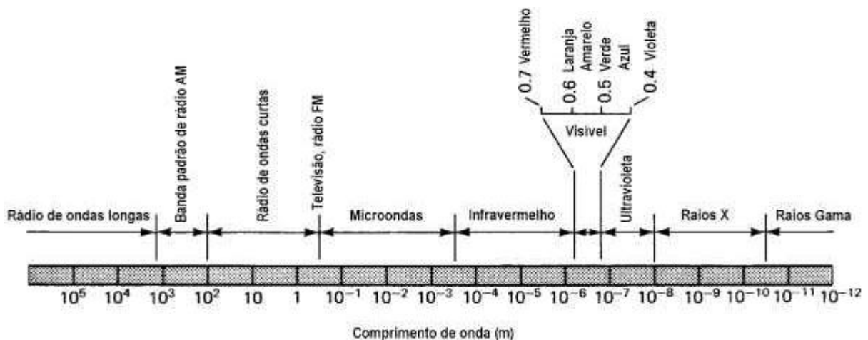
Figura 2.2: Espectro da radiação eletromagnética. Fonte: Barbosa (1996).
