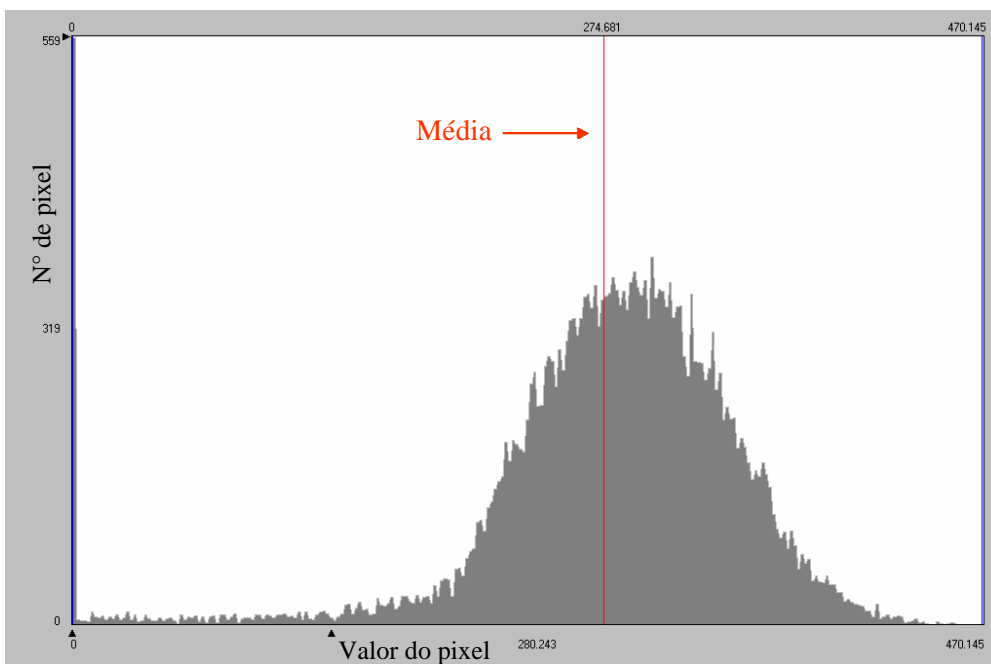
Figura 4.48 - Histograma de frequência do fluxo de calor sensível ( \text{Wm}^{-2} ) obtido com o NOAA-16 em 24/09/2003
