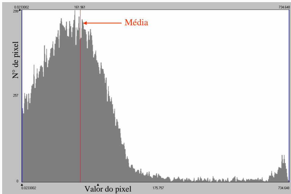
Figura 4.56 - Histograma de frequência do fluxo de calor latente ( \text{Wm}^{-2} ) obtido com o NOAA-16 em 24/09/2003
