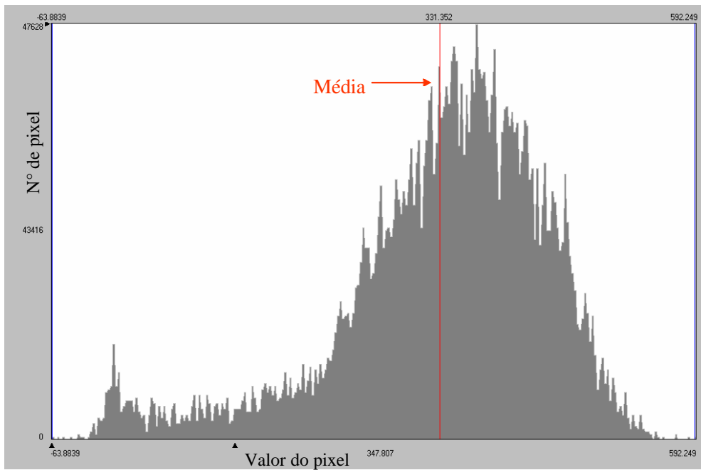
Figura 4.47- Histograma de frequência do fluxo de calor sensível ( \text{Wm}^{-2} ) obtido com o Landsat 5 em 24/09/2003.
