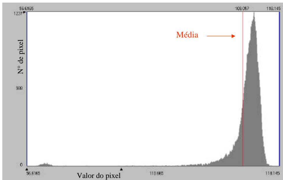
Figura 4.36 - Histograma de frequência de fluxo de calor no solo ( Wm^{-2} ) obtido com o NOAA-16 em 04/10/2001
