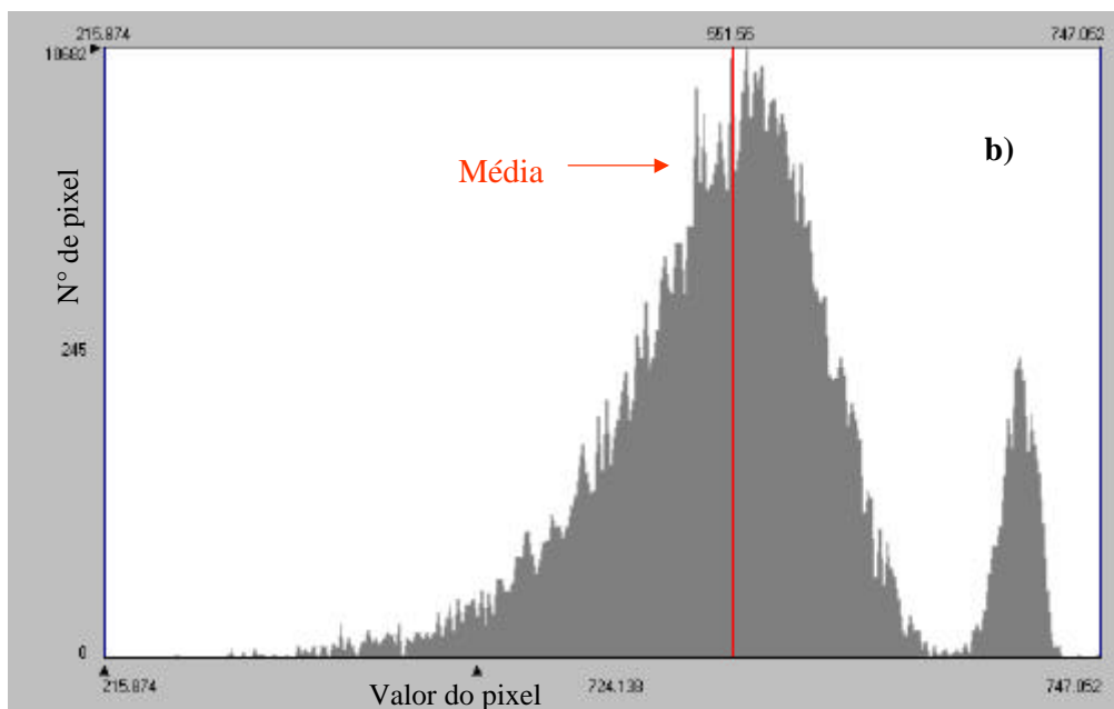
Figura 4.26b - Histograma de frequência do saldo de radiação ( \text{Wm}^{-2} ) obtido com o Landsat 5, em 04/10/2001
