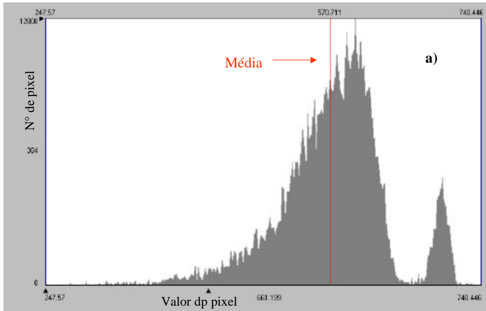
Figura 4.26a – Histograma de frequência do saldo de radiação ( \text{Wm}^{-2} ) obtido com o Landsat 5 em 04/12/2000
