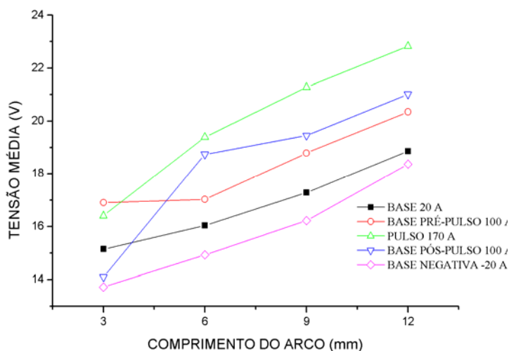
Figura 5.1 - Tensão média em cada intervalo e comprimento de arco.
