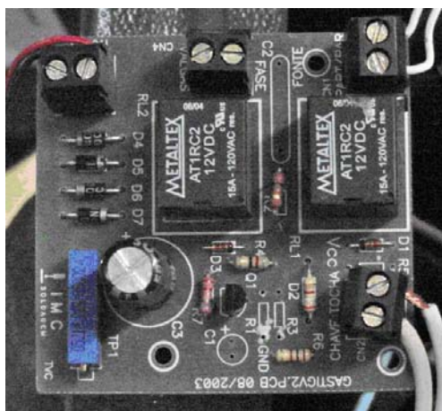
Figura 4.14 – Placa de circuito de controle do retorno do arame
