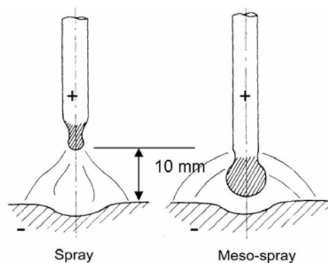
Figura 2.5 - Influência do comprimento do arco na exposição da gota (A5183, \phi 1,6mm, Corrente > 150 A), conforme Kiyohara et al (1979)
