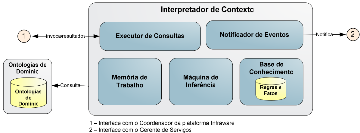
Figura 6-3 – Projeto Conceitual do Interpretador de Contexto
