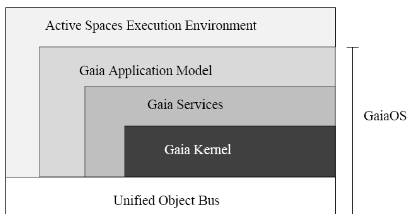
Figura 2-7 - Arquitetura em Camadas do GaioOS.
