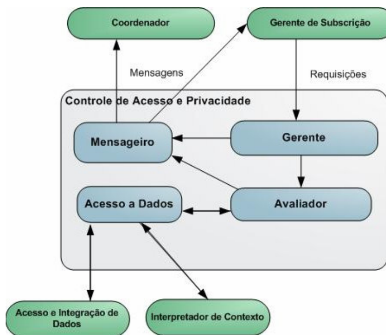
Figura 4-3 – Módulo de Controle de Acesso e Privacidade
