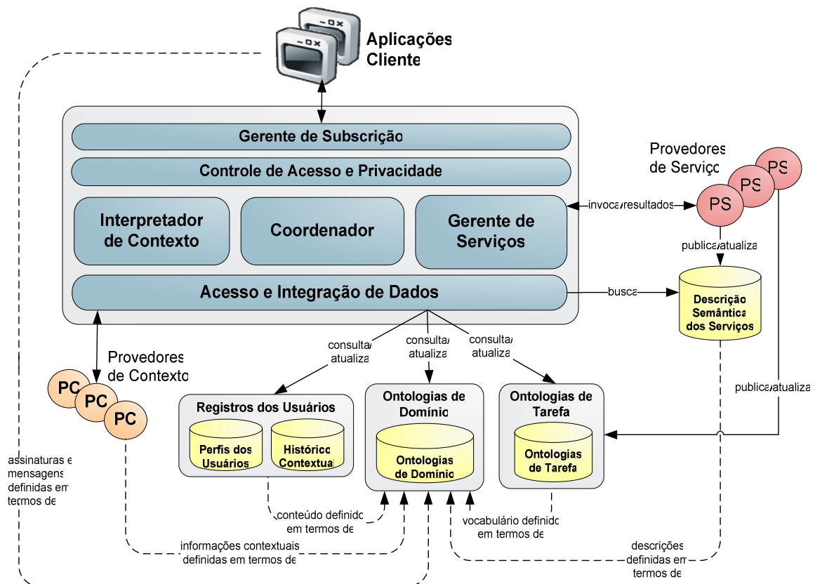
Figura 4-1 – Arquitetura Geral da Plataforma Infracore
