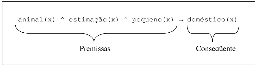
Figura 6-4 – Exemplo de sentença lógica transformada em regra
