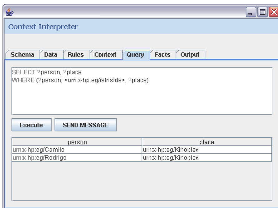
Figura 6-14 – Execução de uma consulta em RDQL
