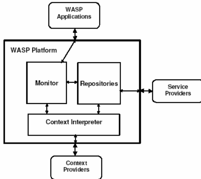
Figura 2-14 - Arquitetura da plataforma WASP.
