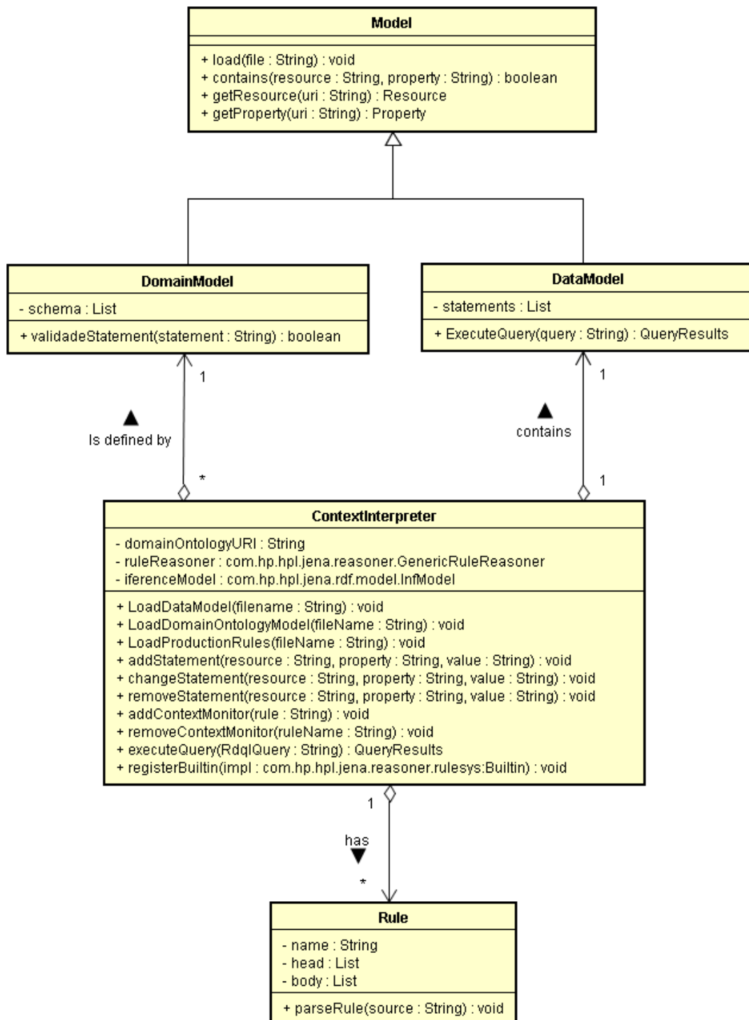
Figura 6-10 – Diagrama de classes utilizadas pelo Interpretador de Contexto
