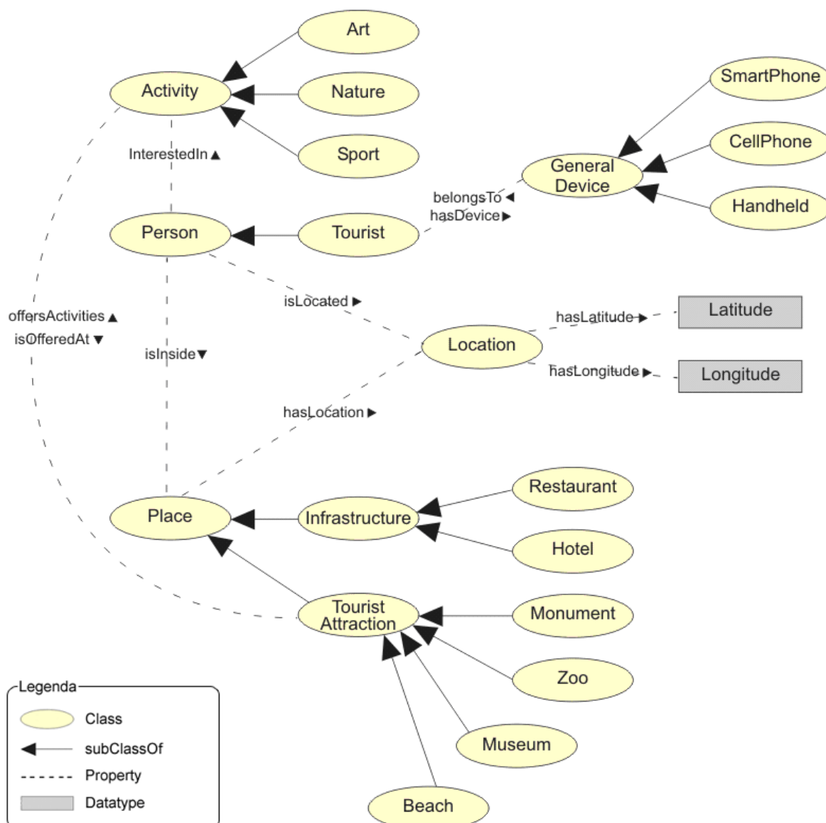
Figura 6-16 – Ontologia simplificada para o domínio do turismo
