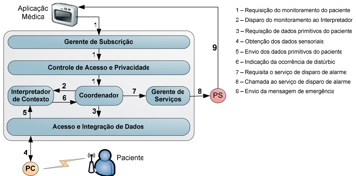
Figura 4-7 – Utilização da plataforma Infracore em um cenário médico-hospitalar
