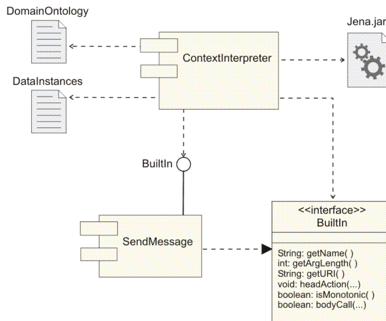
Figura 6-5 – Diagrama de componentes do Interpretador de Contexto
