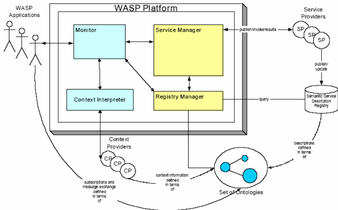
Figura 2-15 – Arquitetura WASP estendida para a utilização de serviços semânticos
