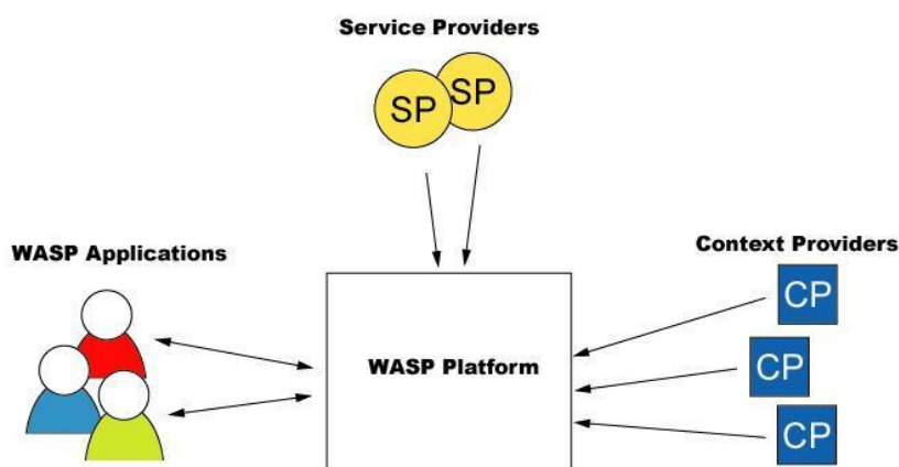
Figura 2-13 - Plataforma WASP e seus relacionamentos.
