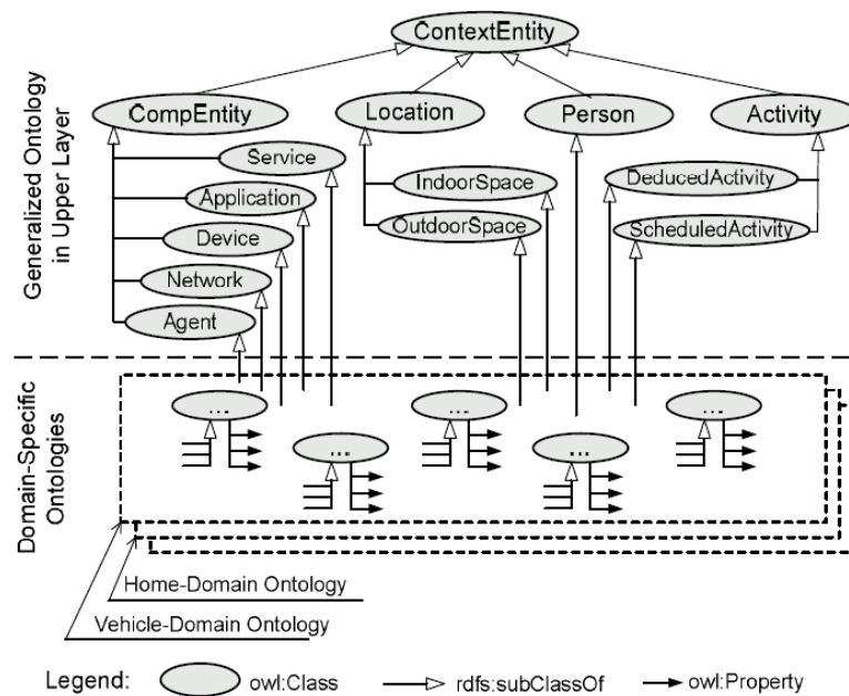
Figura 2-5 – Modelo Ontológico da Arquitetura SOCAM
