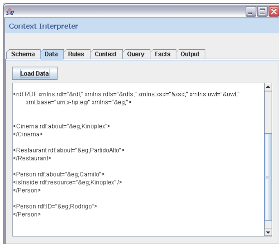
Figura 6-12 – Carga dos indivíduos instanciados
