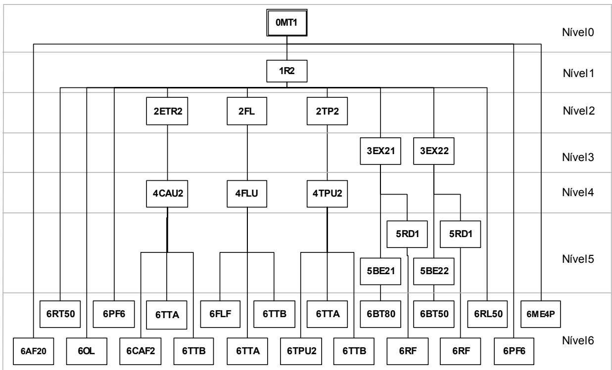
Figura A1.3 – Estrutura do produto Motoredutor 1
