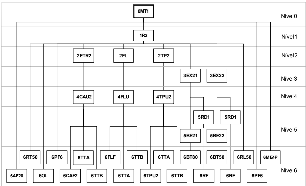
Figura 7.2 – Estrutura do produto Motoreductor 1
