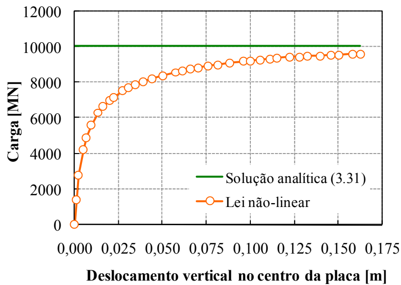
Figura 3.27: Curva carga versus deslocamento vertical.
