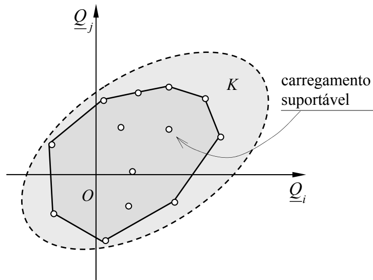
Figura 2.5: Aproximação estática pelo interior.
