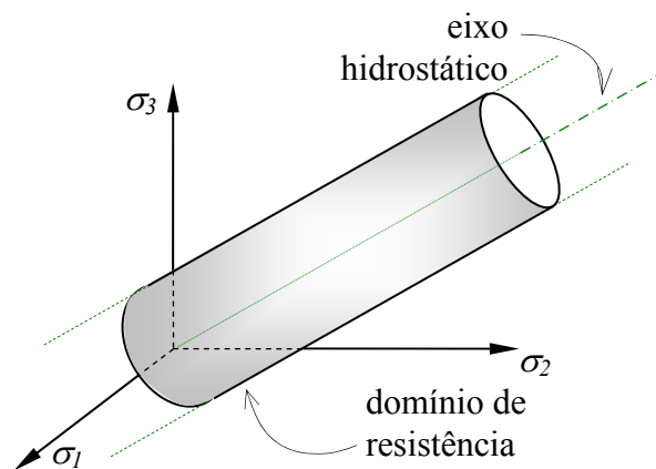
Figura 3.1: Domínio de resistência de von Mises.
