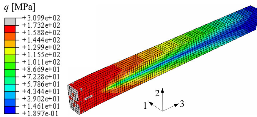
Figura 3.9: Distribuição das tensões equivalentes de von Mises.
