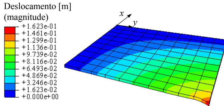
Figura 3.26: Deformada de um quarto da placa.
