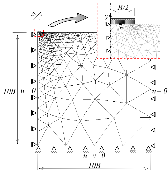
Figura 4.12: Malha de elementos finitos utilizada.
