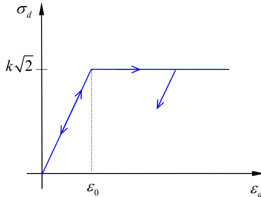
Figura 3.2: Comportamento do material constitutivo.
