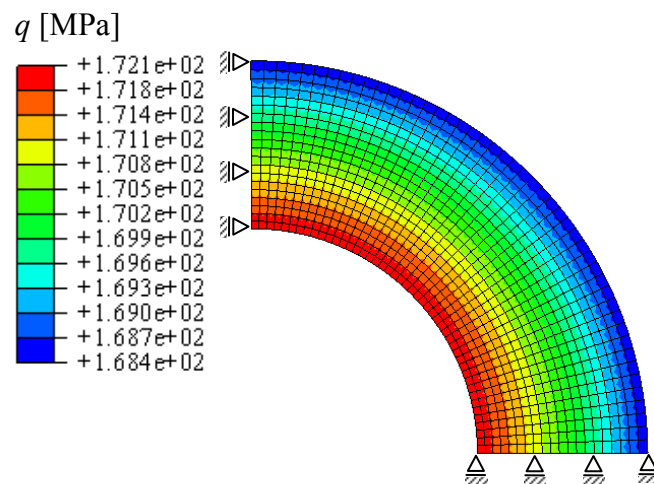
Figura 3.14: Distribuição das tensões equivalentes de von Mises.
