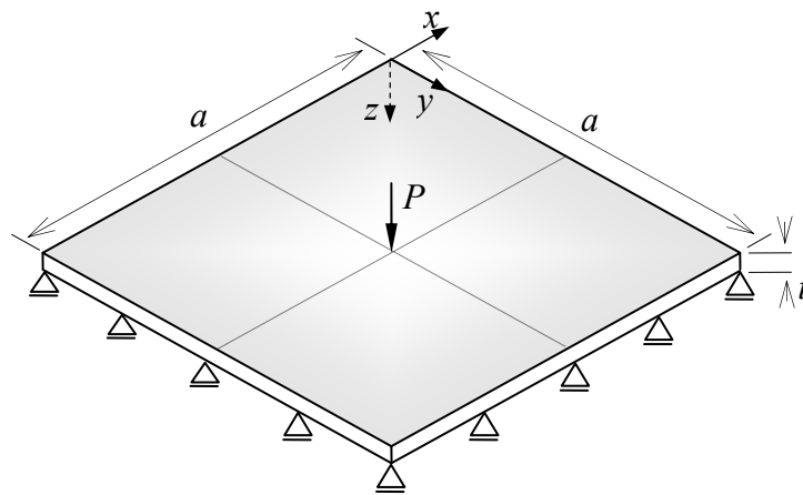
Figura 3.25: Placa quadrada submetida a uma carga concentrada P .
