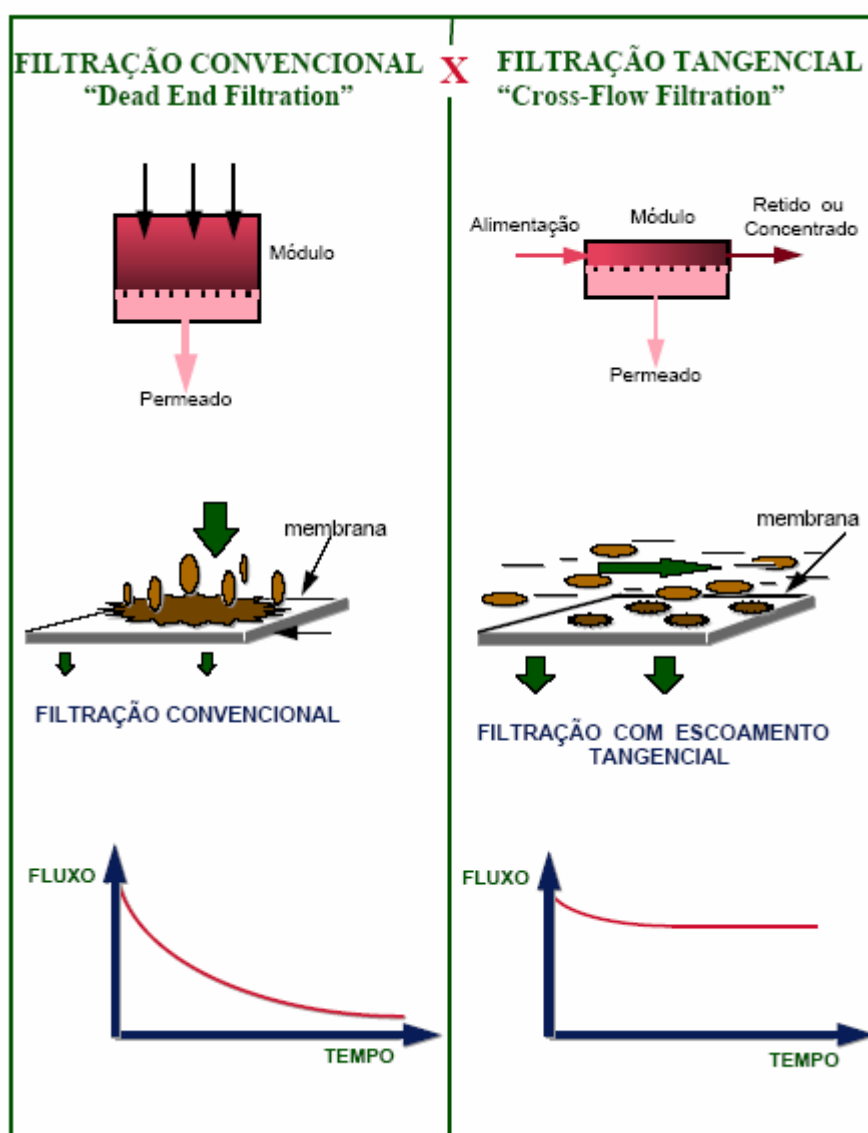
Figura 2.11: Comparação entre filtração convencional e filtração tangencial
