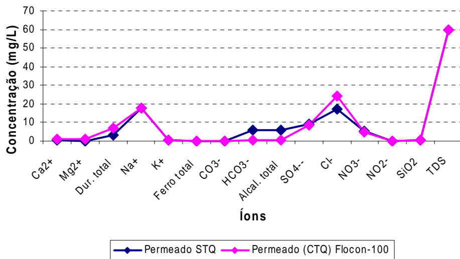
Figura 4.11: Perfil das concentrações do permeado STQ e CTQ (Flocon 100) com a membrana nova
