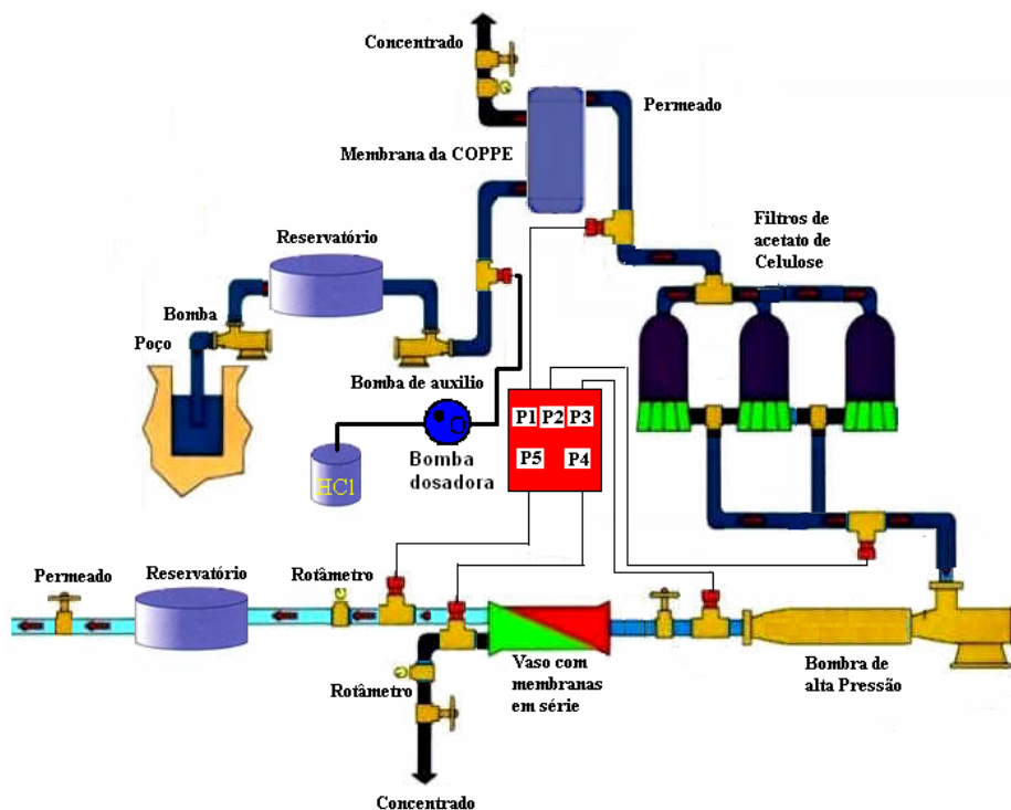
Figura 3.10: Diagrama do Sistema Monitorado da Comunidade do Marinho-PB
