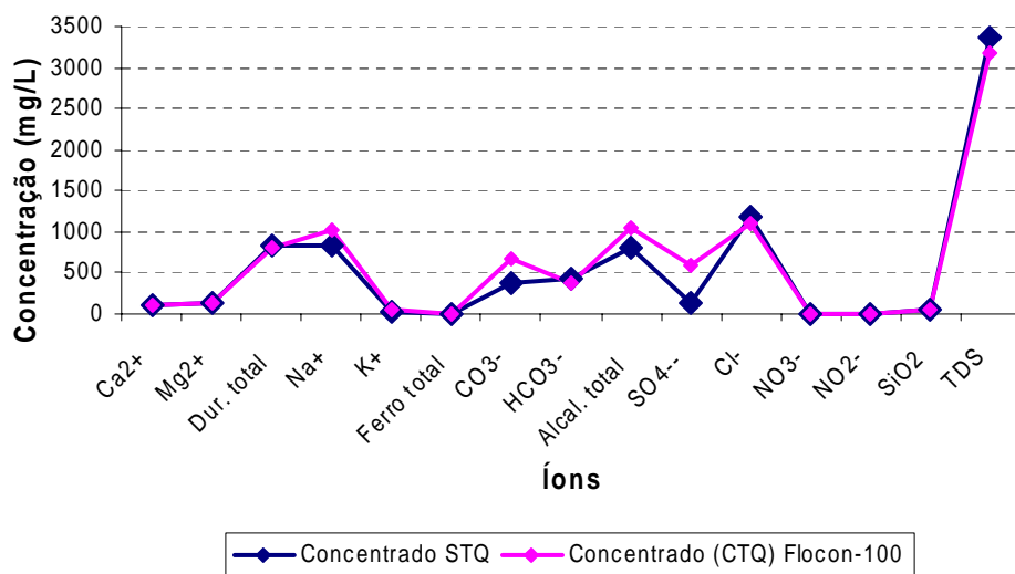
Figura 4.14: Perfil das concentrações do concentrado STQ e CTQ (Flocon 100) com a membrana nova
