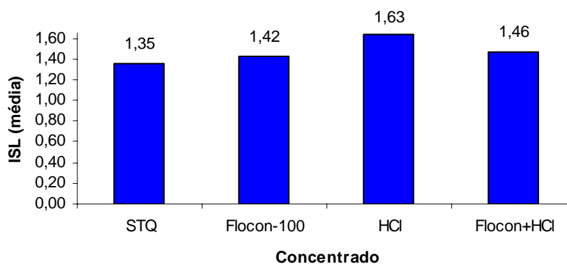
Figura 4.3: Variação do ISL para o concentrado do sistema de dessalinização da comunidade do Marinho-PB em função do pré-tratamento químico aplicado.
