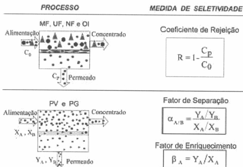
Figura 2.6: Medidas de seletividade em processos com membranas (Habert, et al, 2006)
