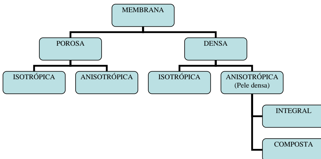
Figura 2.2: Classificação das membranas quanto à morfologia
