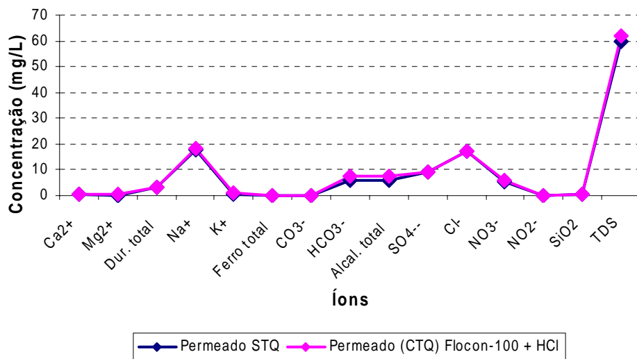
Figura 4.13: Perfil das concentrações do permeado STQ e CTQ (Flocon 100 + HCl) com a membrana nova
