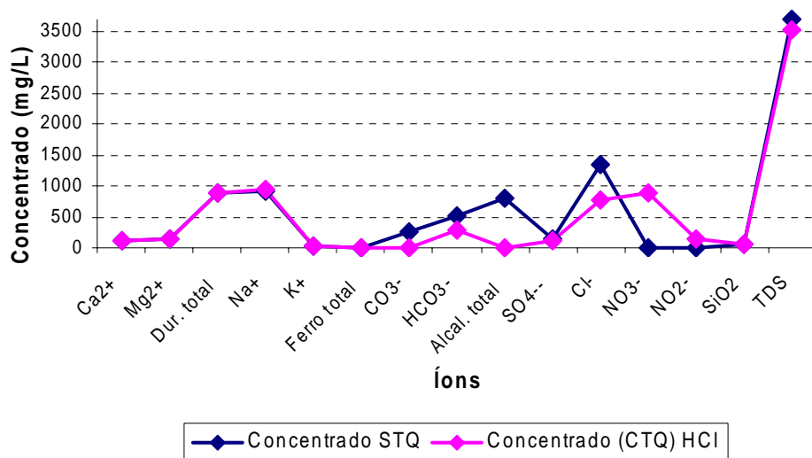
Figura 4.9: Perfil das concentrações do concentrado STQ e CTQ (HCl) com a membrana antiga
