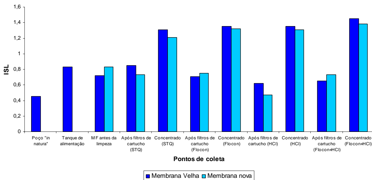
Figura 4.4: Variação do ISL em função da troca das membranas de OI
