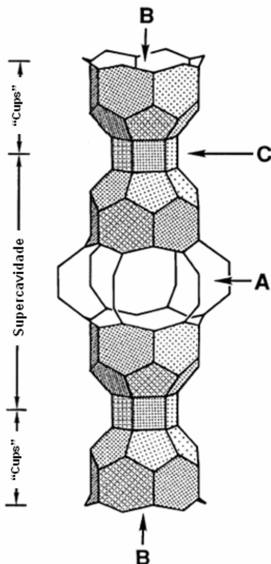
Figura 14: Ilustração esquemática das duas camadas da zeólita MCM-22 mostrando a supercavidade (A) com aberturas de 10 membros e os "cups" externos (B) unidos através dos anéis duplos de 6 membros (prisma hexagonal) (C). Quando duas camadas se unem desse modo, dois "cups" formam a supercavidade. Para maior clareza, somente os átomos T são mostrados.
