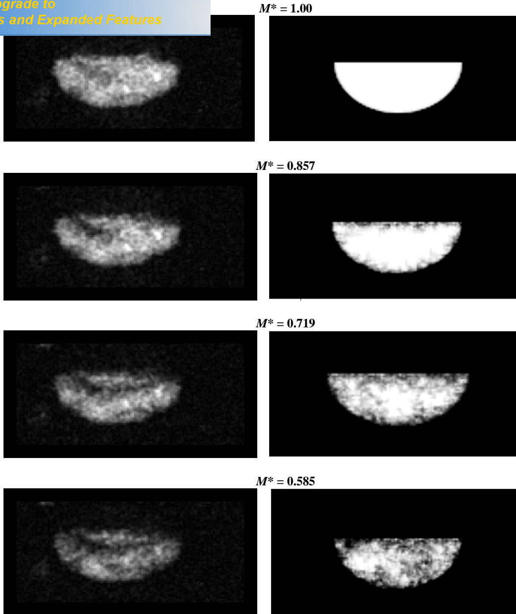
Figura 31 - Evolução no tempo das imagens da gota de água dentro do meio poroso com 120 \mu\text{m} de diâmetro das partículas. Dados experimentais no lado esquerdo (REIS, 2003) e simulação no lado direito.
