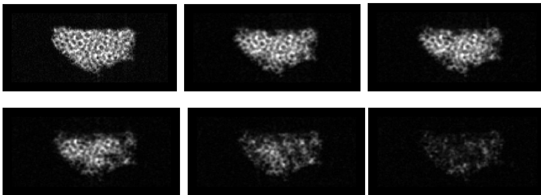
Figura 1 - Imagens de uma gota de líquido absorvida num meio poroso (gota de água de 1,6 mm de diâmetro em um meio poroso composto de esferas de vidro com 400 \mu m de diâmetro). Regiões claras indicam a presença de líquido e a superfície plana na parte superior da gota representa a interface meio poroso/atmosfera (REIS et al., 2003), onde o intervalo de tempo entre as figuras é de aproximadamente 12 minutos.
