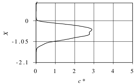
Figura 25 - Evolução no tempo do perfil de concentração de líquido (água) dentro do meio poroso com 400 \mu\text{m} de diâmetro das partículas. Dados experimentais no lado esquerdo (REIS et al, 2003) e simulação no lado direito. O eixo X representa a profundidade da gota em milímetros e o eixo c^* é a concentração adimensional de líquido.
