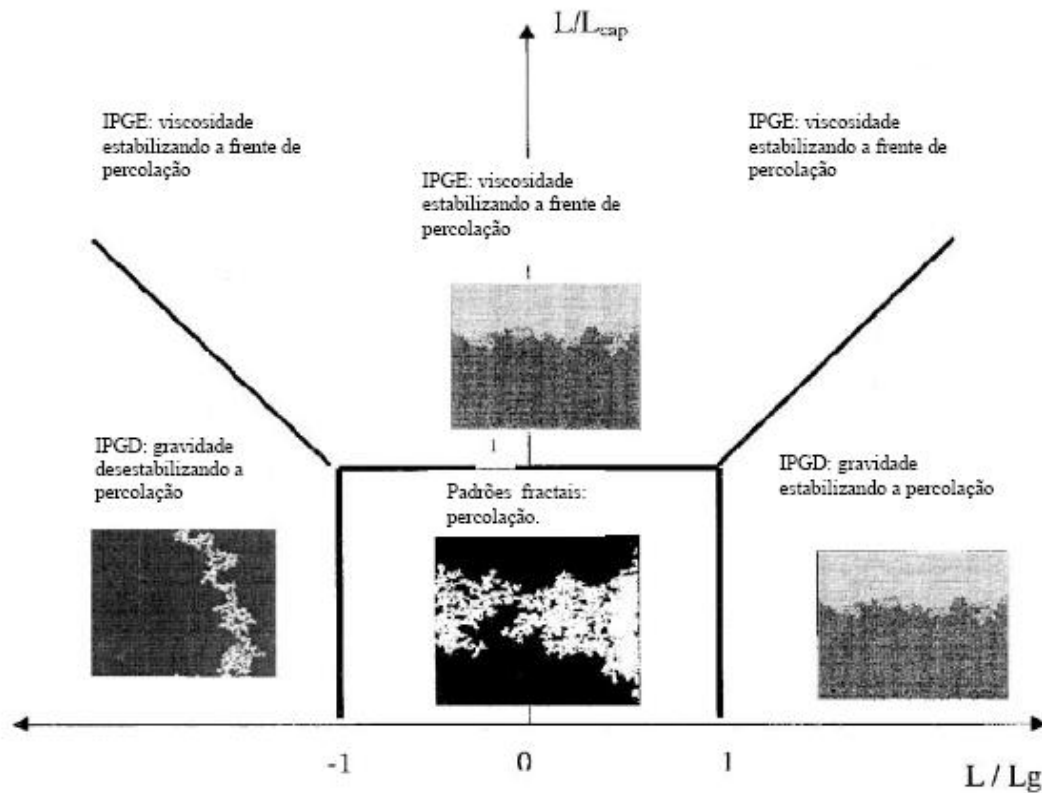
Figura 2 - Diagrama de fase de secagem na ausência dos efeitos dos gradientes térmicos (PLOURD; PRAT, 2003).
