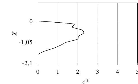
Figura 25 - Evolução no tempo do perfil de concentração de líquido (água) dentro do meio poroso com 400 \mu\text{m} de diâmetro das partículas. Dados experimentais no lado esquerdo (REIS et al, 2003) e simulação no lado direito. O eixo X representa a profundidade da gota em milímetros e o eixo c^* é a concentração adimensional de líquido.
