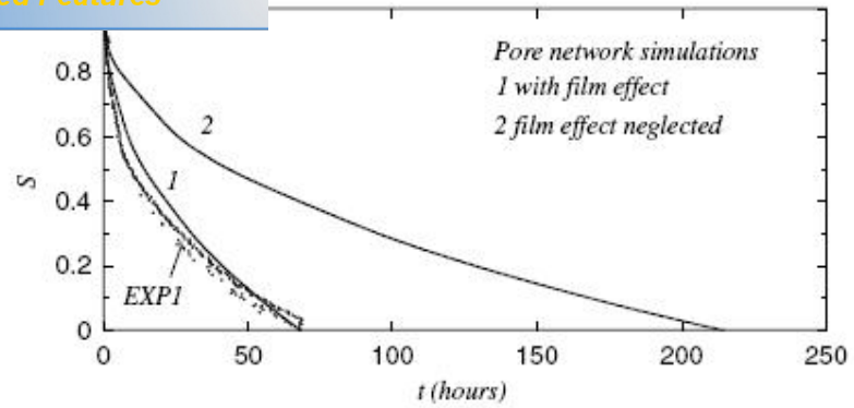
Figura 13 - Curvas de secagem dos experimentos e simulações. S é a saturação do líquido e t o tempo em horas. (PRAT, 2007).
