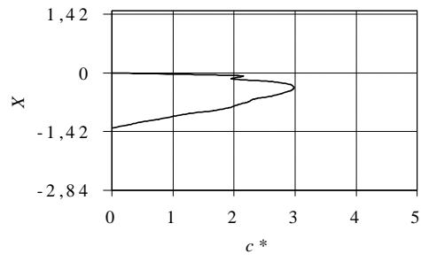
Figura 34 - Evolução no tempo perfil de concentração de líquido (DEM) dentro do meio poroso com 120 \mu\text{m} de diâmetro das partículas e v_f igual a 0.0079. Dados experimentais no lado esquerdo (REIS et al, 2006) e simulação no lado direito.
