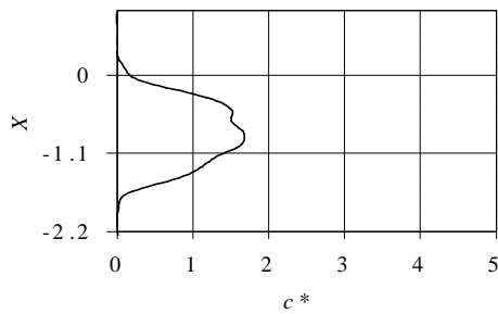
Figura 32 - Evolução no tempo do perfil de concentração de líquido (água) dentro do meio poroso com 120 \mu\text{m} de diâmetro das partículas. Dados experimentais no lado esquerdo (REIS et al, 2003) e simulação no lado direito.
