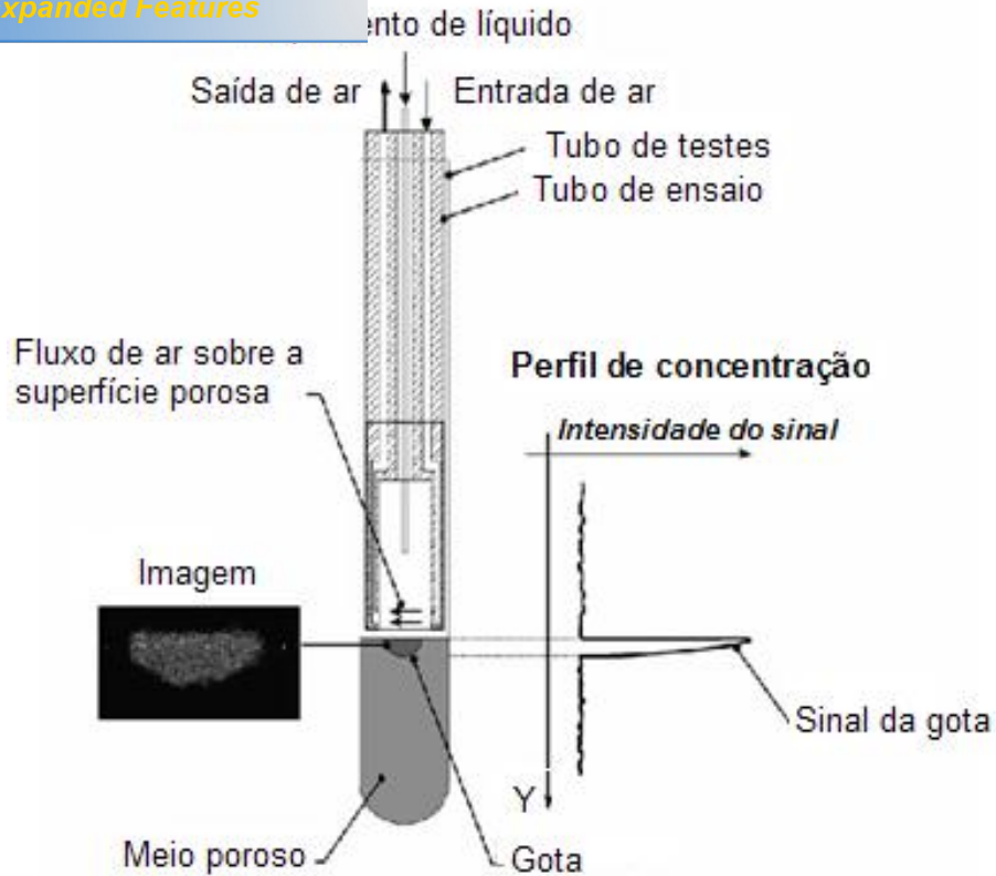
Figura 23 ó Visão lateral da imagem do líquido logo após absorção no substrato e o correspondente perfil de concentração de líquido (REIS et al, 2003).
