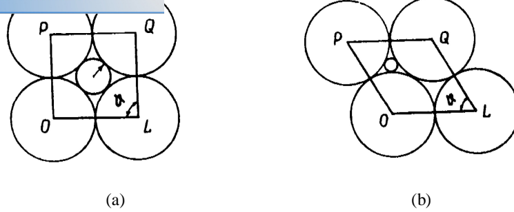
Figura 20 - Compactação das esferas com a formação dos poros. (a) Compactação cúbica ( \vartheta = 90^\circ ). (b) Compactação hexagonal ( \vartheta = 60^\circ ).
