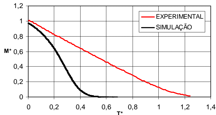
Figura 35 - Fração mássica do líquido remanescente dentro do meio poroso no tempo adimensional para o caso 3.
