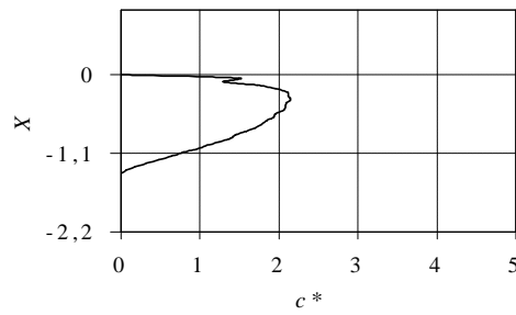
Figura 32 - Evolução no tempo do perfil de concentração de líquido (água) dentro do meio poroso com 120 \mu\text{m} de diâmetro das partículas. Dados experimentais no lado esquerdo (REIS et al, 2003) e simulação no lado direito.
