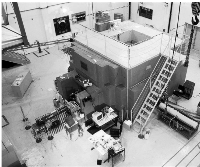
Figura 2.2 - Reator Argonauta.
