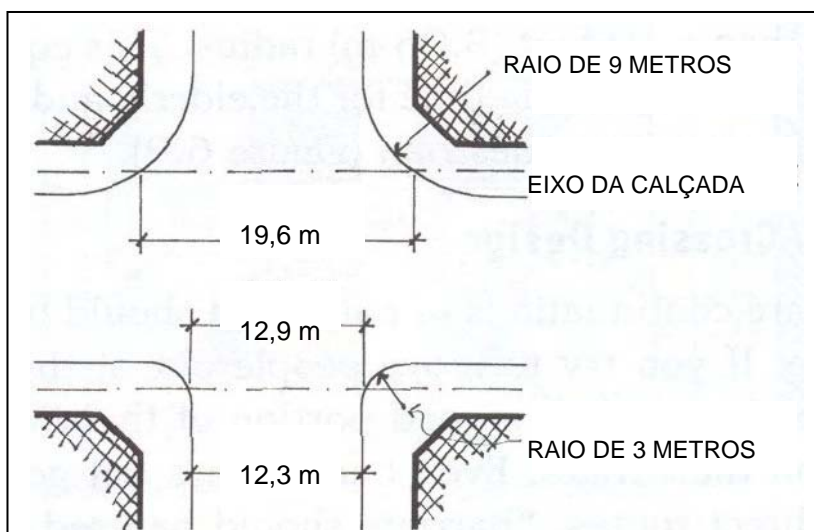
Figura 6.5: Comparação da distância de travessia com diferentes raios de curvatura da calçada junto às esquinas (CHILDS, 1999).
