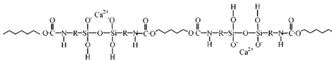
Figura 11: Material híbrido poli(ε-caprolactona)-organosiloxano contendo sais de cálcio.
