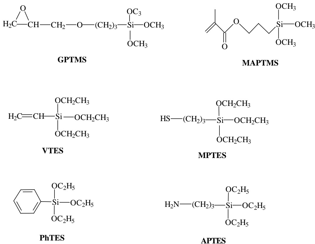
Figura 4: Estruturas de alguns organoalcoxissilanos utilizados como precursores sol-gel no preparo de materiais híbridos. 21
