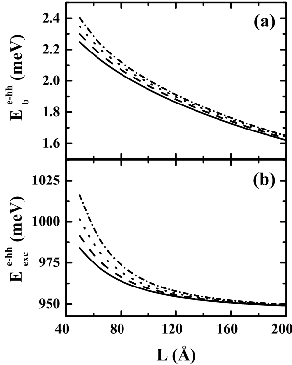
Figura 25: (a) Valores absolutos da energia de ligação e (b) energia total do exciton e-hh em poços quânticos Si/Si_{0.7}Ge_{0.30} tipo-II em função da largura do poço quântico, usando uma função de onda 3D e considerando interfaces abruptas 0 Å (linha sólida), e graduais de 5 Å (linha pontilhada), 10 Å (linha tracejada) e 15 Å (tracejada-pontilhada).
