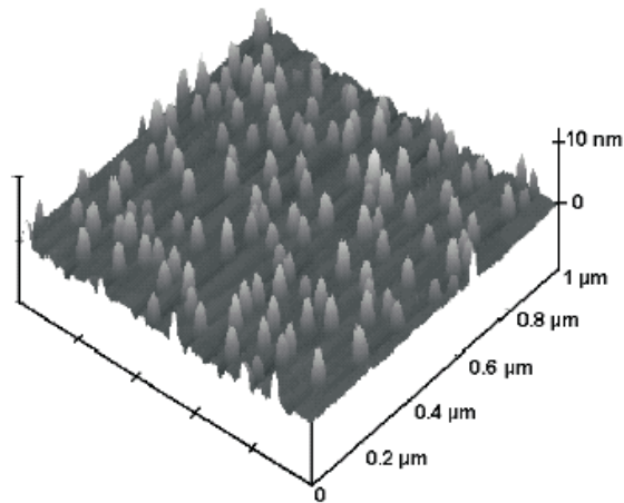
Figura 15: Imagem de pontos quânticos SiGe , crescido em uma camada de Si por MBE, obtida através microscopia de força atômica [48].
