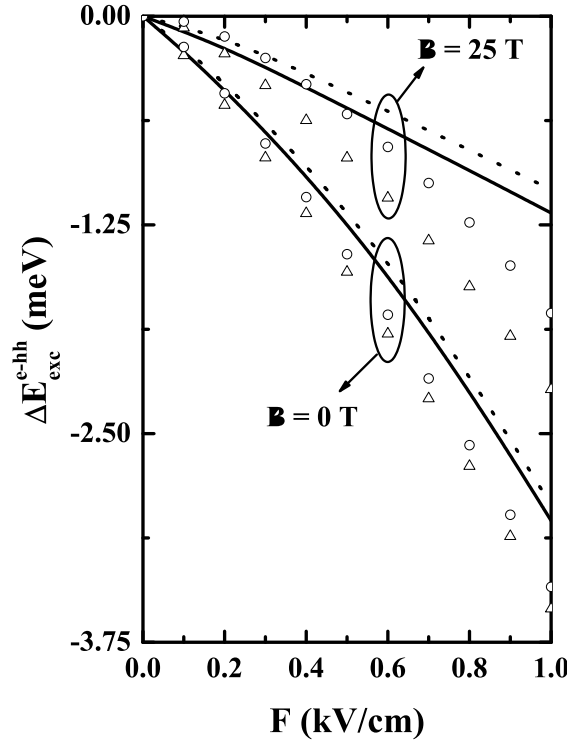
Figura 26: Shift da energia total do exciton como função do campo elétrico em poços quânticos tipo-II Si/Si_{0.7}Ge_{0.30} , para um poço de L = 70 Å de largura, considerando duas possibilidades para a função de onda: 3D (linhas) e 2D (símbolos) com interfaces abruptas (linha sólida) e interface gradual de w = 15 Å (linha pontilhada), para campos magnéticos de B = 0 T e B = 25 T .
