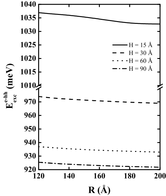
Figura 62: Energia do exciton no estado fundamental em um ponto quântico elipsoidal Si/Si_{0.70}Ge_{0.30} tipo-II em função do raio do QD, sendo a linha sólida para H = 15 \text{ \AA} , a tracejada H = 30 \text{ \AA} , a pontilhada H = 60 \text{ \AA} , e a tracejada-pontilhada H = 90 \text{ \AA} .
