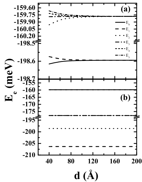
Figura 65: Espectro de energia do elétron em função da distância entre os pontos quânticos para o caso de acoplamento lateral, considerando R_1 = 120 \text{ \AA} e (a) R_2 = 120 \text{ \AA} e (b) 150 \text{ \AA} .
