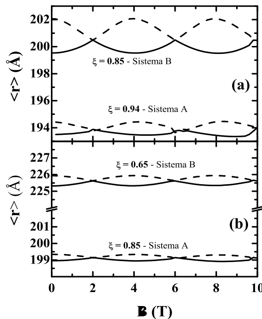
Figura 41: Raio médio do estado fundamental (linha sólida) e primeiro estado excitado (linha tracejada), em função do campo magnético, para o mesmo sistema da Fig. 40.
