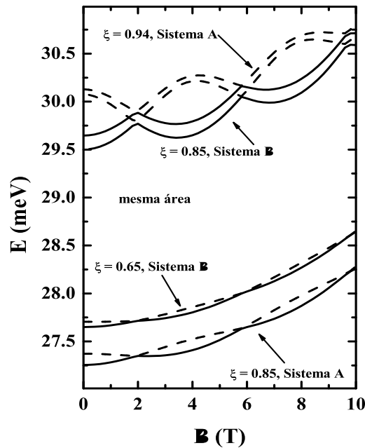
Figura 40: Energia do estado fundamental (linha sólida) e primeiro estado excitado (linha tracejada), em função do campo magnético aplicado, com diferentes valores de excentricidade e considerando os casos onde o anel interno tem simetria cilíndrica e a barreira externa é uma elipse concêntrica (sistema A), e o anel elíptico com mesma excentricidade (sistema B) e mesma área.
