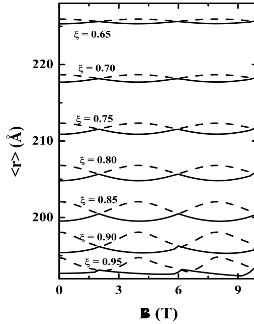
Figura 39: Raio médio do estado fundamental (linha sólida) e primeiro estado excitado (linha tracejada), em função do campo magnético aplicado, para diferentes valores de excentricidade. Para os mesmos parâmetros usado para as Fig. 38.
