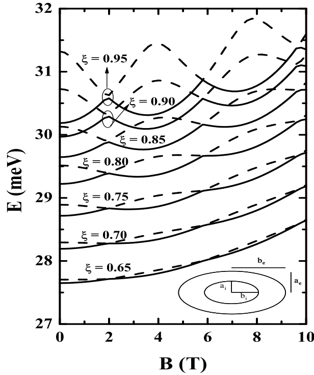
Figura 38: Energia do estado fundamental (linha sólida) e primeiro estado excitado (linha tracejada), em função do campo magnético aplicado, para diferentes valores de excentricidade, R_I = 140 \text{ \AA} , e R_E = 240 \text{ \AA} .
