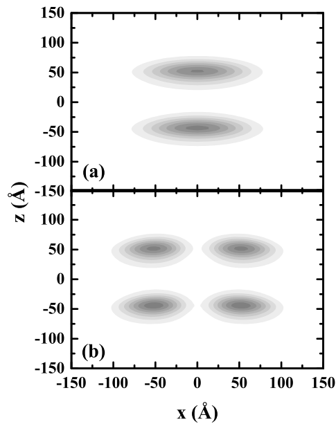
Figura 69: Funções de onda para o (a) estado fundamental e (b) terceiro estado excitado, para o caso de dois pontos acoplados verticalmente, considerando o mesmo raio R_1 = R_2 = 120 \text{ \AA} .
