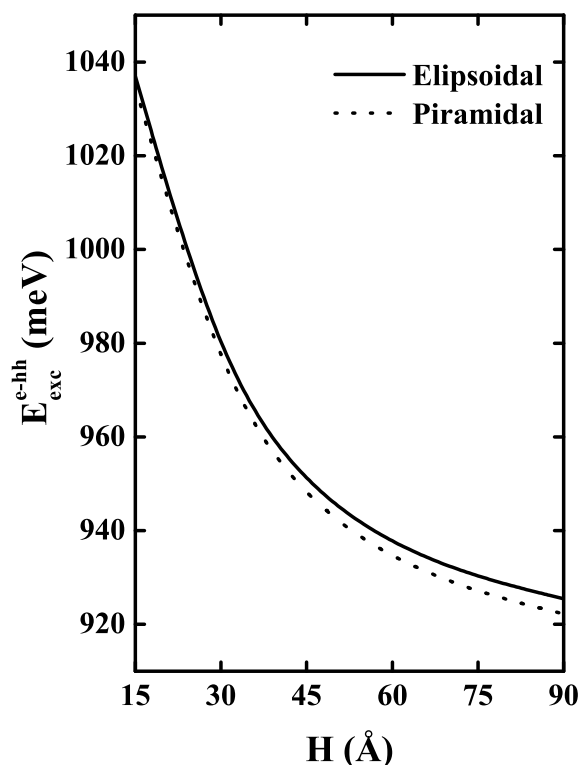
Figura 61: Energia do exciton no estado fundamental em pontos quânticos elipsoidais (linha sólida) e piramidais (linha pontilhada).
