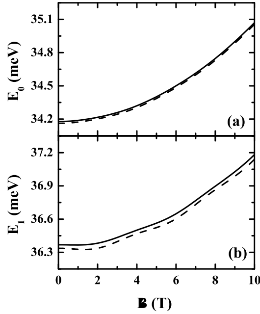
Figura 32: Energia do (a) estado fundamental e (b) primeiro estado excitado, em função do campo magnético aplicado, para uma impureza hidrogênica negativa em duas distâncias diferentes z_i do plano do anel: z_1 = 10 \text{ \AA} (linha sólida) e z_2 = 30 \text{ \AA} (linha tracejada), para os mesmos parâmetros do anel na Fig. 30.
