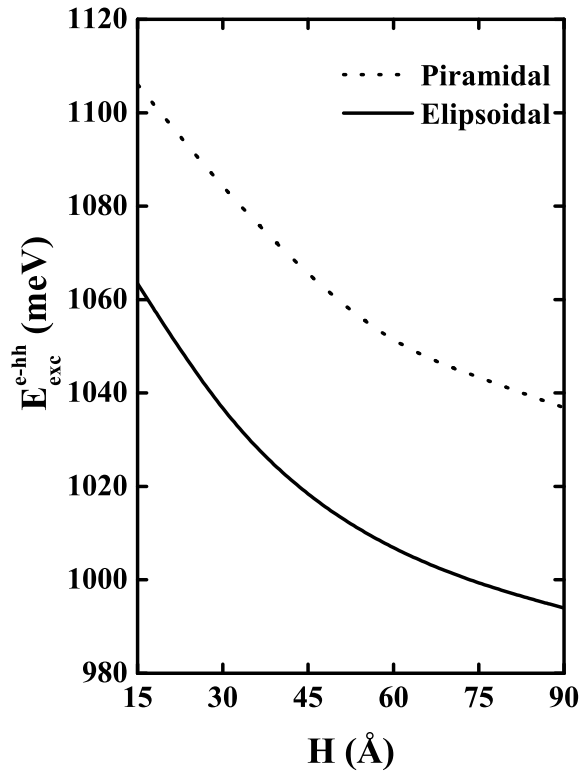
Figura 57: Energia do exciton elétron-buraco pesado ( e - hh ) no estado fundamental em pontos quânticos elipsoidais (linha sólida) e piramidais (linha pontilhada).
