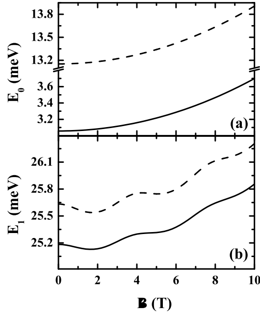
Figura 30: Energia do (a) estado fundamental e (b) primeiro estado excitado, em função do campo magnético aplicado, para uma impureza hidrogênica positiva em duas distâncias diferentes do plano do anel z_i , z_1 = 10 \text{ \AA} (linha sólida) e z_2 = 30 \text{ \AA} (linha tracejada), com a = 140 \text{ \AA} e b = 240 \text{ \AA} .
