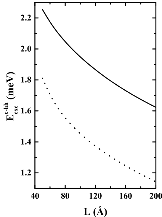
Figura 24: Valores absolutos da energia de ligação dos excitons em poços quânticos Si/Si_{0.70}Ge_{0.30} tipo-II abruptos como função da largura do poço, considerando as aproximações 2D (linha pontilhada) e 3D (linha sólida) para a função de onda.
