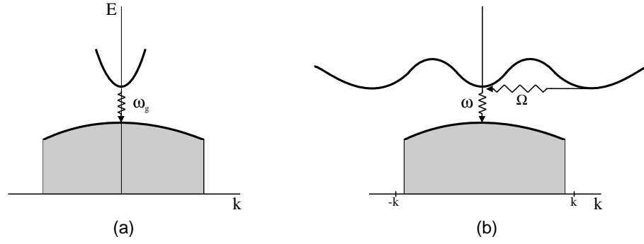
Figura 5: (a) Transição de gap direto, neste caso, a transição através do gap ocorre com a emissão de um fóton de frequência \omega_g = E_g/\hbar e com vetor de onda desprezível na escala da figura. (b) No semiconductor de gap indireto, a transição através do gap envolve um fóton de frequência \omega \approx \omega_g e \kappa \approx 0 e um fônon com frequência \Omega muito menor que \omega_g e vetor de onda \omega_g e \kappa \simeq \kappa_{KZ} , de tal forma a conservar energia e momentum totais.
