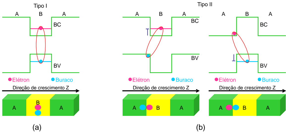
Figura 17: Representação esquemática do alinhamento de bandas tipo-I e tipo-II.
