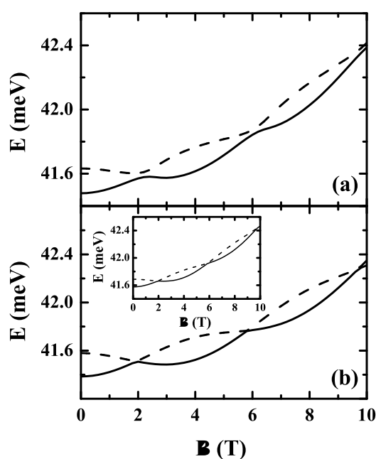
Figura 36: Energia do estado fundamental (linha sólida) e primeiro estado excitado (linha tracejada), com duas impurezas hidrogênicas negativas próximo ao anel quântico de tamanho a = 140 \text{ \AA} e b = 240 \text{ \AA} com a primeira impureza localizada em \vec{r}_{imp}^{(1)} = (190 \text{ \AA}, 0, z_1) e a segunda em \vec{r}_{imp}^{(2)} = (-190 \text{ \AA}, 0, z_2) . Em (a) z_1 = 10 \text{ \AA} e z_2 = 30 \text{ \AA} , (b) z_1 = z_2 = 30 \text{ \AA} e z_1 = z_2 = 10 \text{ \AA} no inset , respectivamente.
