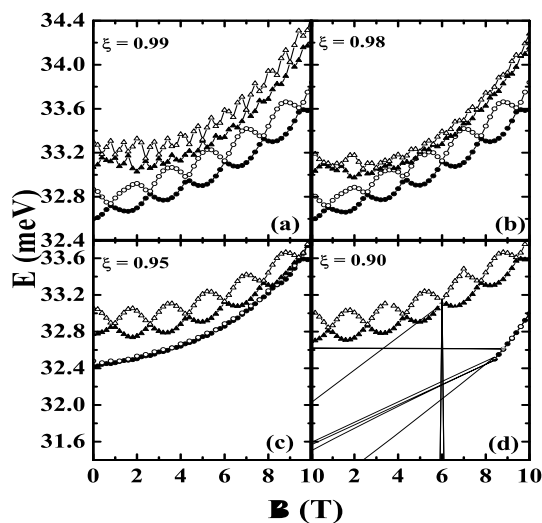
Figura 54: Espectro da energia em função do campo magnético, considerando ambos anéis, interno e externo, como sendo elíptico, com \xi = 0.99 (a), \xi = 0.98 (b), \xi = 0.95 (c) e \xi = 0.90 (d).
