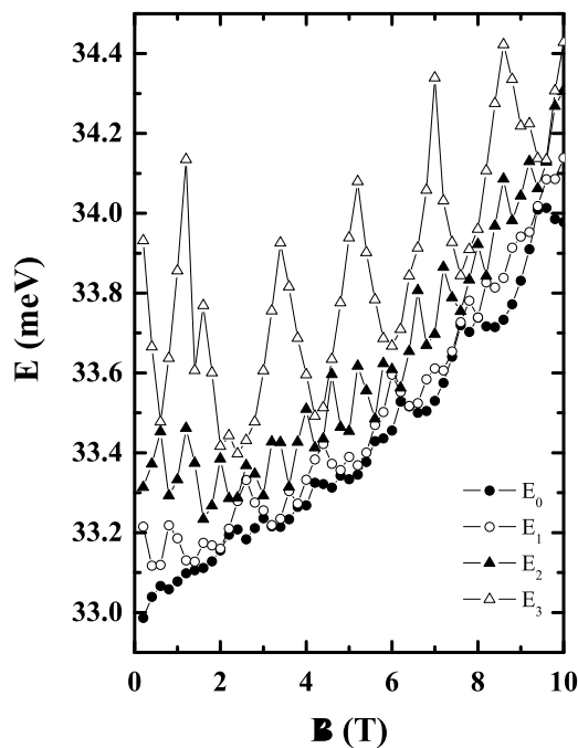
Figura 48: Espectro de energia em função do campo magnético em um anel duplo com geometria circular, com R_{1,j} = 230 \text{ \AA} , R_{1,e} = 330 \text{ \AA} , R_{2,j} = 400 \text{ \AA} e R_{2,e} = 500 \text{ \AA} .
