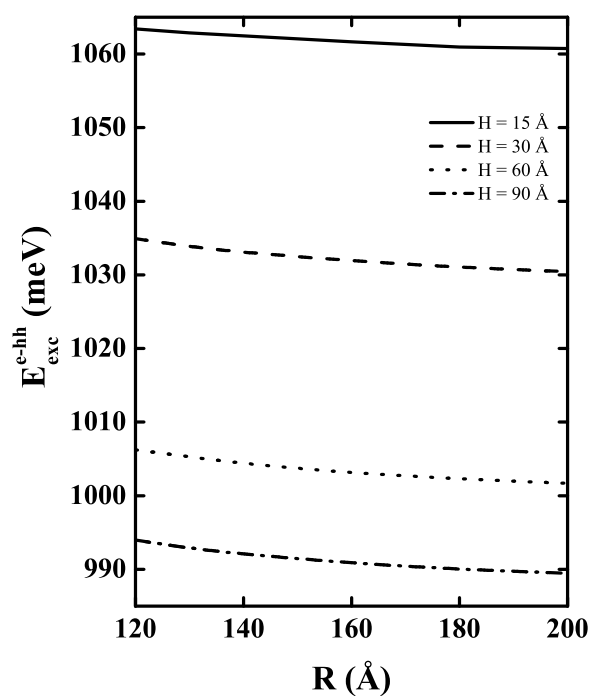
Figura 58: Energia do exciton no estado fundamental em um ponto quântico elipsoidal Si/Si_{0.85}Ge_{0.15} tipo-I em função do raio do QD, sendo a linha sólida para H = 15 \text{ \AA} , a tracejada H = 30 \text{ \AA} , a pontilhada H = 60 \text{ \AA} , e a tracejada-pontilhada H = 90 \text{ \AA} .
