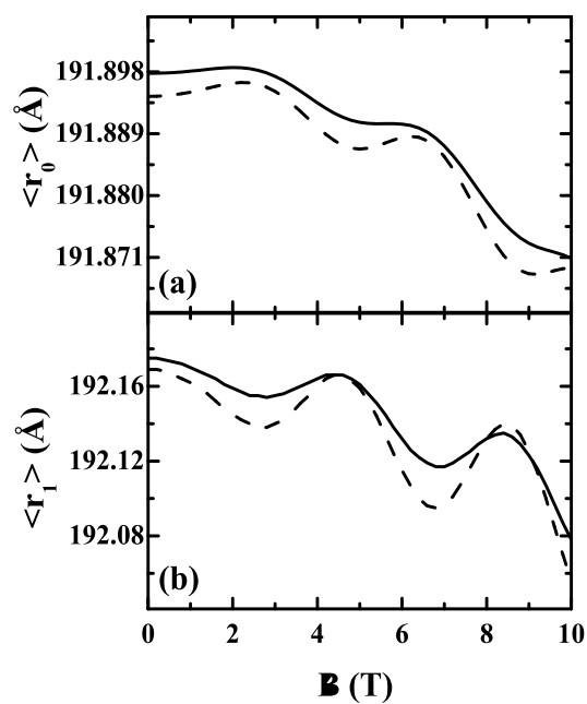
Figura 33: Raio médio do (a) estado fundamental e (b) primeiro estado excitado, em função do campo magnético aplicado, para uma impureza hidrogênica negativa em duas distâncias diferentes do plano do anel: z_1 = 10 Å (linha sólida) e z_2 = 30 Å (linha tracejada) para os mesmos parâmetros do anel na Fig.30.
