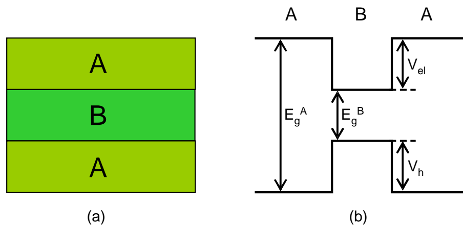
Figura 10: Poço quântico formado pela justaposição de várias camadas semicondutoras.
