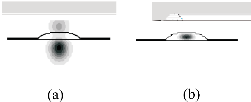
Figura 60: Funções de onda do (a) elétron e (b) buraco numa estrutura elipsoidal tipo-II sobre o potencial do ponto.
