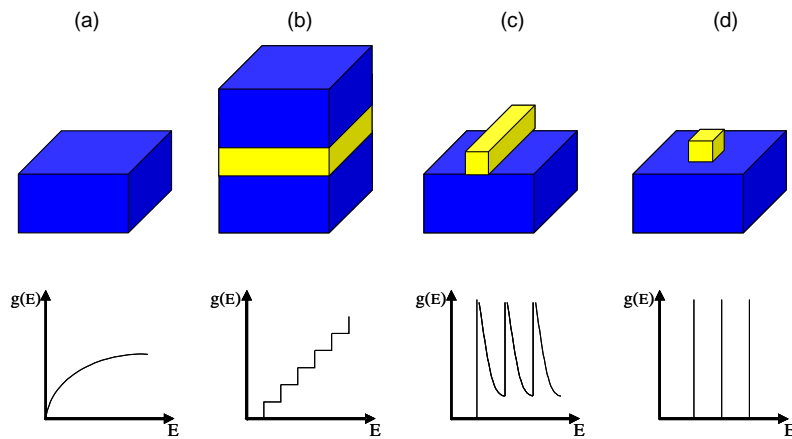
Figura 8: Confinamento das hetero-estruturas em relação a dimensionalidade, de um material bulk-3D (a) até o ponto quântico-0D (d), passando por um poço-1D (b) e um fio quântico-2D (c) e seus respectivos densidades de estados.
