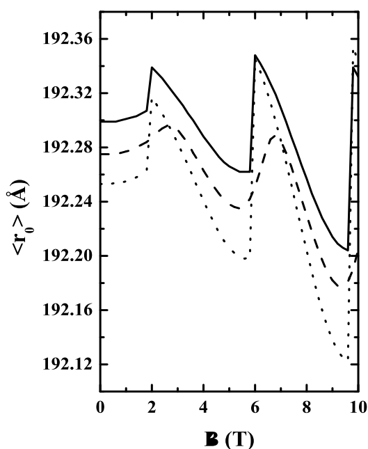
Figura 37: Raio médio do estado fundamental com duas impurezas hidrogênicas negativas no anel quântico com tamanho a = 140 \text{ \AA} e b = 240 \text{ \AA} com a primeira impureza fixa em \vec{r}_{imp}^{(1)} = (190 \text{ \AA}, 0, z_i) e a segunda em \vec{r}_{imp}^{(2)} = (-190 \text{ \AA}, 0, z_i) , em duas diferentes posições no plano do anel, z_1 = 10 \text{ \AA} (linha sólida) e z_2 = 30 \text{ \AA} (linha tracejada), e para a primeira impureza fixa em \vec{r}_{imp}^{(1)} = (190 \text{ \AA}, 0, 30 \text{ \AA}) e a segunda em \vec{r}_{imp}^{(2)} = (190 \text{ \AA}, 0, 30 \text{ \AA}) (linha pontilhada).
