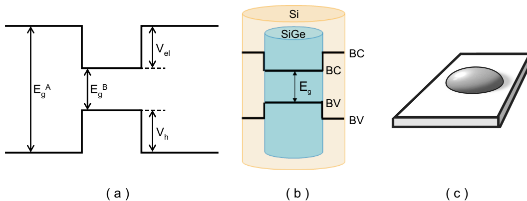
Figura 9: Representação esquemática de uma heterojunção entre dois semicondutores diferentes: (a) formando um potencial de confinamento num poço, (b) num fio quântico e (c) um ponto quântico.
