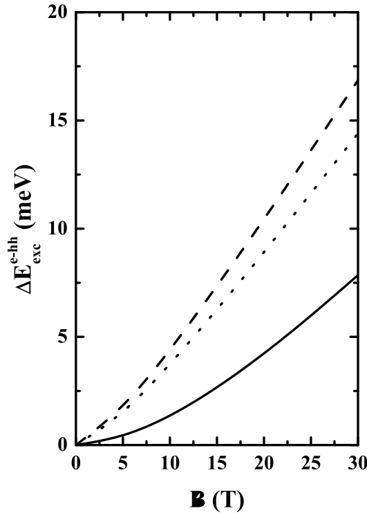
Figura 27: Shift da energia total do exciton em função do campo magnético B , para poços quânticos abruptos de 70 \text{ \AA} de largura Si/Si_{0.82}Ge_{0.18} tipo-I (sólido) e Si/Si_{0.70}Ge_{0.30} tipo-II usando as aproximações 2D (linha pontilhada) e 3D (linha tracejada).
