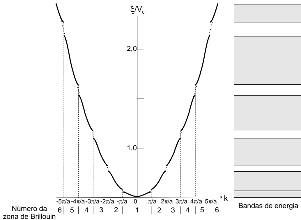
Figura 3: Energias permitidas em função do vetor \kappa , para uma rede unidimensional de periodicidade a . A linha tracejada é a energia para o caso de um elétron livre. As bandas de energia permitidas e proibidas resultantes aparecem à direita.
