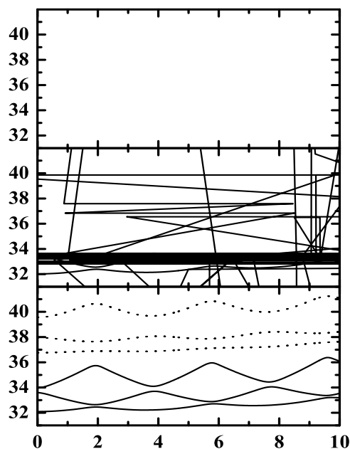
Figura 43: (a) Espectro de energia do elétron e (b) transições das energias do estado fundamental (sólida) para o primeiro (tracejada), segundo (pontilhada) e terceiro (tracejada-pontilhada) estados excitados, em função do campo magnético para um anel ideal, considerando R_I = 140 \text{ \AA} e R_E = 240 \text{ \AA} .
