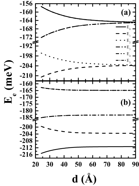
Figura 68: Espectro de energia do elétron em função da distância entre os pontos quânticos para o caso de acoplamento vertical, considerando R_1 = 120 \text{ \AA} e R_2 = 120 \text{ \AA} (a) e 150 \text{ \AA} (b).
