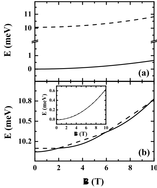
Figura 34: Energia do estado fundamental (linha sólida) e primeiro estado excitado (linha tracejada), para duas impurezas hidrogênicas positivas próximo ao anel quântico de tamanho a = 140 \text{ \AA} e b = 240 \text{ \AA} com a primeira impureza localizada em \vec{r}_{imp}^{(1)} = (190 \text{ \AA}, 0, z_1) e a segunda em \vec{r}_{imp}^{(2)} = (-190 \text{ \AA}, 0, z_2) . Em (a) z_1 = 10 \text{ \AA} e z_2 = 30 \text{ \AA} , (b) z_1 = z_2 = 30 \text{ \AA} ( z_1 = z_2 = 10 \text{ \AA} no inset ).
