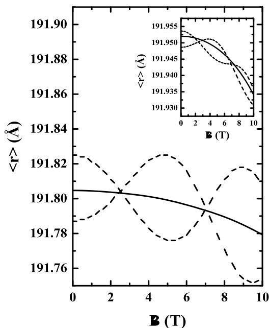
Figura 35: Raio médio do estado fundamental e primeiro estado excitado, para o mesmo anel e parâmetros usado na Fig.34. A linha tracejada corresponde a z_1 = z_2 = 30 \text{ \AA} ( z_1 = z_2 = 10 \text{ \AA} no insete), e a linha sólida para z_1 = 10 \text{ \AA} e z_2 = 30 \text{ \AA} o estado fundamental (estado excitado no inset ), respectivamente.
