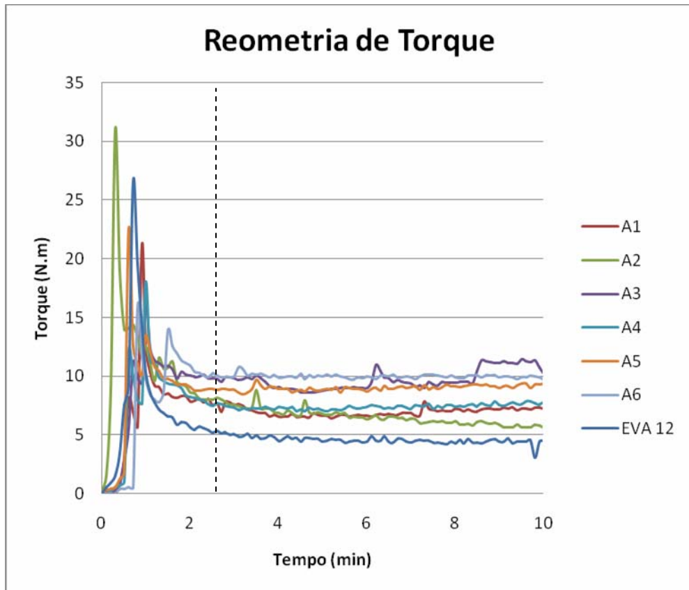
Figura 27. Reometria das composições propostas.
