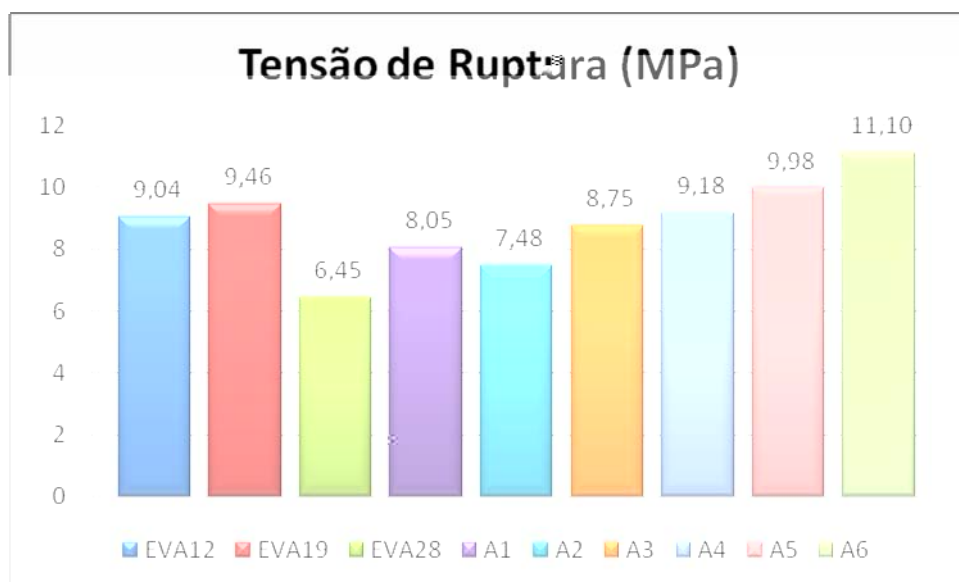
Figura 34. Tensão de ruptura (MPa).
