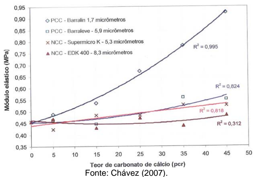
Figura 12. Módulo elástico da espuma de EVA em função do teor de CaCO 3 .
