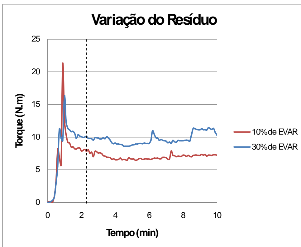
Figura 28. Reometria do aumento no teor de resíduo.
