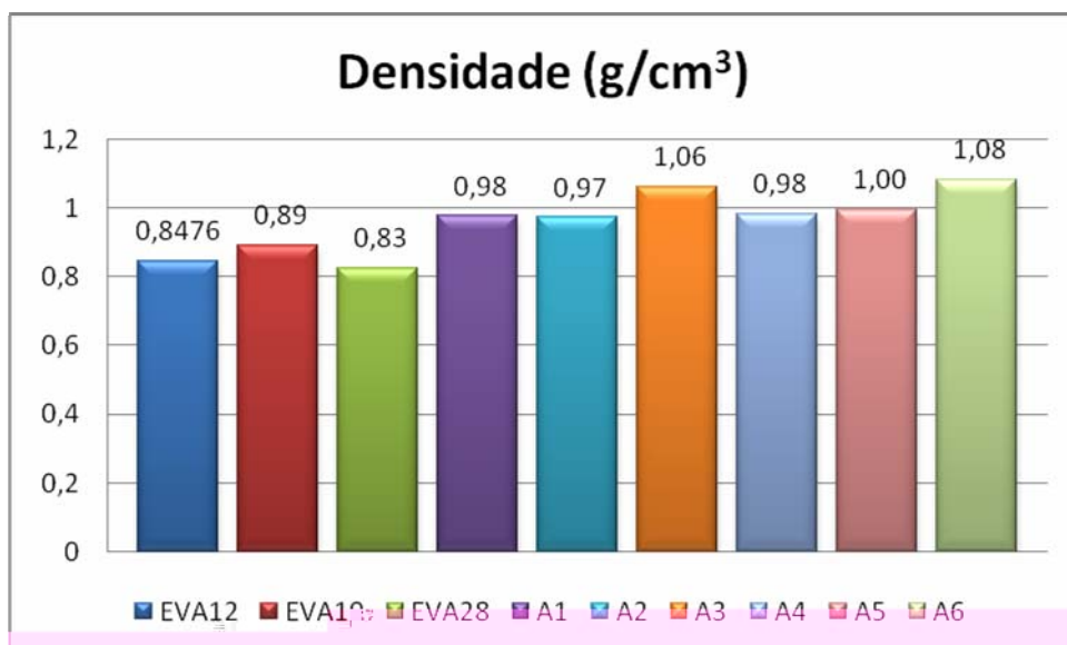
Figura 35. Densidade.
