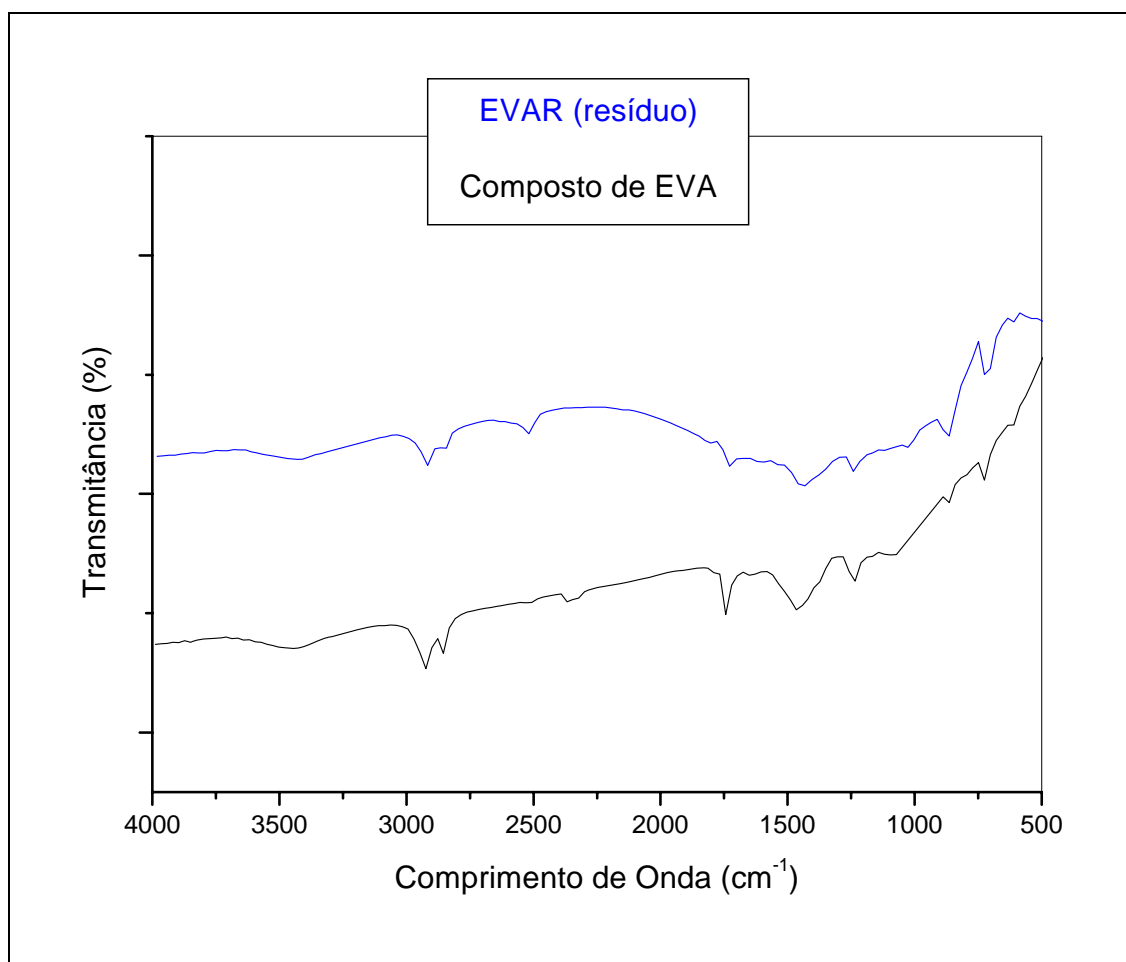
Figura 31. FTIR do resíduo e do material reciclado.
