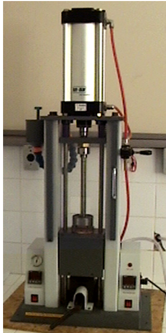
Figura 19. Injetora Ray Ran.
