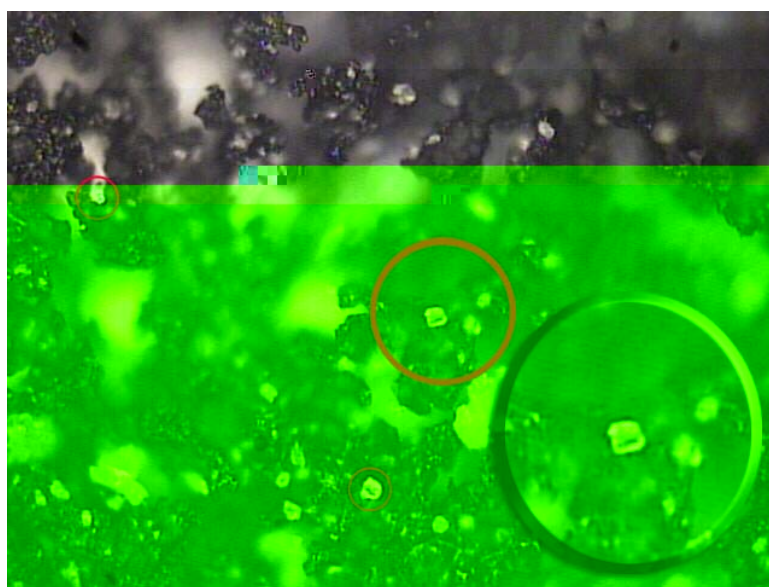
Figura 24. Microscopia Ótica da Amostra do Composto de EVAR preto passante na malha 100 (Aumento 100x).
