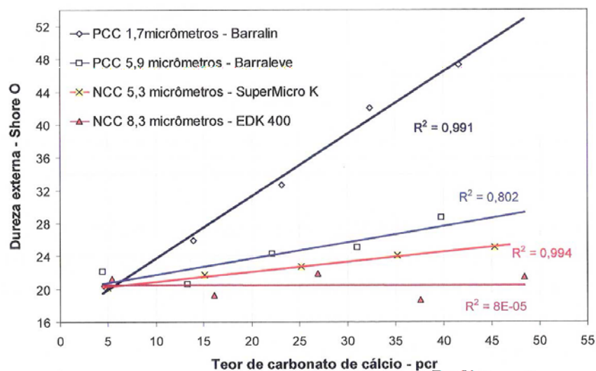
Figura 11. Dureza da Espuma de EVA em função do Teor de \text{CaCO}_3 .
