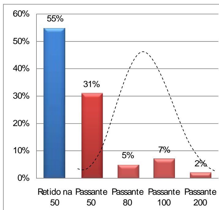
Figura 23. Granulometria do resíduo em porcentagem. Vermelho é a porcentagem granulométrica utilizada na pesquisa.
