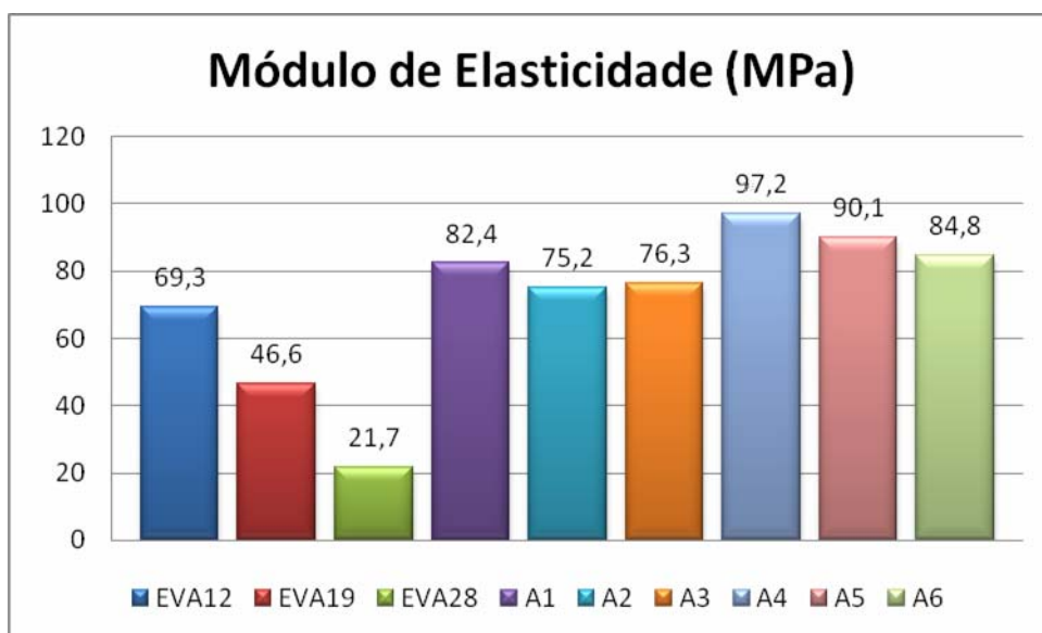
Figura 33. Módulo elástico.
