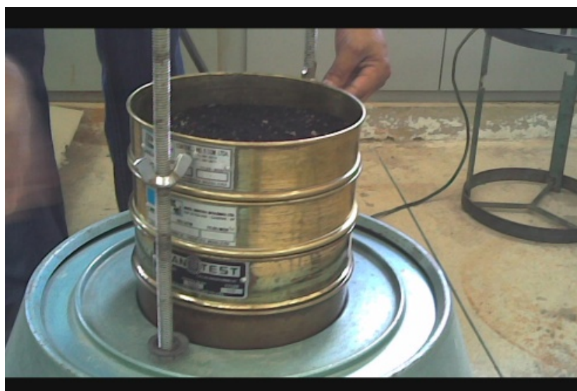
Figura 16. Classificação Granulométrica do Resíduo.
