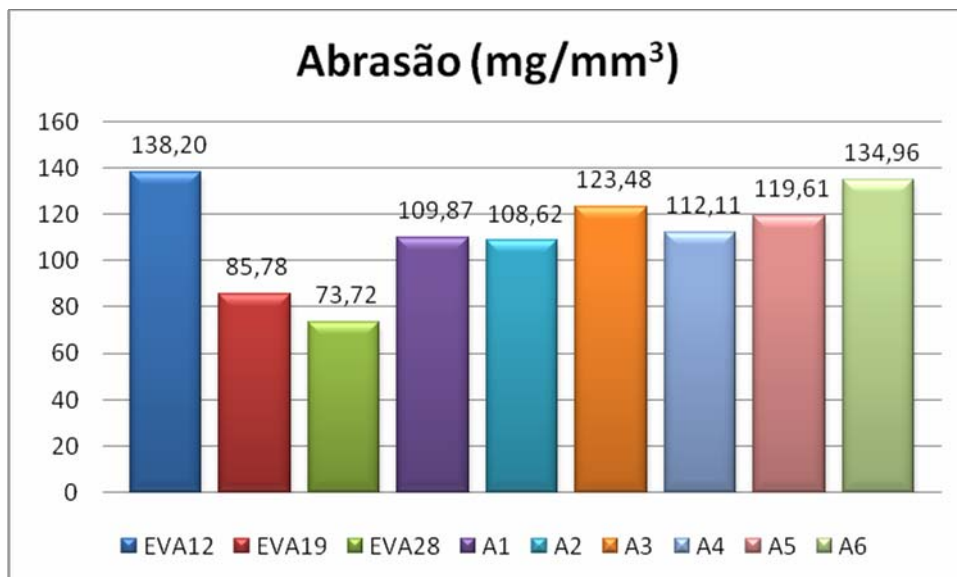
Figura 37. Resistência a Abrasão.
