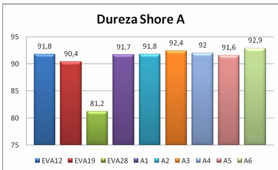
Figura 36. Dureza.
