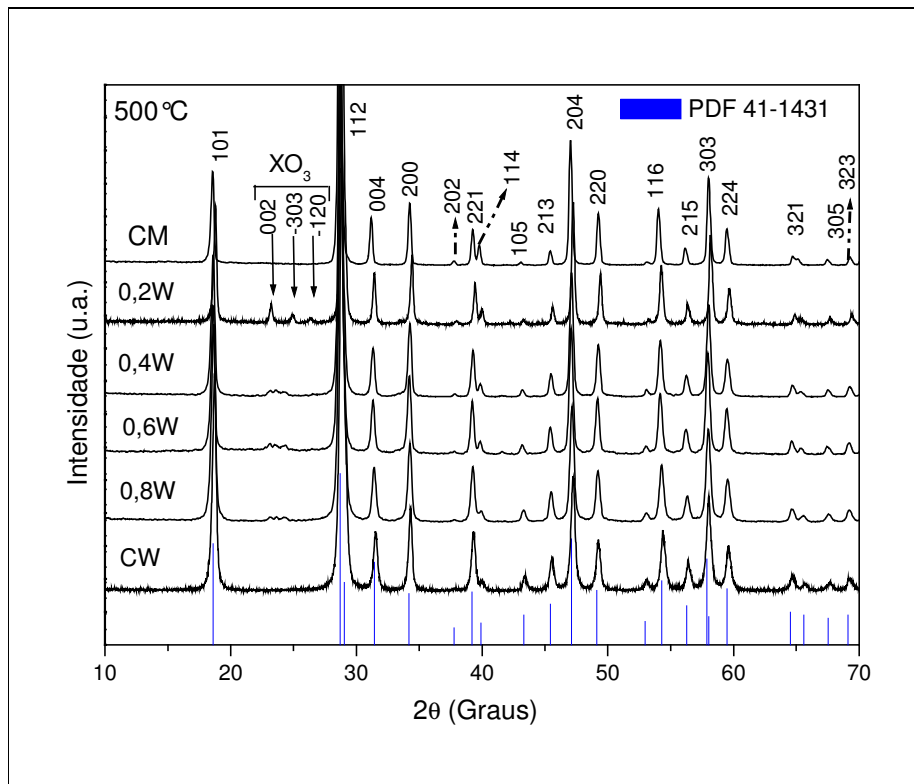
Figura 17: Difratoigramas de raio X dos pós do CM, CMW E CW tratados a 500°C, comparados a ficha JCPDS n° 41-1431.
