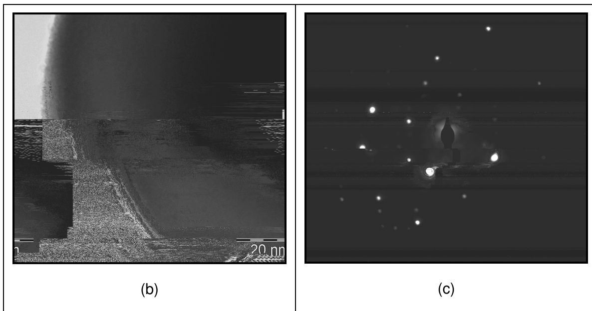
Figura 64: Micrografias obtidas por MET dos pós da mistura 0,8W tratados a 700^{\circ}\text{C} (a), superfície da partícula (b) e padrão de difração de elétrons (c).
