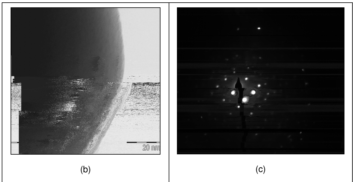
Figura 60: Micrografias obtidas por MET dos pós do CaMoO 4 (CM) tratados a 700 °C (a), superfície da partícula (b) e padrão de difração de elétrons (c)
