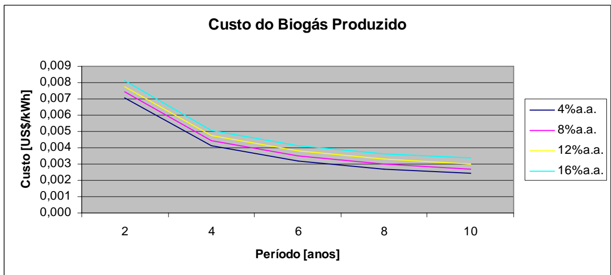
Figura 34 – Custos do biogás produzido pela mini-ETE
