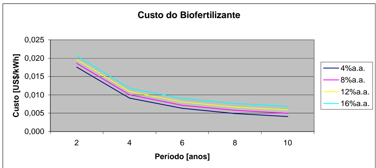
Figura 22 – Custos do biofertilizante produzido pelo sistema BGFM
