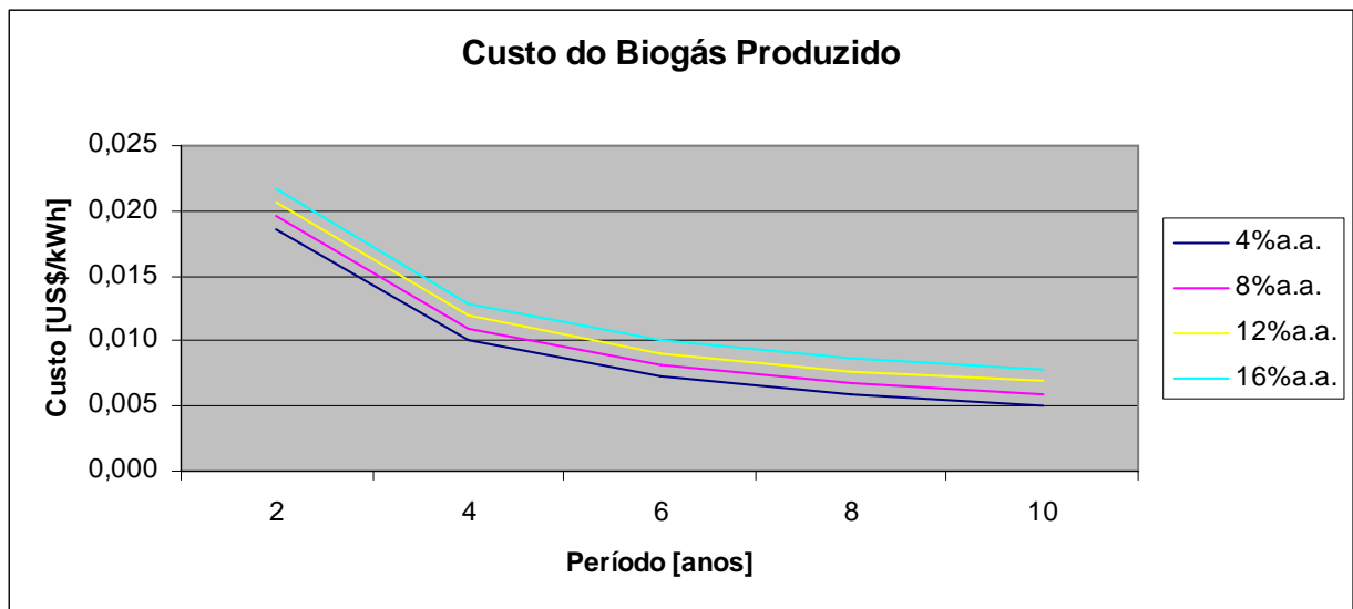
Figura 23 – Custos do biogás produzido pelo sistema BGFM
