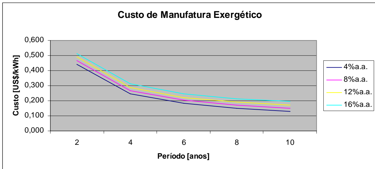
Figura 25 – Custo de manufatura exergético do sistema BGFM
