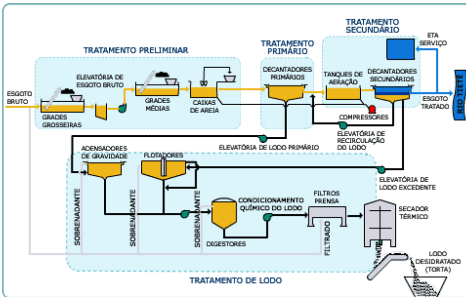
Figura 6 – Etapas do tratamento de esgoto
