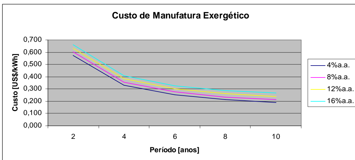
Figura 36 – Custo de manufatura exergético da mini-ETE
