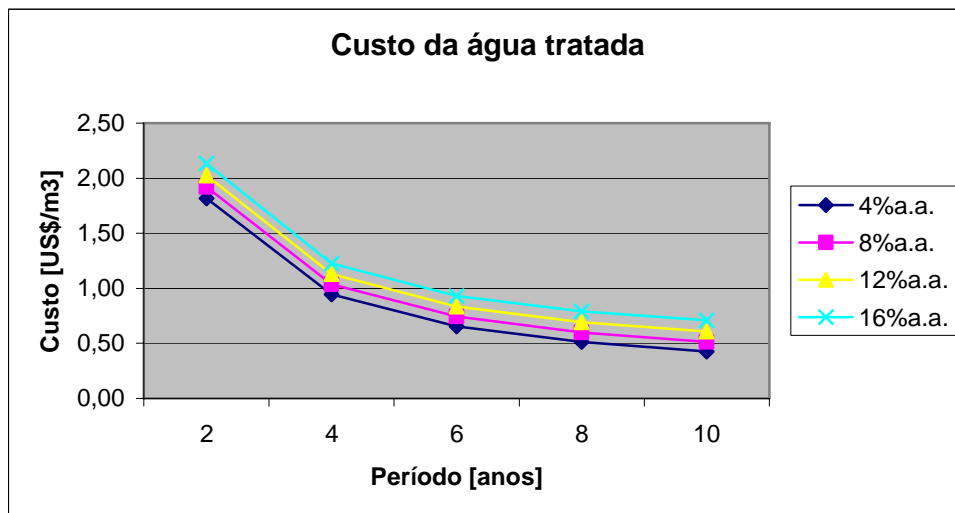
Figura 49 – Custo água tratada para o sistema disponível no mercado nas diversas condições de análise
