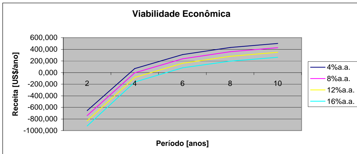
Figura 26 – Receita anual do sistema BGM para os períodos observados
