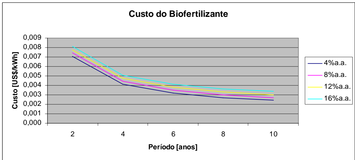
Figura 33 – Custos do biofertilizante produzido pela mini-ETE
