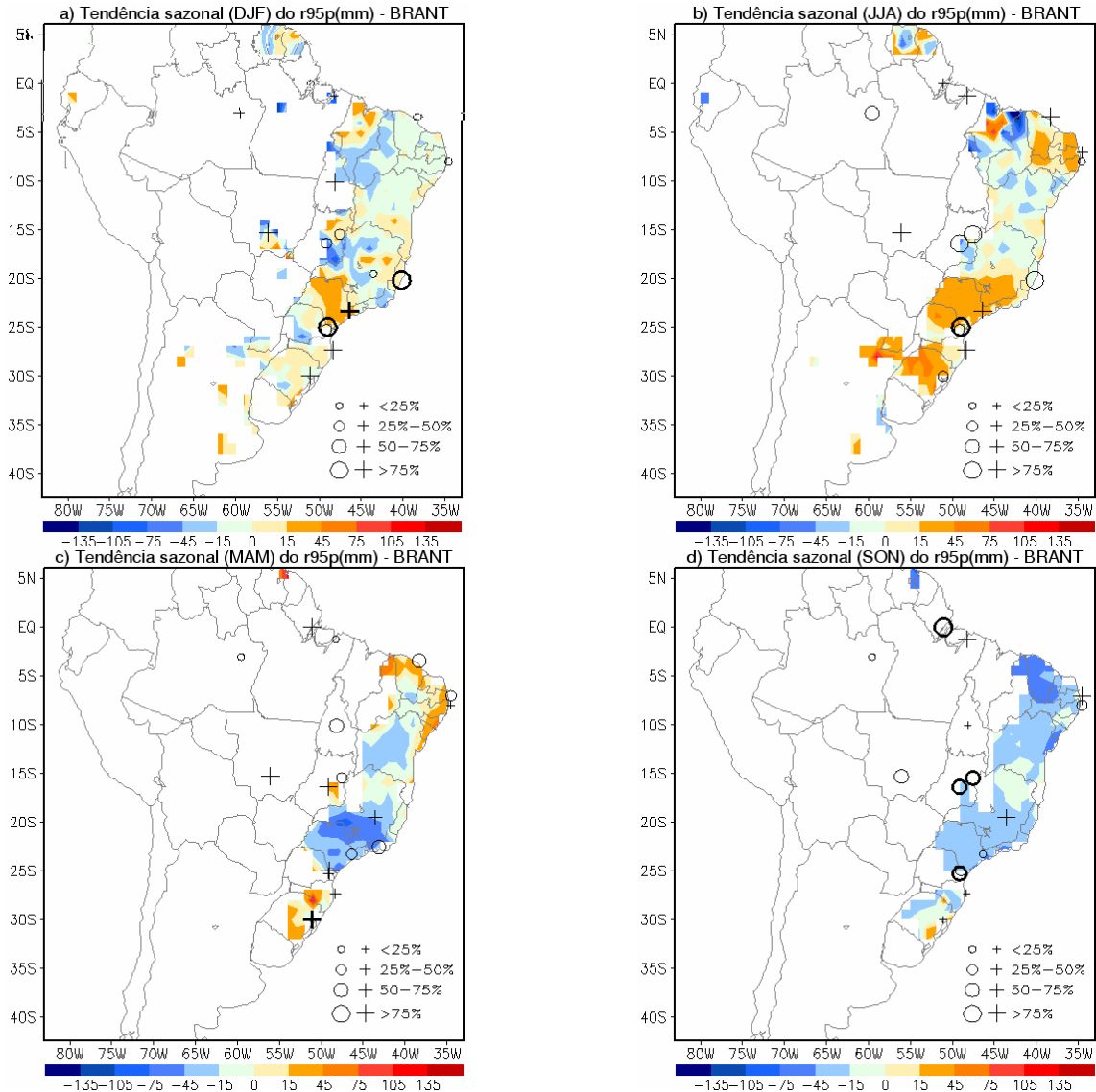
Fig. 7B. Tendência do índice sazonal r95p (mm) sobre a América do Sul durante o período de 1961-1990 obtida a partir da análise de BRANT: (a) verão (DJF), (b) inverno (JJA), (c) outono (MAM) e (d) primavera (SON). O intervalo e a escala de intensidade são mostrados no rodapé da figura.
