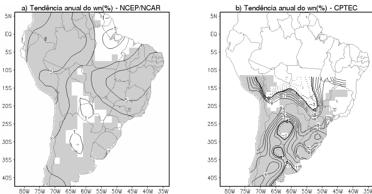
Fig. 4.5. Tendência do índice anual wn (%) durante o período de 1961-1990 obtida a partir da (a) reanálise do NCEP/NCAR, (b) análise do CPTEC (1959-2000) sobre a América do Sul, (c) estações de superfície no Brasil e (d) no Estado de São Paulo. (a-b) O sombreado destaca as regiões com tendência significativa no nível de 5%. O contorno zero está em negrito, os positivos contínuos e os negativos pontilhados. (c-d) A tendência positiva é representada por '+' e a negativa por 'o', sendo os seus tamanhos proporcionais à magnitude da tendência, conforme escala indicada nos mapas. Os símbolos em negrito indicam tendência estatisticamente significativa no nível de 5%.
