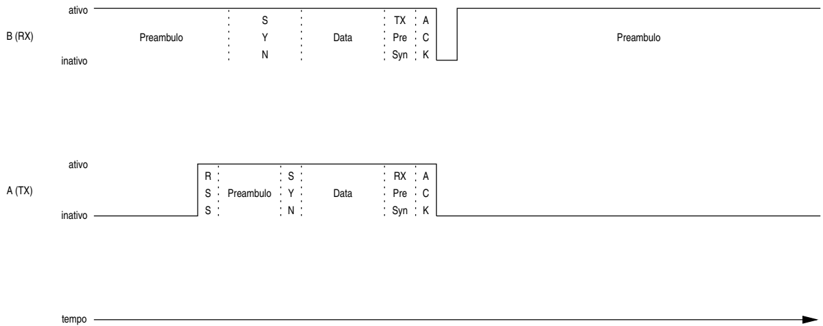
Figura 4.5: Comunicação bem sucedida no C-MAC/CSMA Simplex
