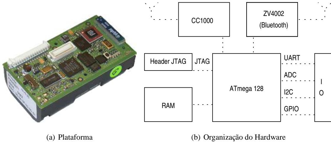
Figura 2.12: BTnode
