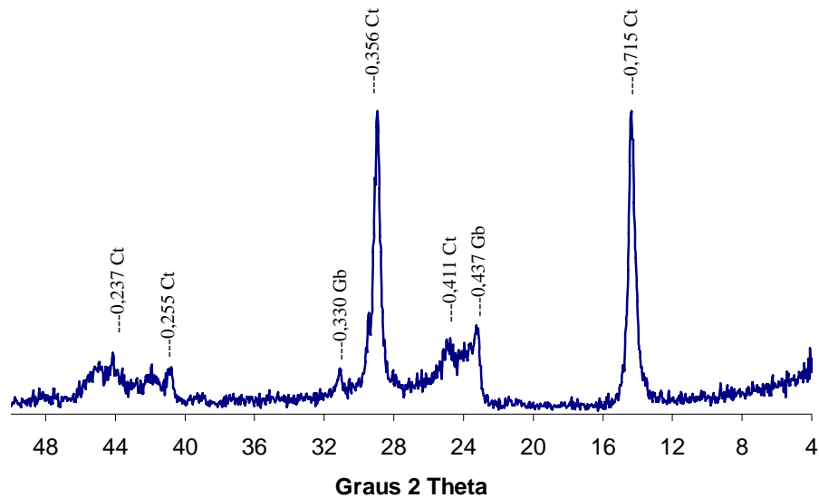
Anexo C. Difratograma de raios X da fração argila (montagem orientada) de amostra de Latossolo (Berilo-MG) contendo Ct: caulinita; Gb: gibbsita. Números representam espaçamento d em nm. CoK /Ni.
