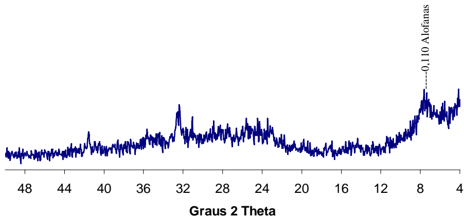
Anexo B. Difratoograma de raios X da fração argila (montagem orientada) de amostra de Criosolo (Antártica) contendo Alofanas e aluminosilicatos amorfos. Números representam espaçamento d em nm. CoK /Ni.
