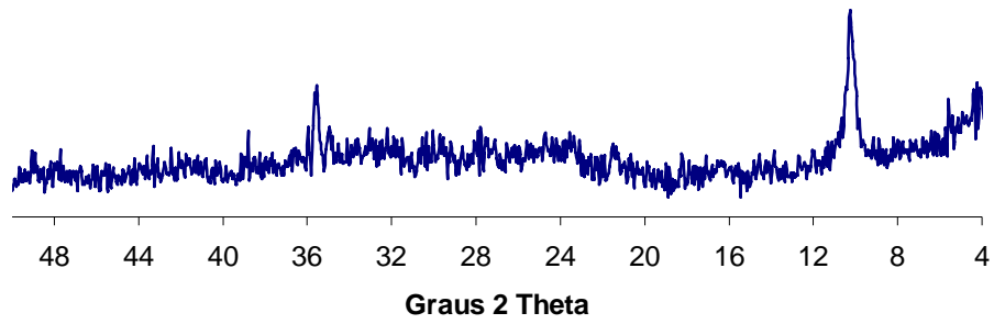
Anexo G. Difratoograma de raios X da fração argila (montagem orientada) de amostra de Organosolo (Ilha de Trindade) contendo Gb: gibbsita; Gt: goethita; Bt: biotita. Números representam espaçamento d em nm. CoK /Ni.
