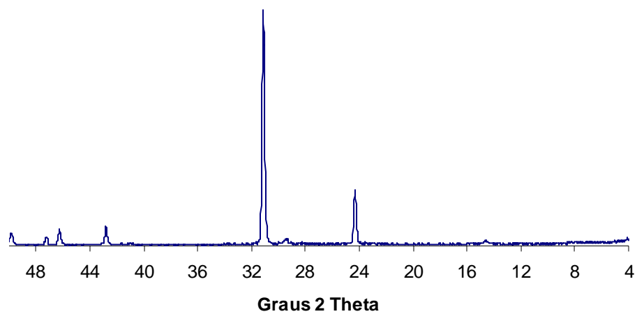
Figura 2. Difratoograma de raios X (montagem em pó) de amostra de madeira petrificada antes do ataque ácido, contendo Qz: quartzo, Gt: Goethita, Hm: Hematita. Números representam espaçamento d em nm. CoK /Ni.
