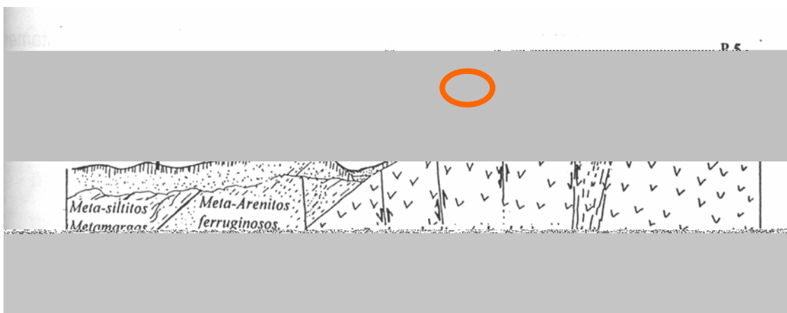
Figura 5. Perfil geológico esquemático da topolitossequência e posição do solo, simbolicamente representado nesta figura como P7. (Fonte: Rolim Neto, 2002).
