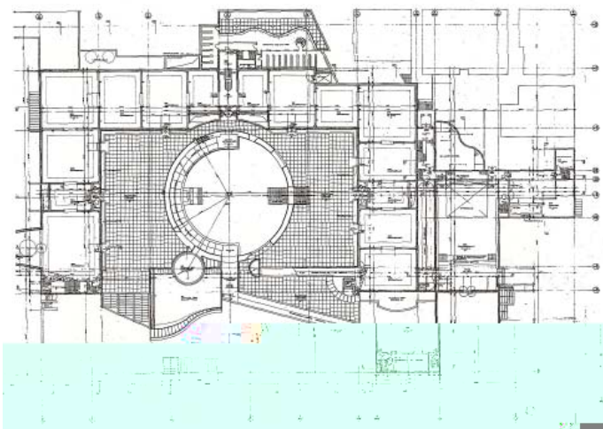
Fig.35 – Planta baixa: Museu Staasgalerie, 1977-1983.
