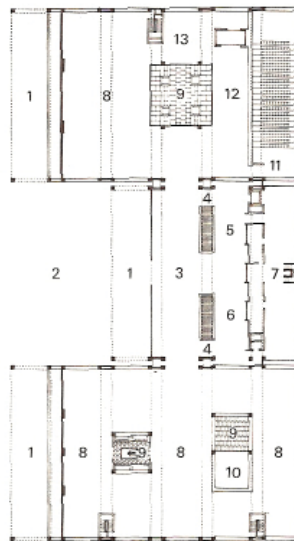
Fig. 30 – Planta Baixa: Museu de Belas Artes de Kimbell, 1967-1972. Detalhe para as galerias (nº8) integradas e da presença de espaços como lanchonete (nº12), auditório (nº11) e loja de livros(nº5).
