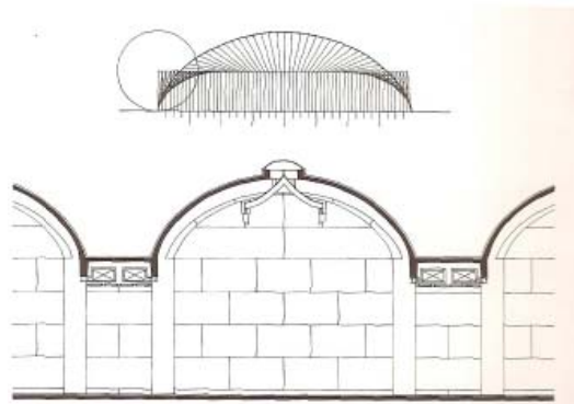
Fig. 29 – Corte abóbodas: Museu de Belas Artes de Kimbell, 1967-1972.
