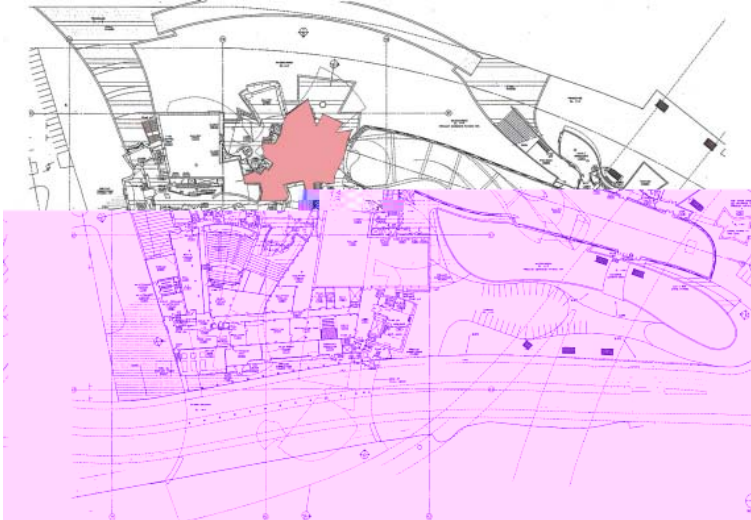
Fig. 43 – Planta 1º piso: Museu Guggenheim de Bilbao, 1997. Átrio em destaque na planta.
