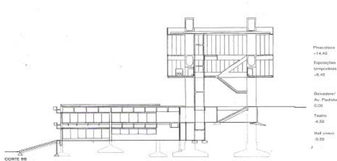
Figura 23 – Corte do MASP mostrando o Trianon e o Museu.
