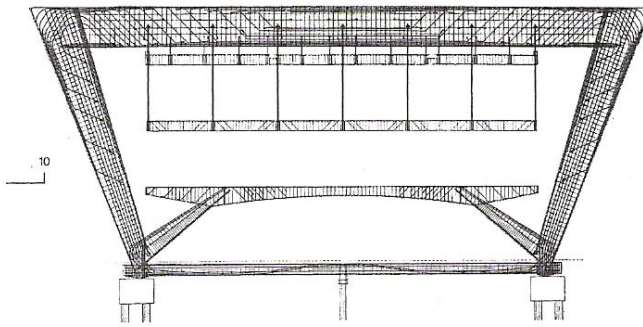
Figura 19 – Esquema estrutural do MAM.
