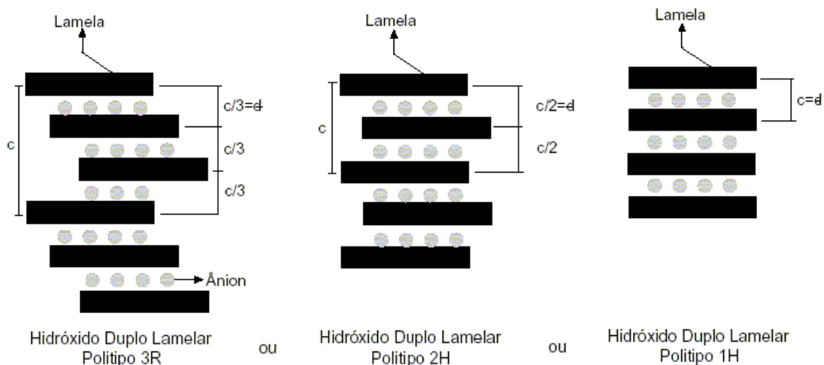
Figura 2: Esquema representando os possíveis politipos para os hidróxidos duplos lamelares 9 .
