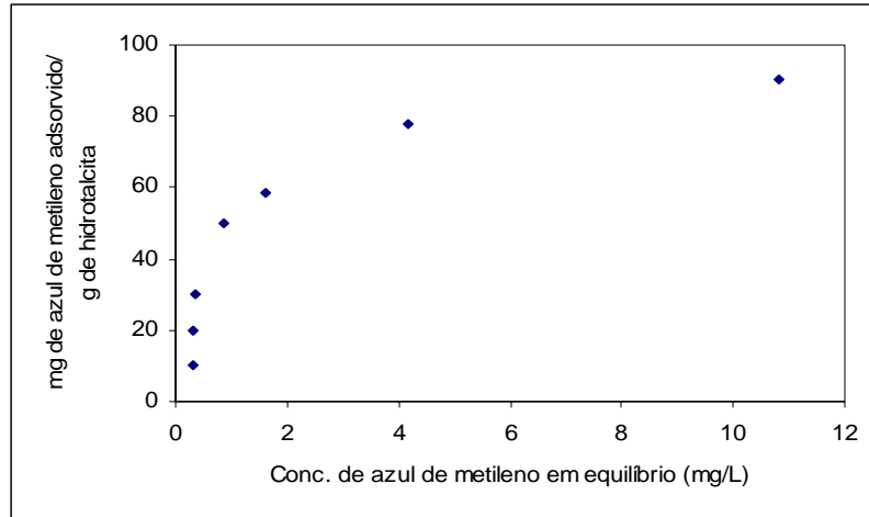
Figura 45: Isoterma de adsorção do azul de metileno em hidrotalcita.
