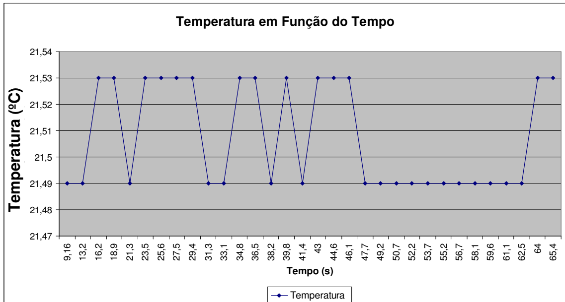
Figura 58 – Demonstração da temperatura em função do tempo.
