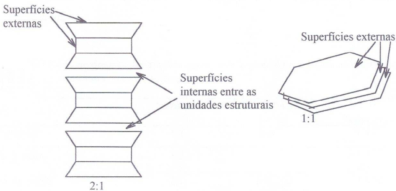
Figura 10. Esquemática das superfícies de exposição interna e externa dos argilominerais secundários 62 .
