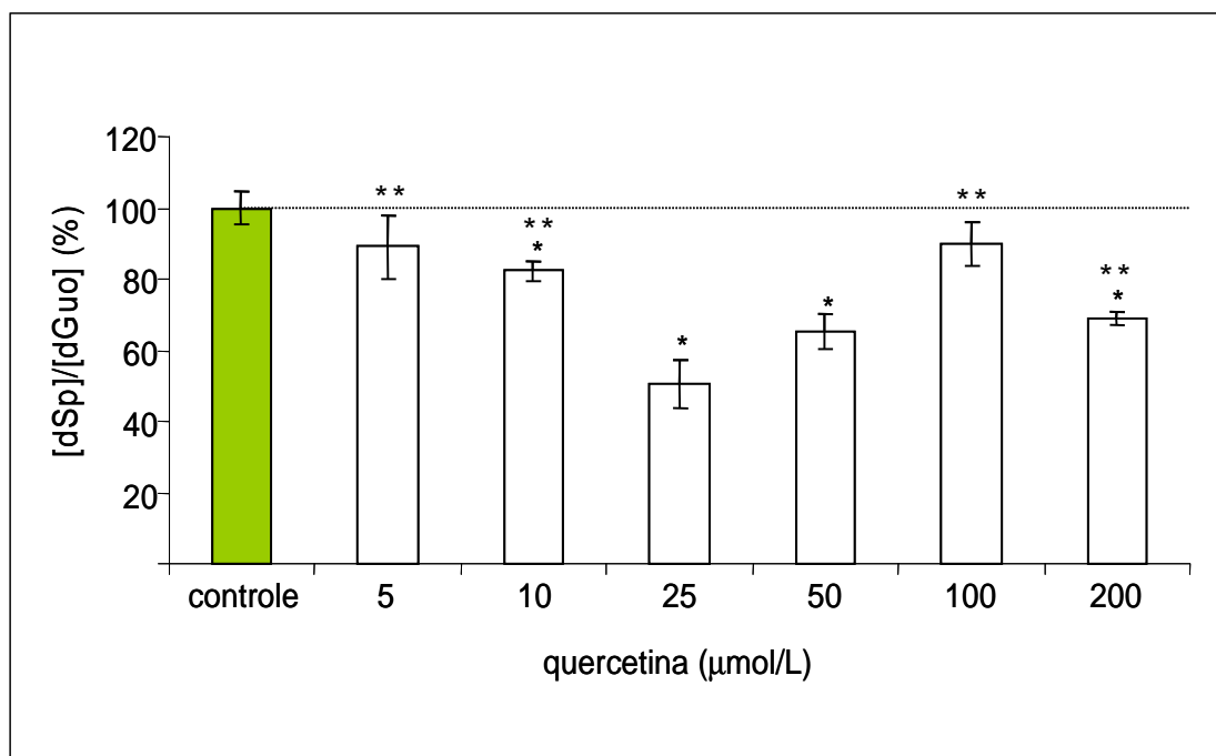
FIGURA 21 – DETECÇÃO DA dSP, NA INCUBAÇÃO DA dGUO COM DIFERENTES CONCENTRAÇÕES DE QUERCETINA
