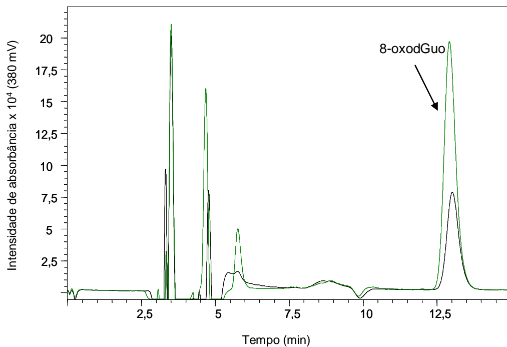
FIGURA 14 – CROMATOGRAMA REPRESENTATIVO DA DETECÇÃO DA 8-oxodGUO
