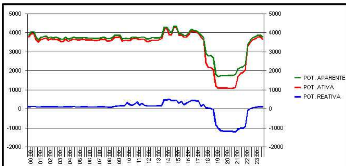
Gráfico 3.1. Curva de Carga Típica.
