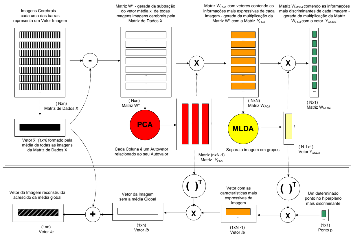
Figura 3.5 – Diagrama da Análise Multivariada PCA + MLDA (Adaptado de THOMAZ et. al., 2006) [58].
