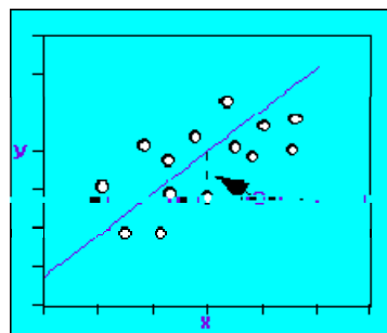
Figura 3.3. O modelo linear de duas variáveis: y = b_0 + b_1x + e (Adaptado de Trochim, W. - 2000).
