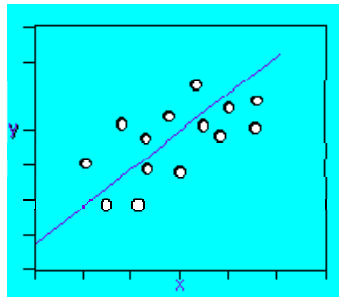
Figura 3.2. Uma linha reta resumindo os dados das duas variáveis (Adaptado de Trochim, W. - 2000).
