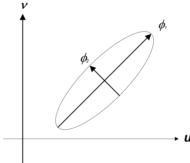
Figura 3.4 – Análise de componentes principais com os autovetores \phi_1 e \phi_2 .
