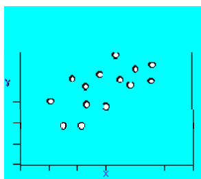
Figura 3.1 – Gráfico com duas variáveis (Adaptado de Trochim, W. - 2000).
