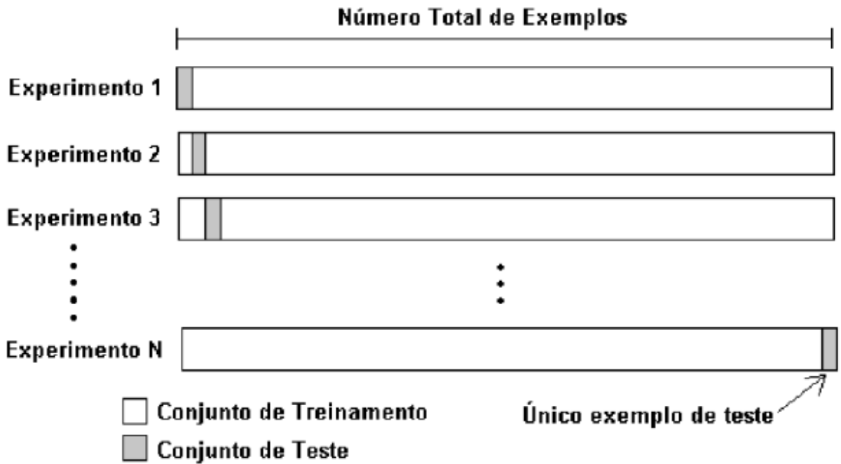
Figura 5.23 – Exemplo do método de validação cruzada Leave-one-out aplicado a um conjunto de N exemplos.
