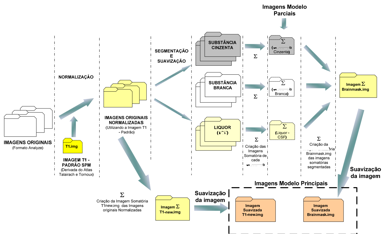
Figura 4.7 – Fluxograma descrevendo as etapas da fase de criação de imagens modelos para o pré-processamento.
