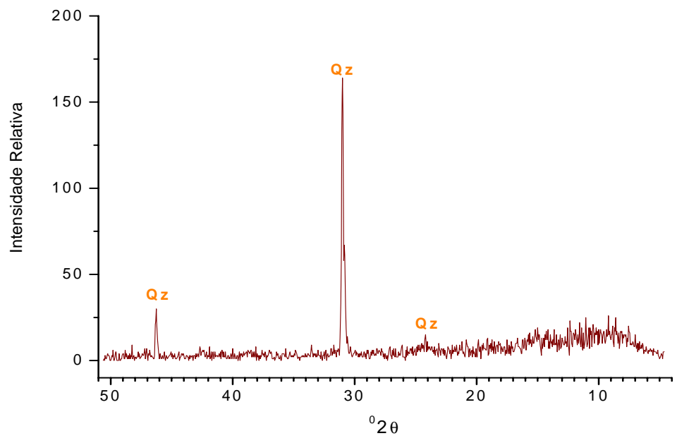
Figura 3 – Difratoograma da fração areia da amostra de solo.
