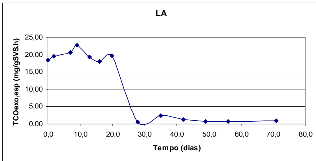
FIGURA 4.8: Variação da TCO exo,esp do lodo gerado no sistema LA, num teste de sobrevivência.
