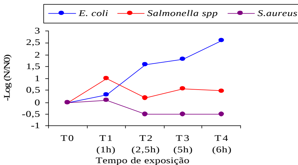
Figura 5.13 – Eficiência da desinfecção com radiação UV de lâmpadas fluorescentes germicidas 15W (NARDS) na inativação das populações de Salmonella spp., E. coli e S. aureus (ATCC 25923) (CG/PB -11/05/2006)
