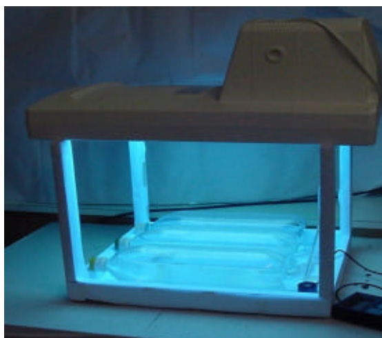
Figura 4.13 – Garrafas expostas à radiação UV de lâmpadas solares 20W (PHILIPS Clio) no Laboratório de Química Biológica do Instituto de Química da UNICAMP (Campinas/SP – 20/08/06)
