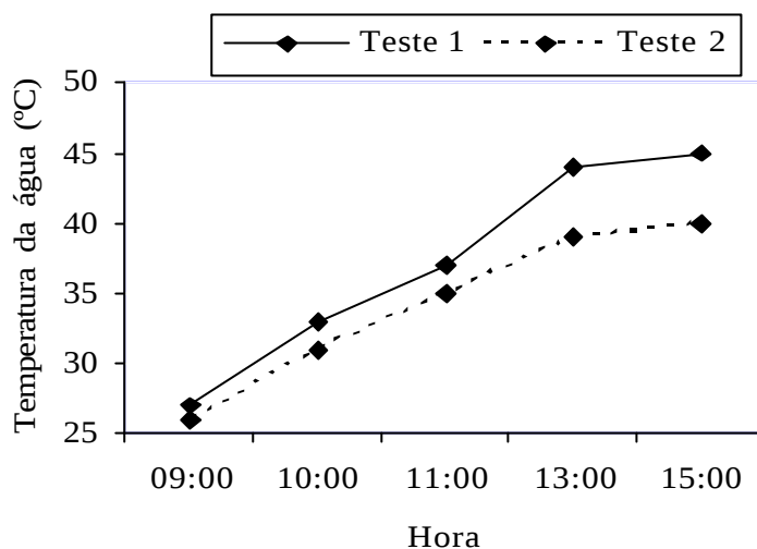
Figura 5.4 – Variação da temperatura nas amostras de água expostas ao sol e inoculadas com E. coli (ATCC25922) (Testes 1 e 2) nas garrafas controle durante 6 horas de exposição à radiação solar (CG/PB – 08 e 12/11/06)
