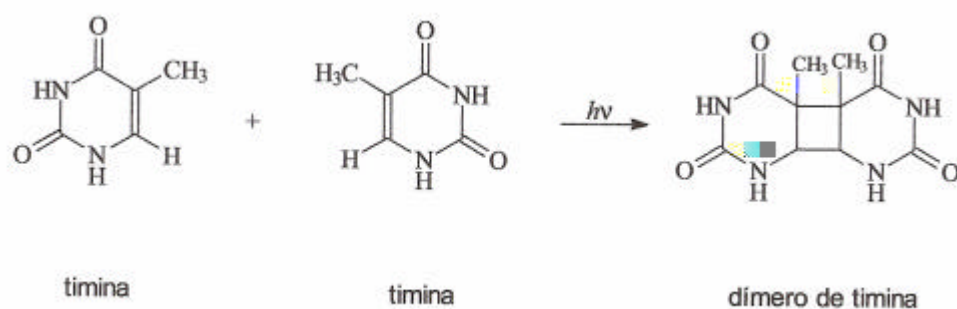
Figura 3.2 – Dimerização fotoquímica de duas bases nitrogenadas
