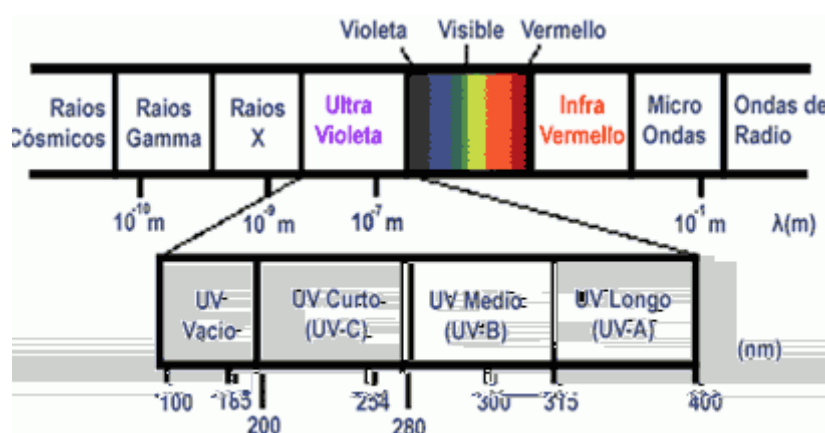
Figura 3.1 – Espectro eletromagnético
