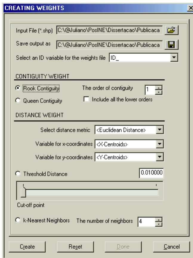
Figura 3.8 - Janela de criação da matriz de dependência espacial
