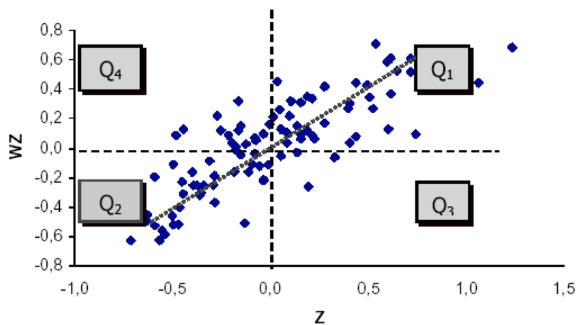
Figura 3.10 - Gráfico de espalhamento de Moran Fonte: Câmara et al. (2000)
