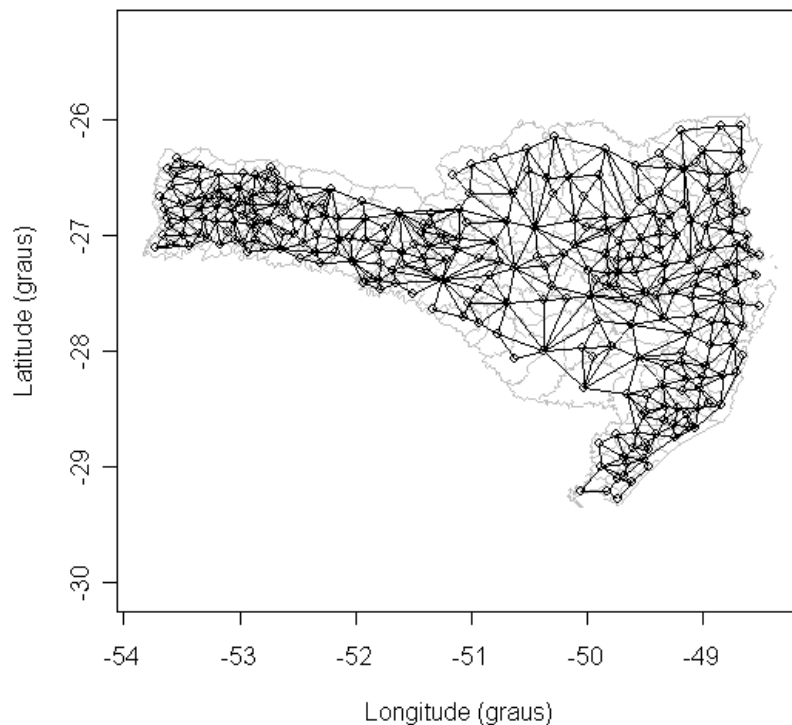
Figura 4.3 - Representação gráfica da estrutura de dependência espacial
