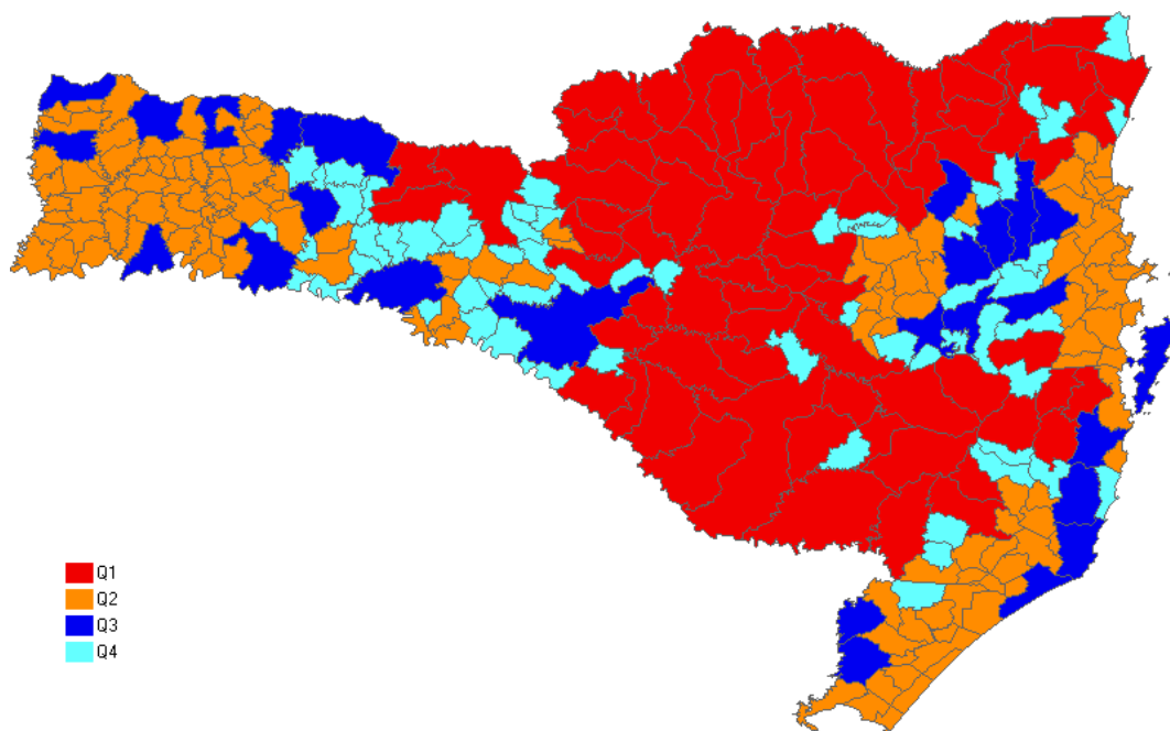
Figura 3.13 - Box Map para a variável área
