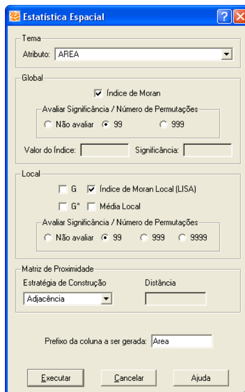
Figura 3.9 - Janela de cálculo das estatísticas espaciais no programa TerraView
