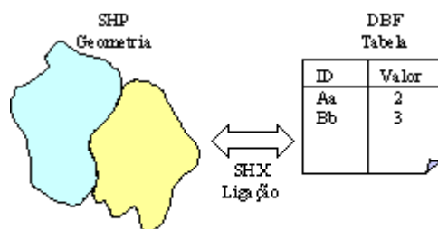
Figura 2.8 - Estrutura do formato Shape da ESRI
