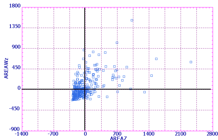
Figura 3.11 - Gráfico de espalhamento de Moran para a variável área
