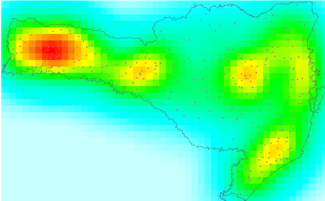
Figura 3.21 - Superfície estimada com base na distribuição das sedes dos municípios catarinenses
