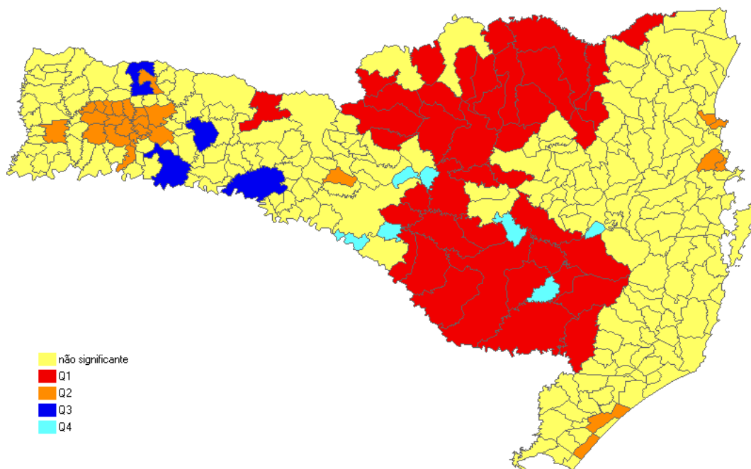
Figura 3.17 - Moran Map para a variável área
