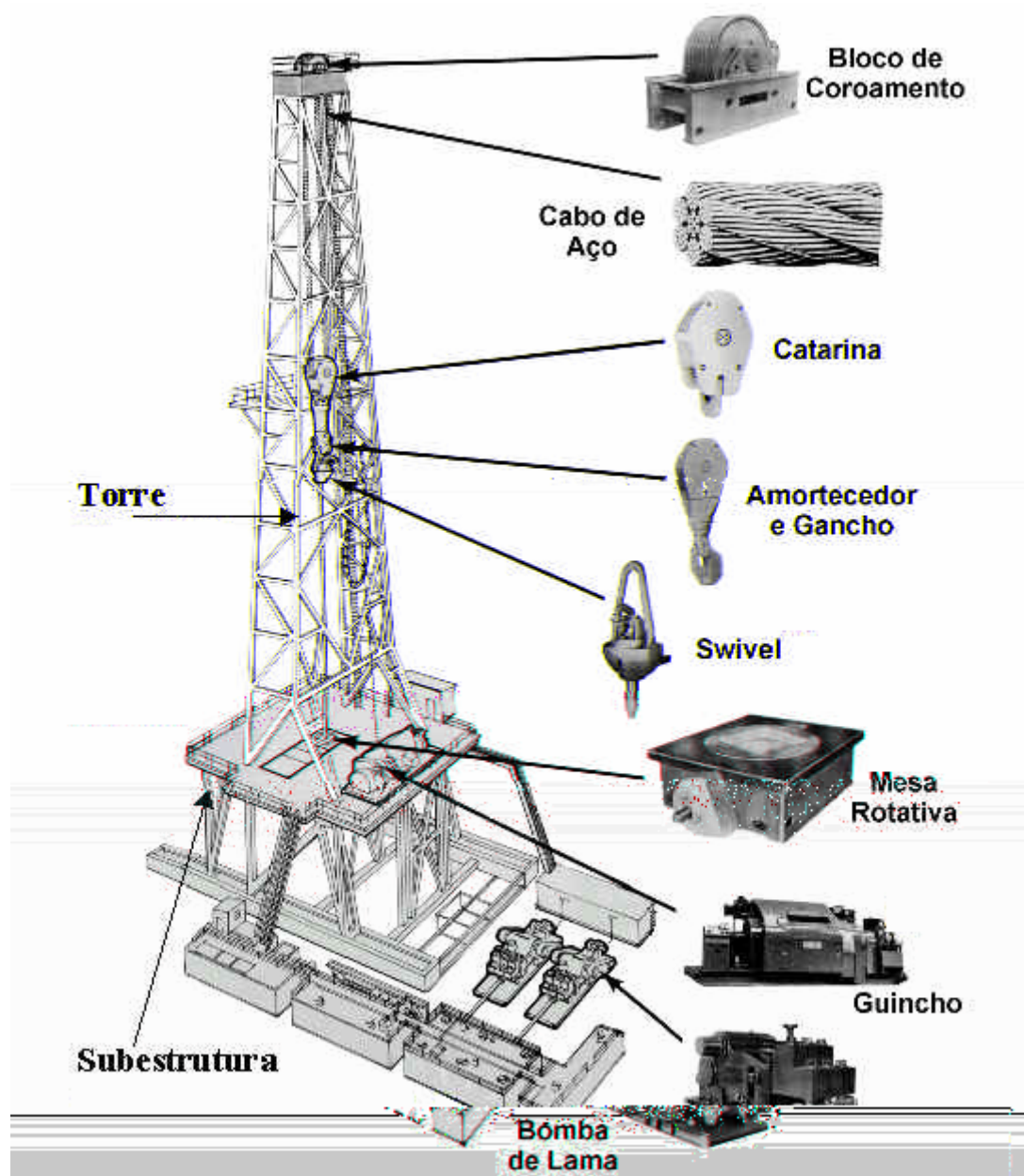
FIGURA 3.1 – Sonda (Extraído de DOMINGOS, Luís. Perfuração no mar . Disponível em: < http://histpetroleo.no.sapo.pt/perf_mar.htm >. acesso em: 1 mar. 2004).
