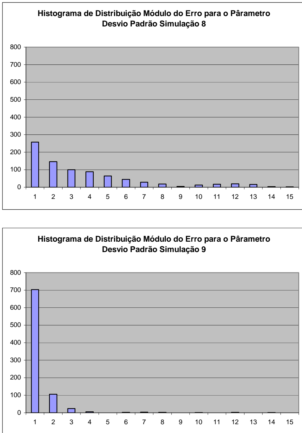
FIGURA 5.7 – Histogramas de distribuição do erro nas simulações 8 e 9. O no eixo x estão valores de tempo/10, ou seja cada unidade representa 10 horas, e em y a freqüência com que tal erro ocorre nos dados utilizados para teste e validação.
