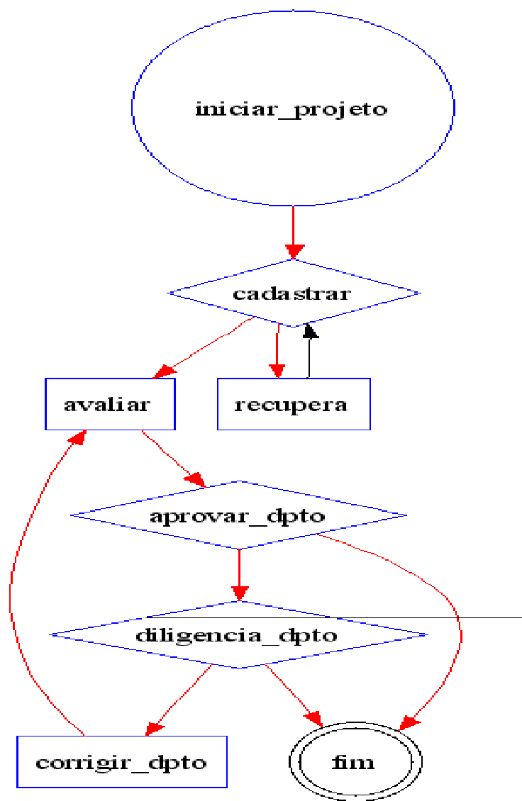
Figura 11 – Workflow - Projeto de Pesquisa
