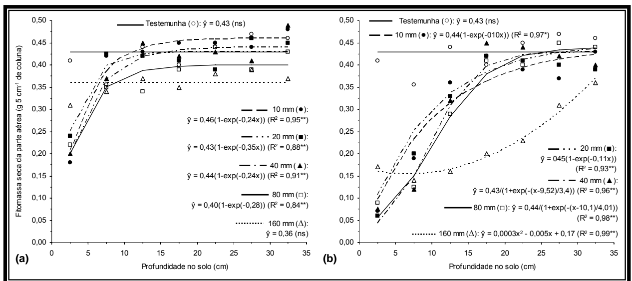
FIGURA 2: Fitomassa seca de Sorghum bicolor coletado a cada 5cm ao longo das colunas de solo que receberam ametryn (a) e a mistura de clomazone+hexazinone (b), em razão de percolação de 10, 20, 40, 80 e 160 mm, mais o tratamento testemunha (ausência de herbicida). * e ** significativos a 5% e 1% de probabilidade, respectivamente. ns: não significativo.
