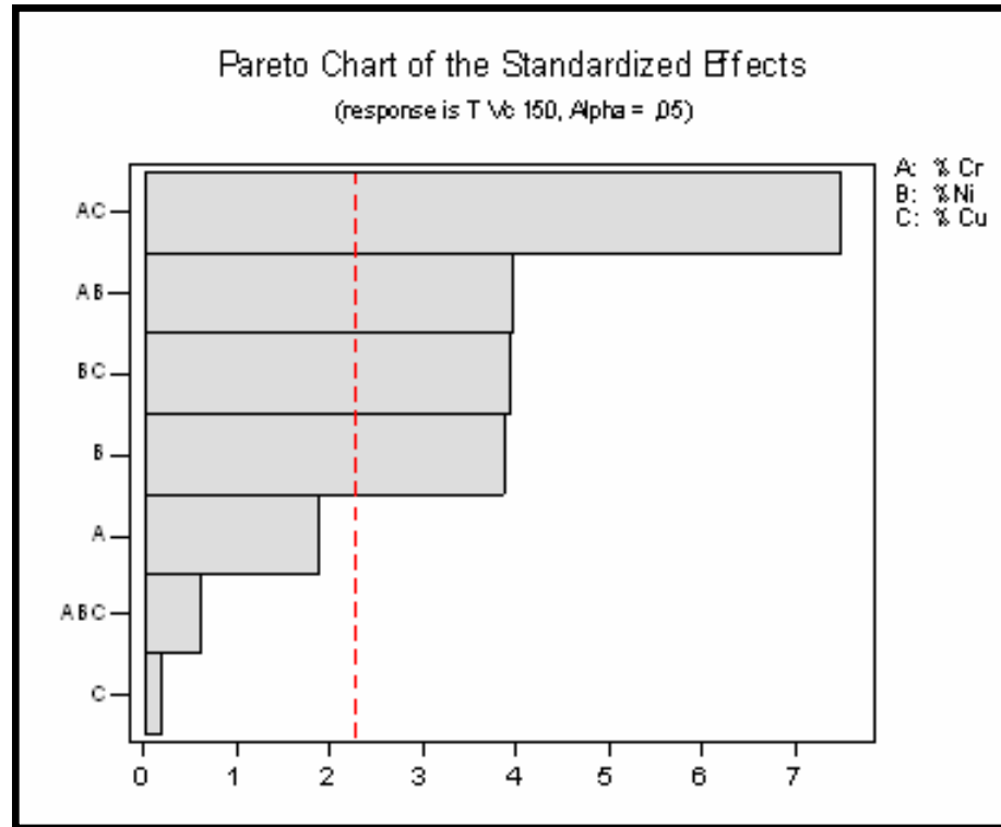
Figura 7.2 – Diagrama de Pareto: efeitos dos elementos e suas interações – Vc 150 m/min.
