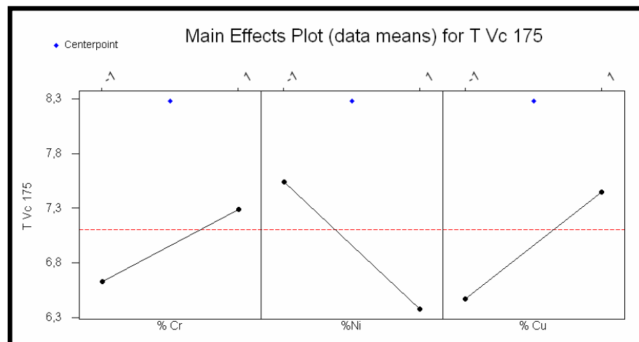
Figura 7.11 - Factorial Plot para os efeitos principais – Vc 175 m/min com fluido de corte.
