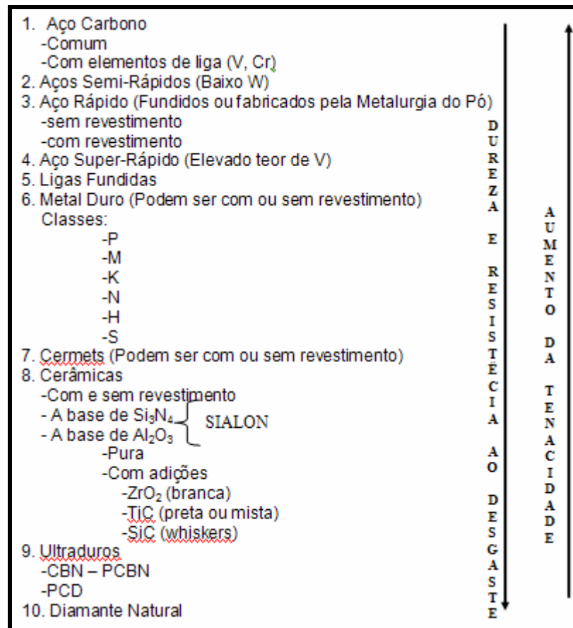
Figura 2.1 - Lista dos materiais para ferramentas de corte (Adaptado de Machado & Silva, 2004).
