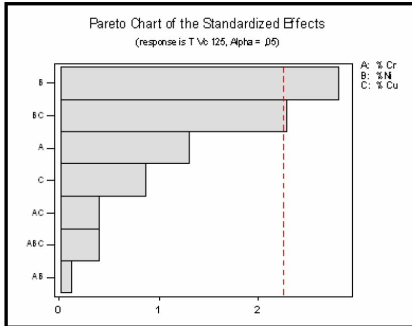
Figura 7.8 – Diagrama de Pareto: efeitos dos elementos e suas interações – Vc 125 m/min.
