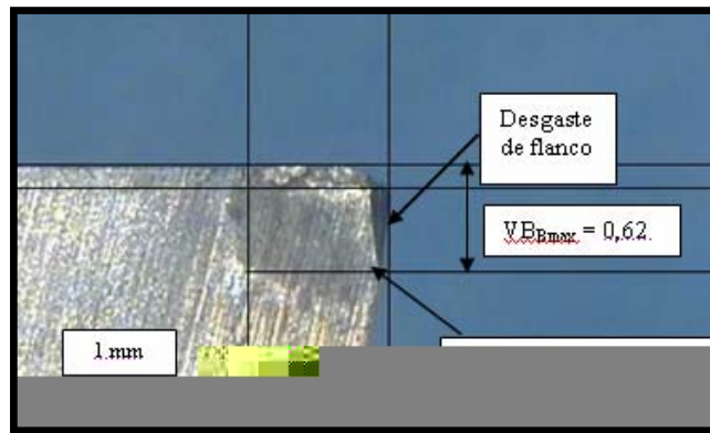
Figura 7.18 – Desgaste de flanco observado na ferramenta de aço-rápido. Aumento 25x, V_c = 150 m/min, a_p = 1 mm, f = 0,1 mm/v.
