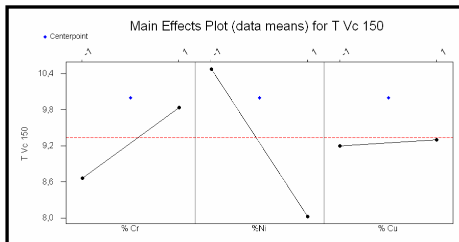
Figura 7.3 - Factorial Plot para os efeitos principais – Vc 150 m/min.
