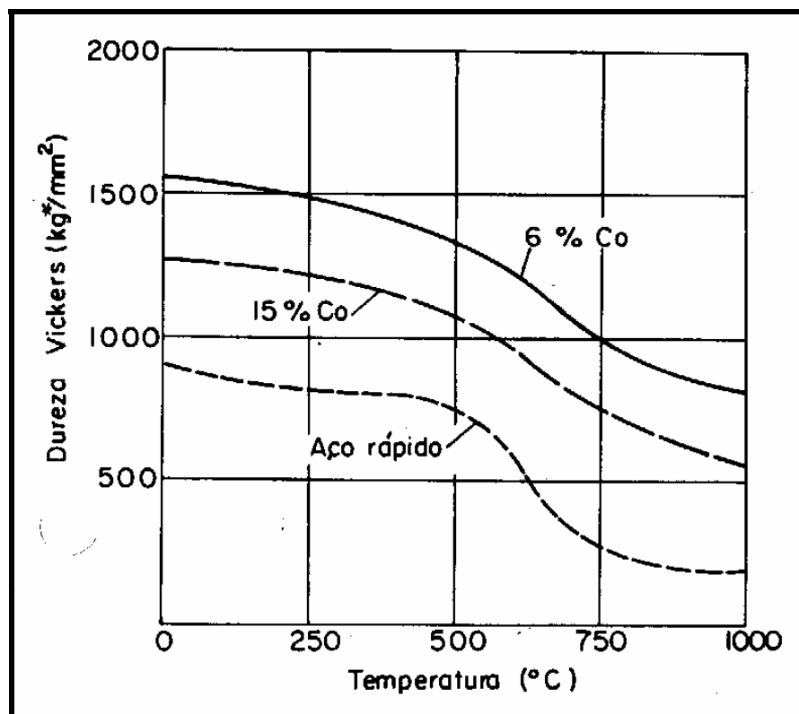
Figura 2.2-Influência da % cobalto e da temperatura na dureza do metal duro (Adaptado Diniz, 2003).
