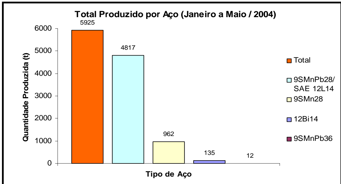
Figura 4.3 - Produção total dos aços-de-corte-fácil da Aços Villares (Prado & Pimentel, 2004).
