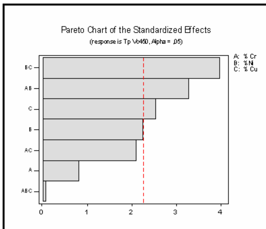
Figura 7.14 – Diagrama de Pareto: efeitos dos elementos e suas interações – Vc 450 m/min.
