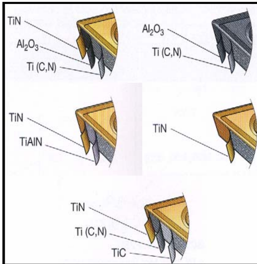
Figura 2.6 – Disposição dos principais revestimentos do metal duro (Adaptada Sandvik, 2005)
