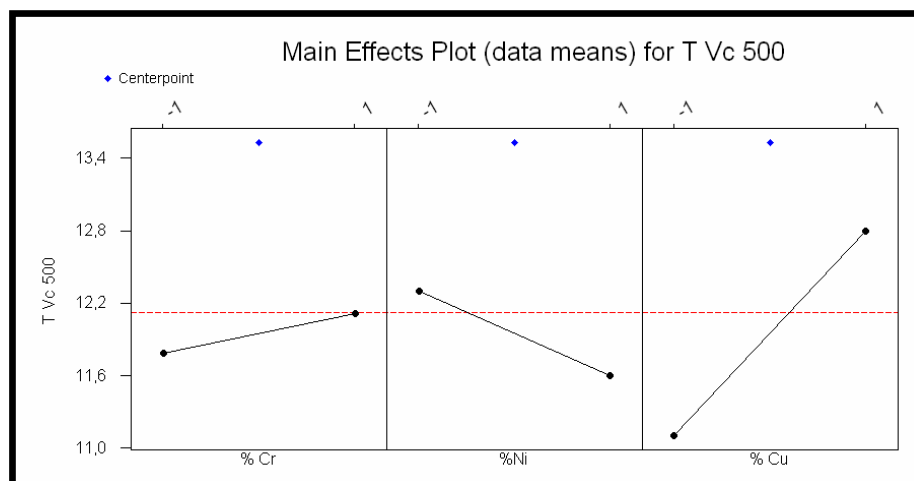
Figura 7.13 - Factorial Plot para os efeitos principais – Vc 500 m/min.
