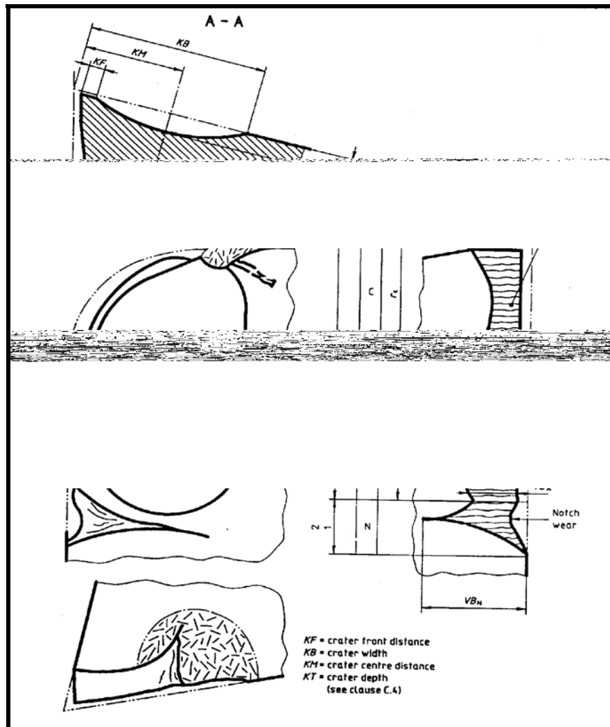
Figura 2.13 – Desgaste da ferramenta (Adaptado Norma ISO 3685, 1993).
