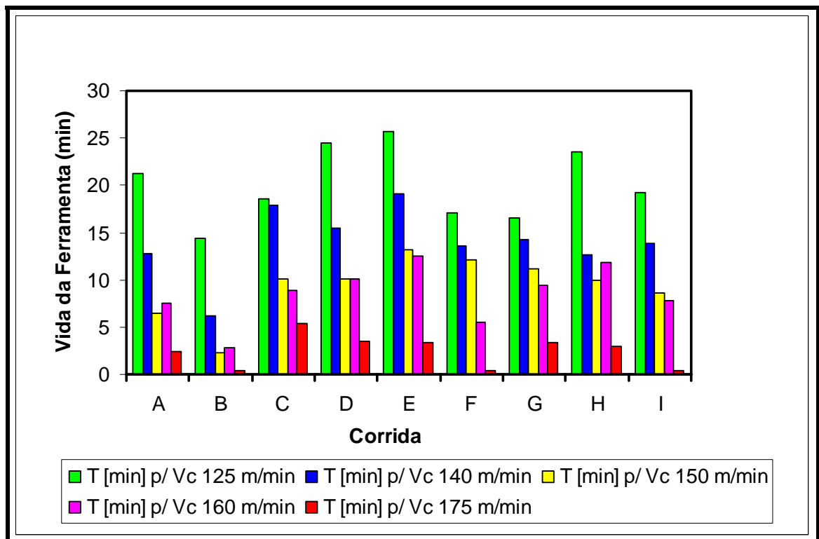
Figura 7.1 – Comparação entre as vidas médias das ferramentas de aço-rápido.
