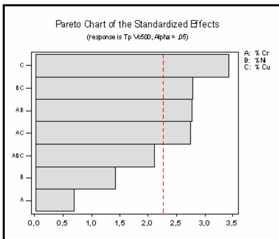
Figura 7.12 – Diagrama de Pareto: efeitos dos elementos e suas interações – Vc 500 m/min.
