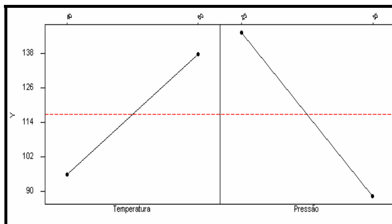
Figura 5.6 – Exemplo do Factorial Plot para os efeitos principais (Adaptada Paiva 2004)
