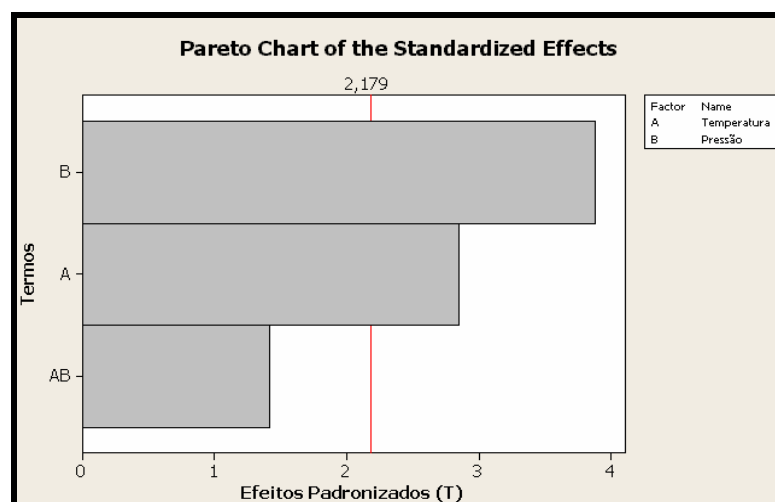
Figura 5.5 – Exemplo do diagrama de Pareto: efeitos dos elementos e suas interações (Adaptada Paiva, 2004)
