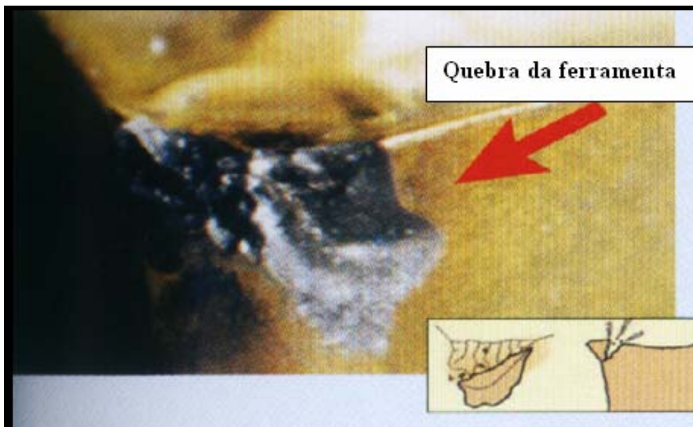
Figura 2.11 – Quebra da ferramenta (Adaptada Sandvik, 2005).
