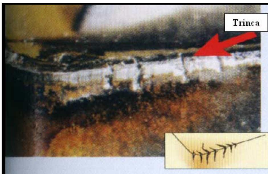
Figura 2.8 – Trincas ou fissuras térmicas na aresta de corte (Adaptada Sandvik, 2005).
