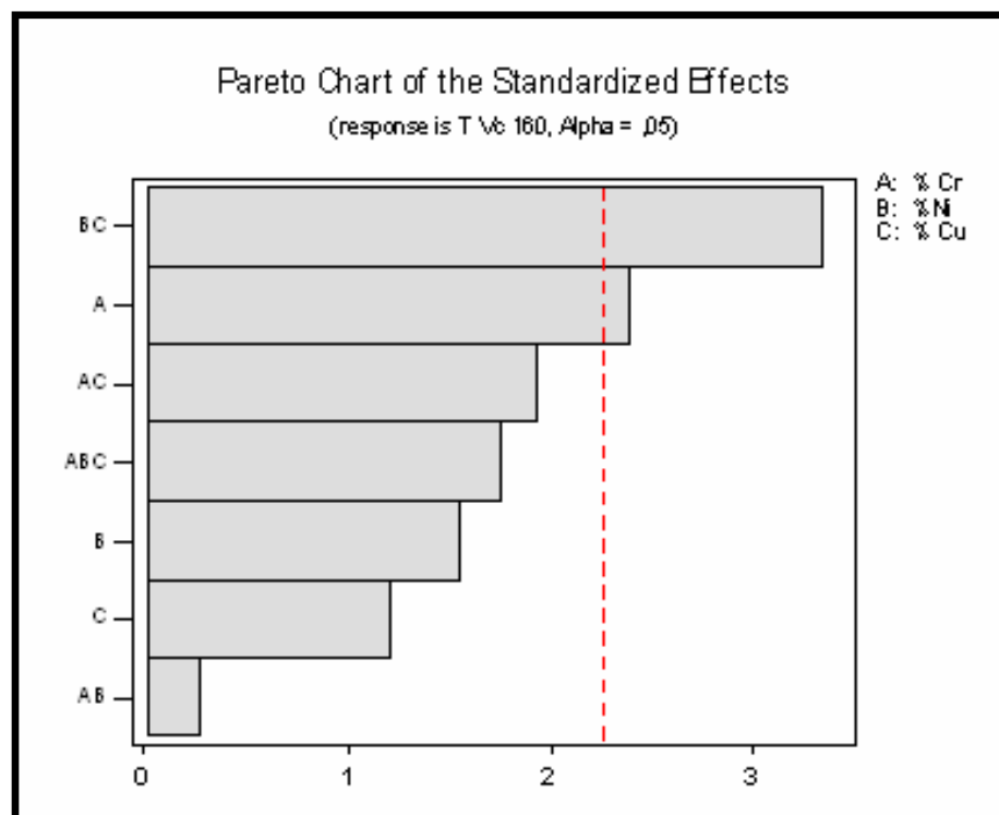
Figura 7.4 – Diagrama de Pareto: efeitos dos elementos e suas interações – Vc 160 m/min.
