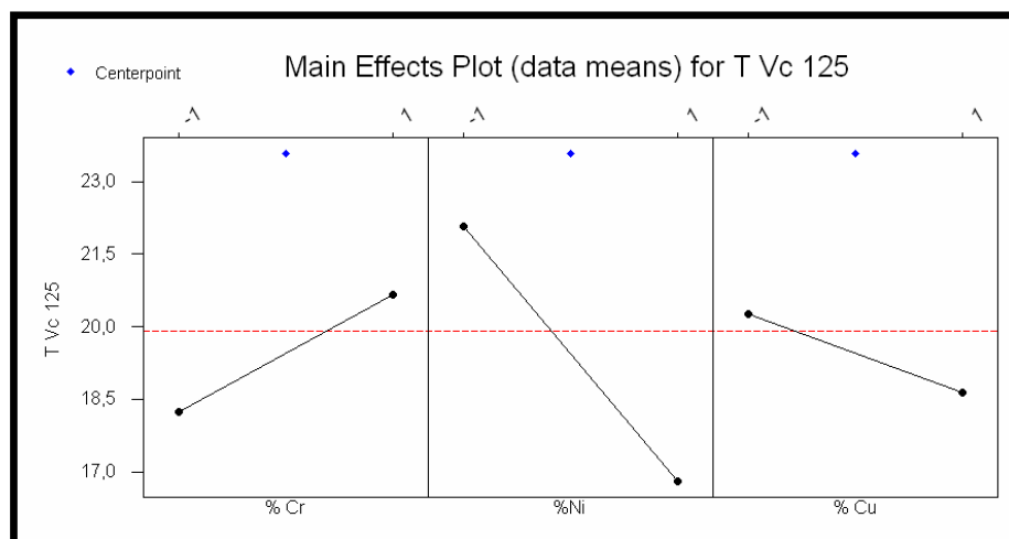
Figura 7.9 - Factorial Plot para os efeitos principais – Vc 125 m/min.
